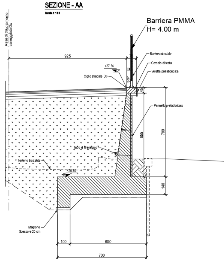
Fig. 1 - Sezione quotata del muro
