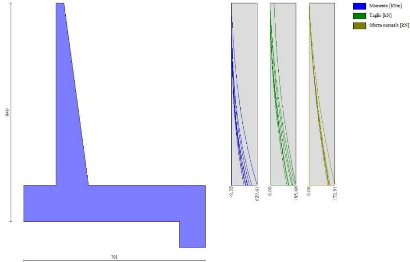
Fig. 8 - Paramento
