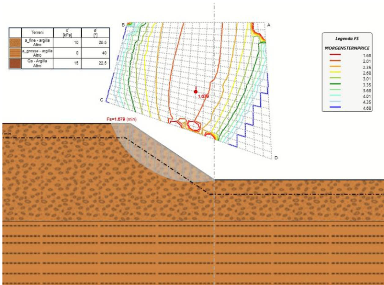
Figura 5: Verifica di stabilità globale in condizioni statiche.
