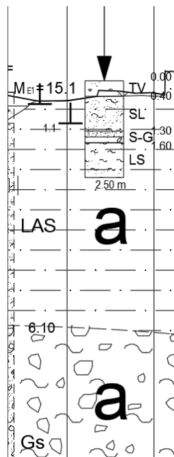
Figura 4: Sezioni geotecniche per l'opera in esame
