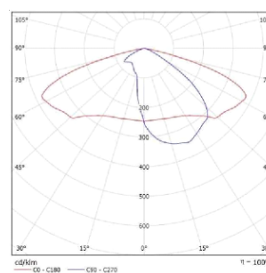
CURVA FOTOMETRICA
