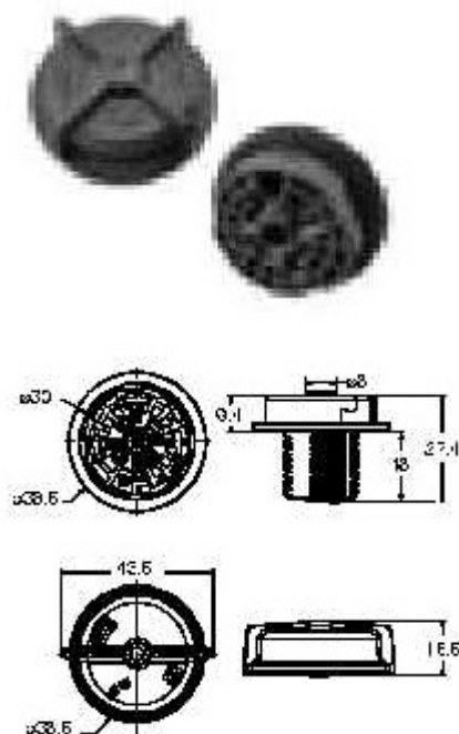
Dispositivo punto-punto
