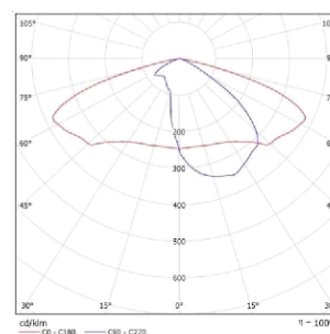
CURVA FOTOMETRICA
