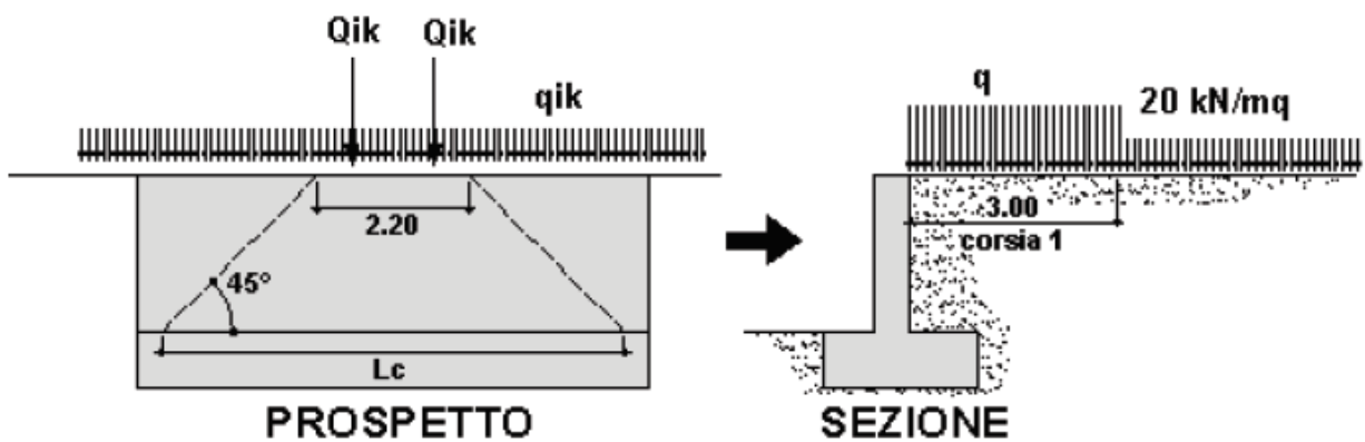
5-Schema di diffusione dei carichi mobili
