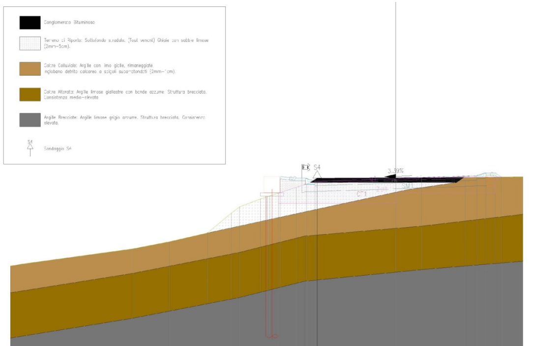
4 - Sezione geologica
