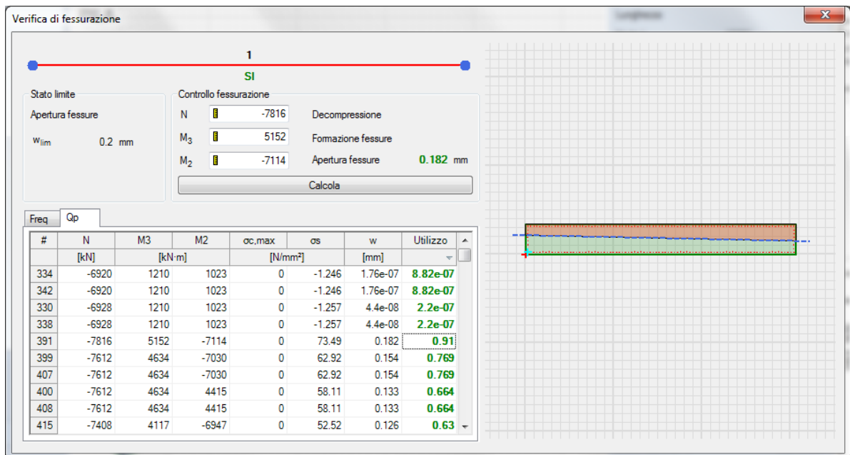
Figura 12-9 – Dettaglio verifica fessurazione comb. q.perm. (unità di misura: kN; m; °C)
