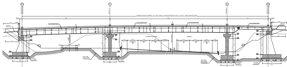
Figura 1-1: Prospetto longitudinale
