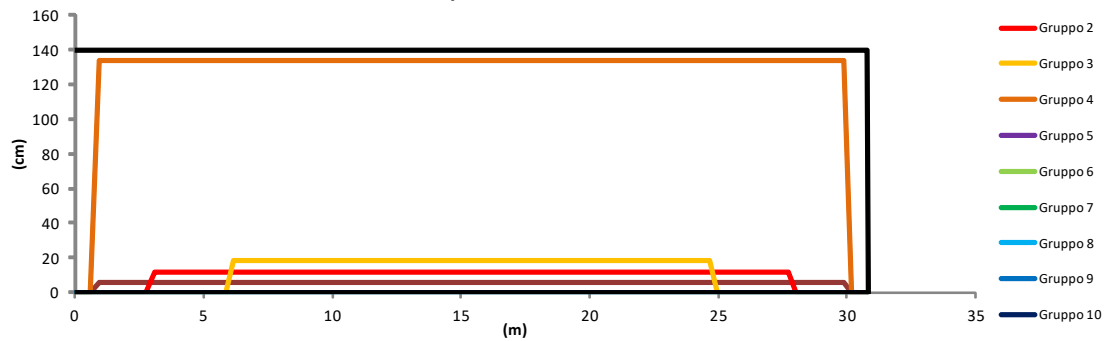
Disposizione Trefoli 6/10S
