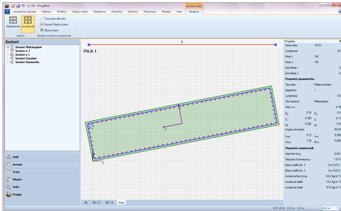
Figura 10-1 – Pila 1: sezione di verifica 4.78 x 1.00 – \phi 26/10
