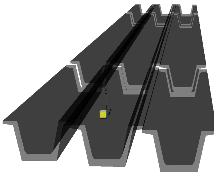
Figura 5-1: Modello di calcolo: dettaglio travi
