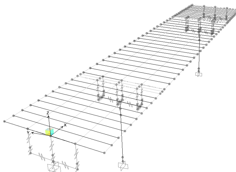
Figura 5-3: Modello di calcolo: con elementi shell soletta non in vista
