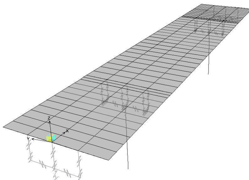
Figura 5-2: Modello di calcolo: con elementi shell soletta in vista
