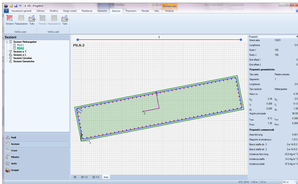
Figura 11-1 – Pila 2: sezione di verifica 4.78 x 1.00 – \phi 26/10
