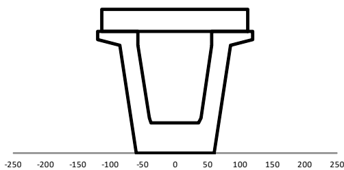
SEZIONE TIPO B
