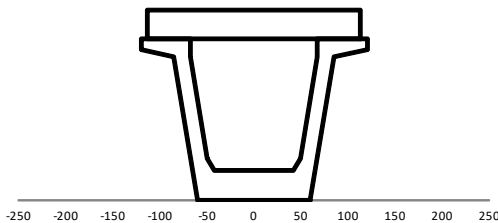
SEZIONE TIPO A
