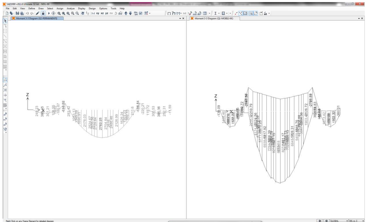
Figura 7-5: Momento flettente M33 – trave 1 – sollecitazioni elementari
