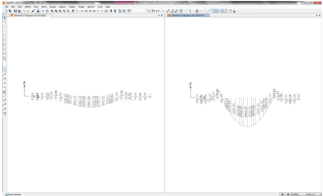
Figura 7-4: Momento flettente M33 – trave 1 – sollecitazioni elementari
