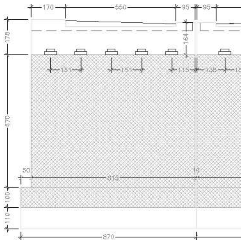
F 3. Rampe laterali – Prospetto spalle
