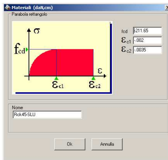
F 16. Calcestruzzo soletta C35/45 – Legame costitutivo
