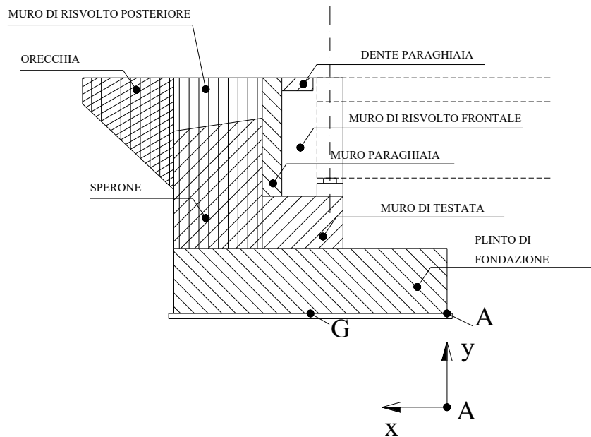
F 13. Schema longitudinale spalla – Elementi strutturali
