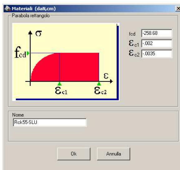
F 15. Calcestruzzo trave c.a.p. C45/55 – Legame costitutivo
