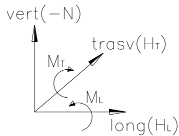
F 14. Convenzione per le sollecitazioni
