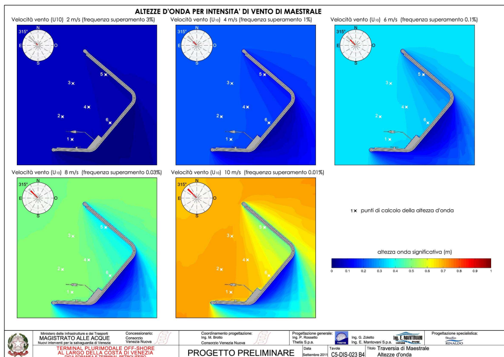
Figura 44: traversia di Maestrale - altezze d'onda per diverse intensità del vento
