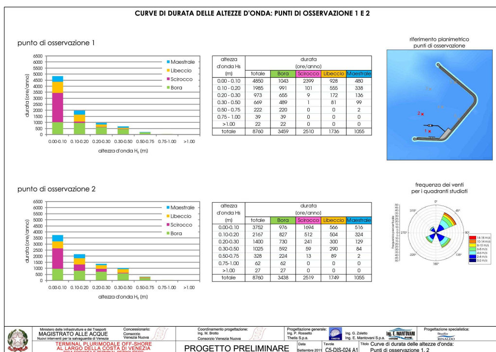
Figura 45: curve di durata delle altezze d'onda – punti di osservazione 1 e 2
