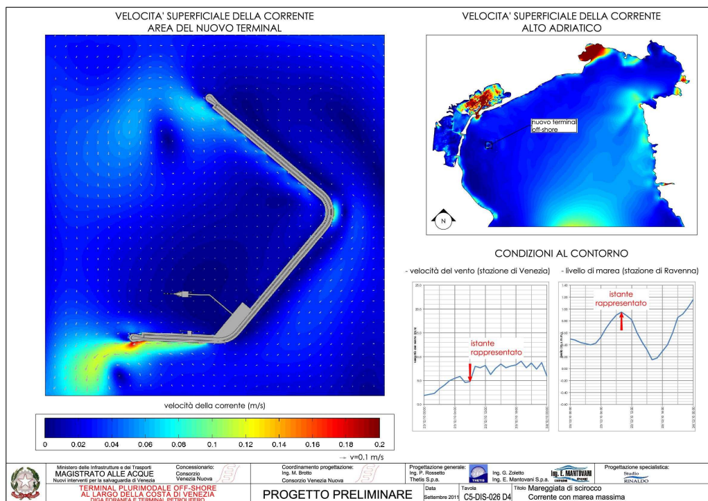
Figura 69: velocità della corrente con mareggiata di scirocco – marea massima
