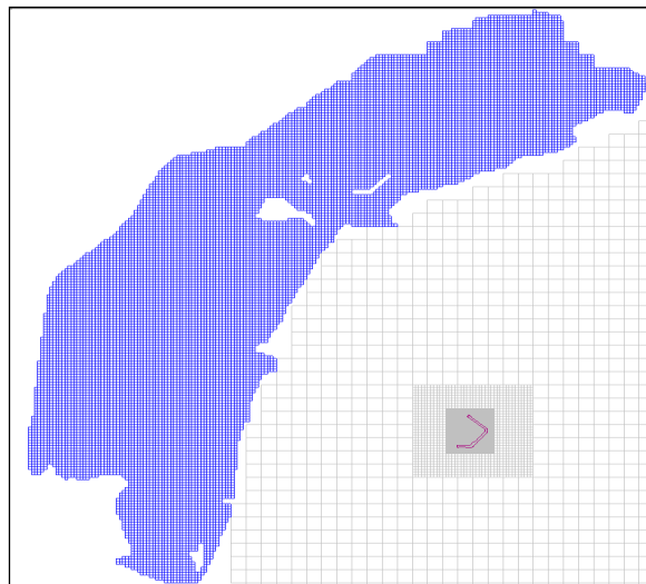
Figura 5: griglia n.3 – Laguna di Venezia
