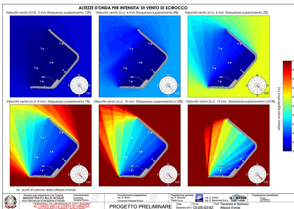
Figura 42: traversia di Scirocco - altezze d'onda per diverse intensità del vento
