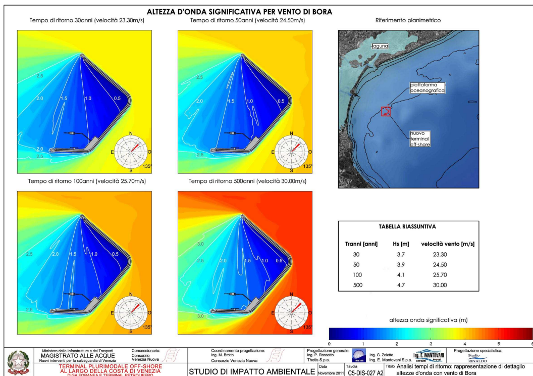
Figura 31: altezze d'onda significative in relazione al tempo di ritorno con vento di bora – area portuale
