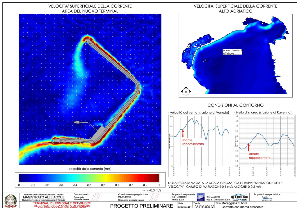
Figura 63: velocità della corrente con mareggiata di bora – marea crescente
