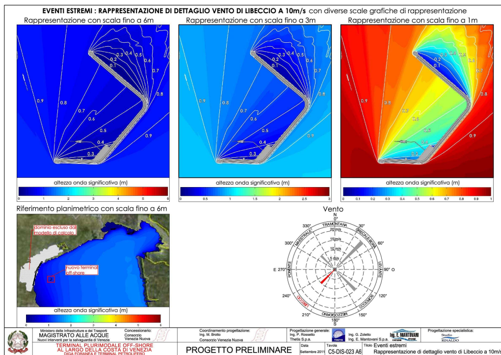
Figura 39: vento di Libeccio a 10 m/s - rappresentazione di dettaglio delle altezze d'onda
