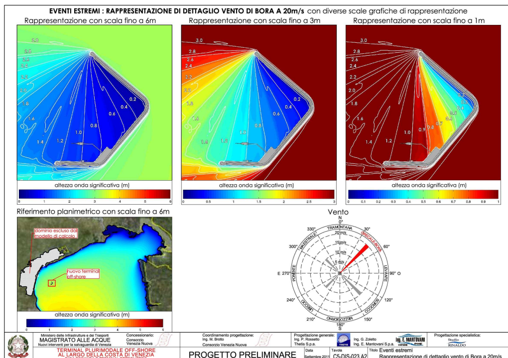
Figura 36: vento di Bora a 20 m/s - rappresentazione di dettaglio delle altezze d'onda
