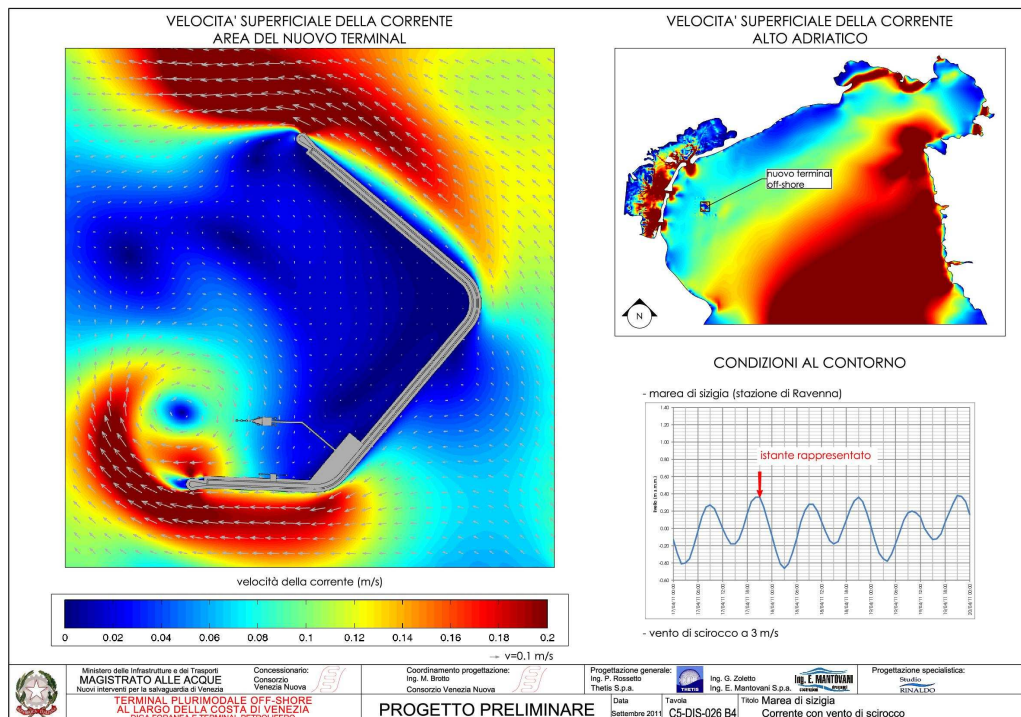
Figura 57: velocità della corrente con vento di scirocco – marea di sizigia
