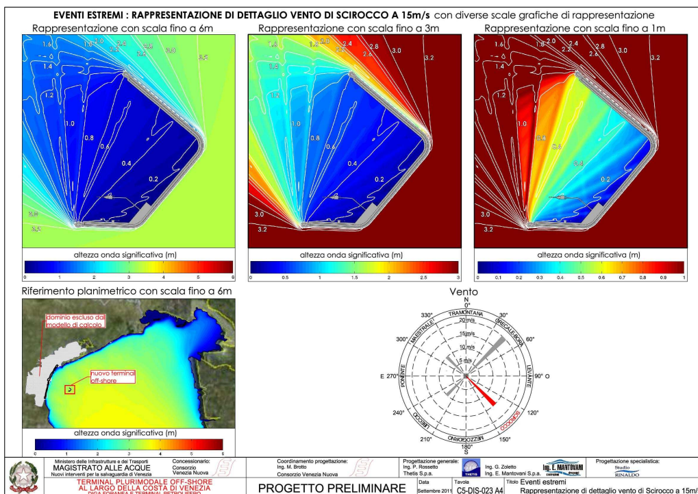
Figura 38: vento di Scirocco a 15 m/s - rappresentazione di dettaglio delle altezze d'onda
