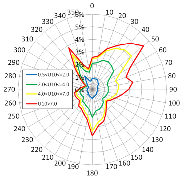
Figura 11: rosa di distribuzione media annuale del vento in corrispondenza alla diga Sud di Lido.
