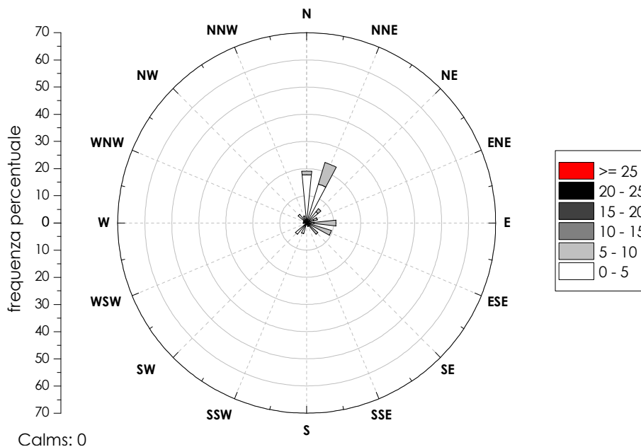
Figura 65: frequenza dei venti registrati dalla stazione mareografica di Venezia 22/12/2010 - 25/12/2010
