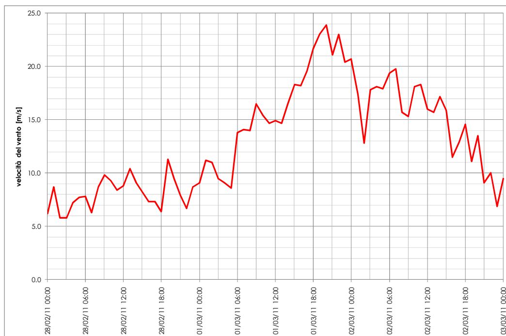
Figura 60: velocità del vento per la stazione mareografica di Ravenna 28/02/2011 - 03/03/2011
