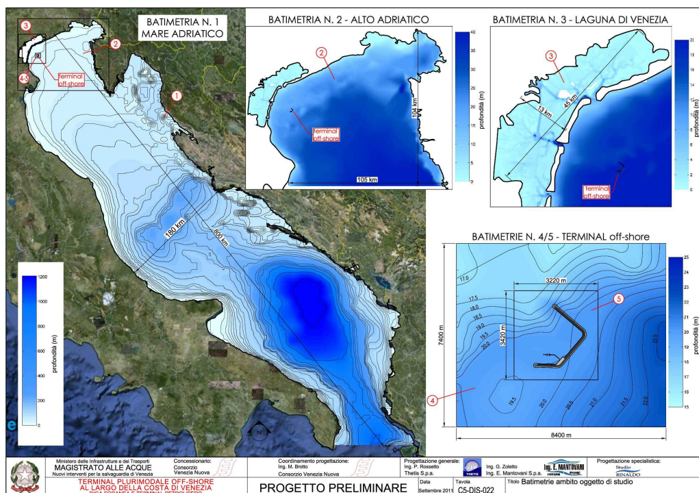
Figura 8: carte batimetriche
