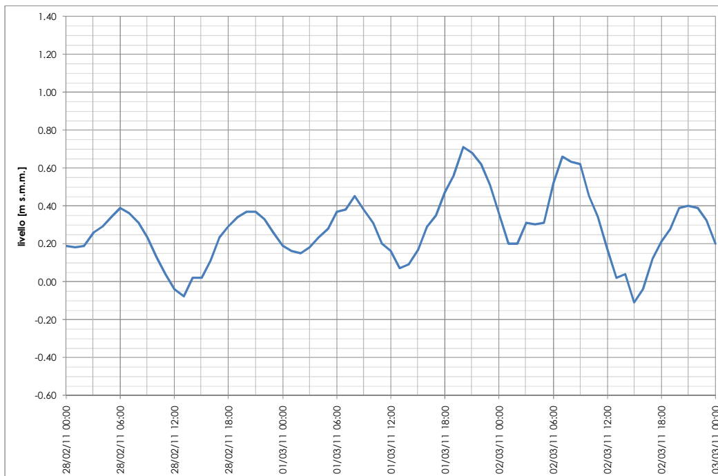
Figura 61: livelli di marea per la stazione mareografica di Ravenna 28/02/2011 - 03/03/2011
