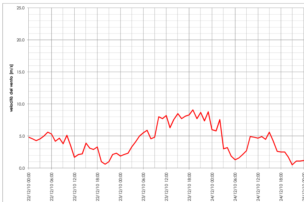
Figura 66: velocità del vento per la stazione mareografica di Ravenna 22/12/2010 - 25/12/2010
