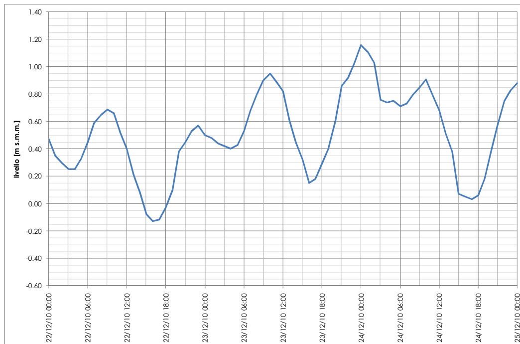
Figura 67: livelli di marea per la stazione mareografica di Ravenna 22/12/2010 - 25/12/2010
