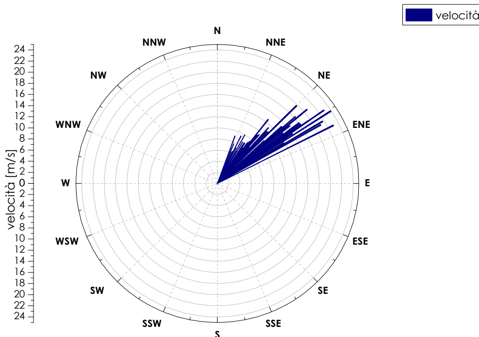
Figura 58: intensità e direzione dei venti registrati dalla stazione mareografica di Venezia 28/02/2011 - 03/03/2011
