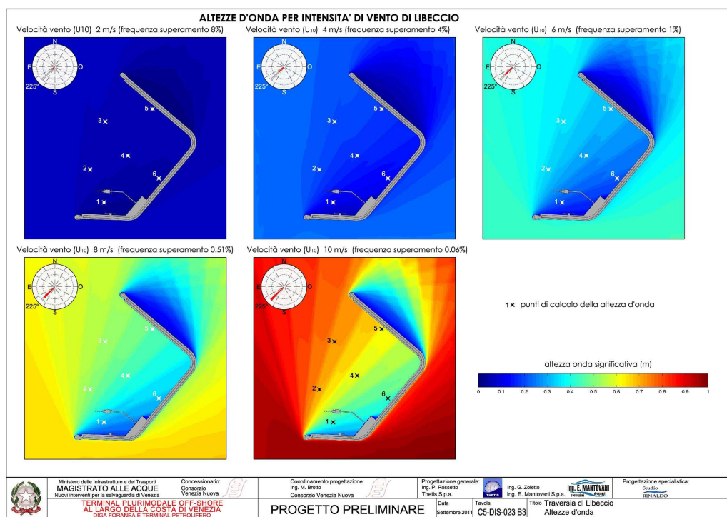
Figura 43: traversia di Libeccio - altezze d'onda per diverse intensità del vento
