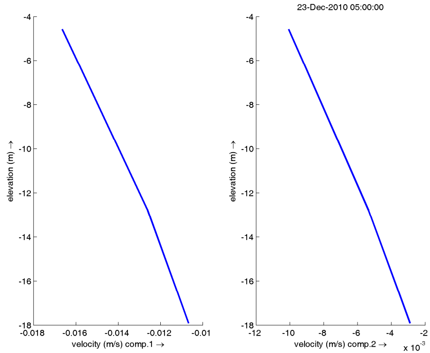
Figura 50: andamento delle componenti x e y della velocità lungo la verticale nel punto 1
