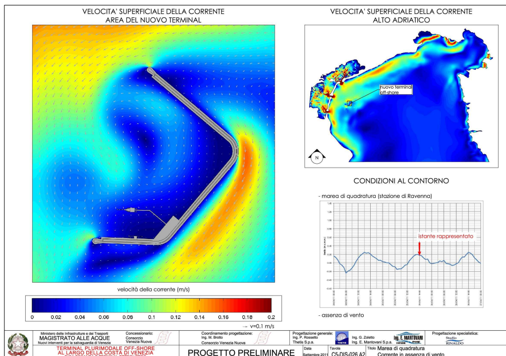
Figura 53: velocità della corrente in assenza di vento – marea di quadratura
