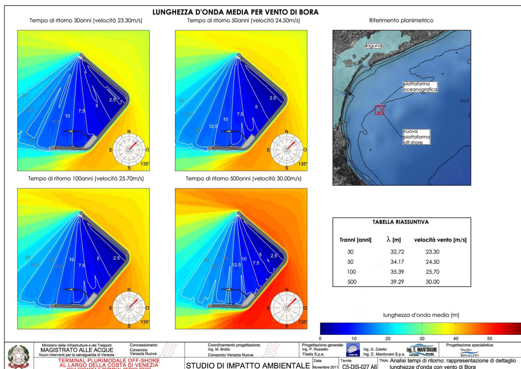
Figura 33: lunghezze d'onda in relazione al tempo di ritorno con vento di bora – area portuale
