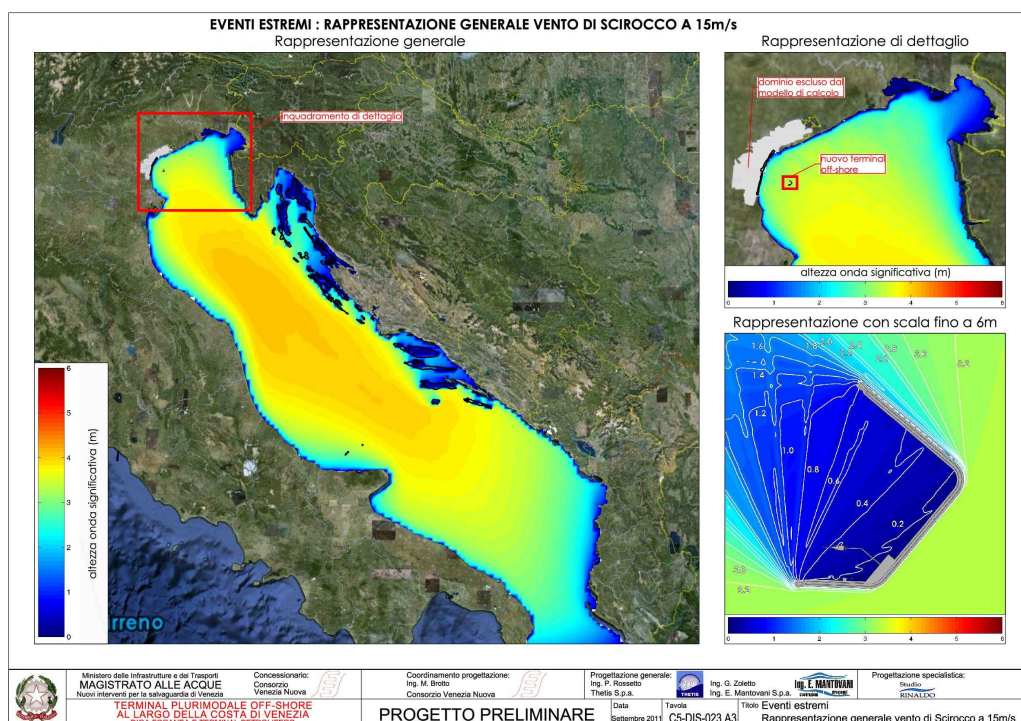
Figura 37: vento di Scirocco a 15 m/s - rappresentazione generale delle altezze d'onda
