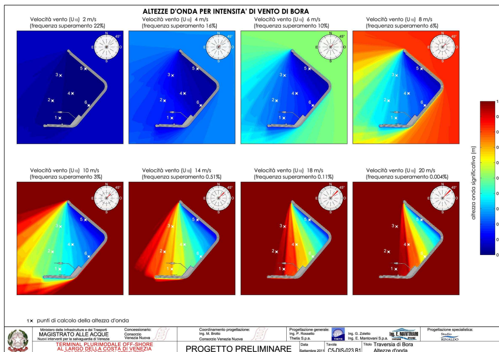
Figura 41: traversia di Bora - altezze d'onda per diverse intensità del vento
