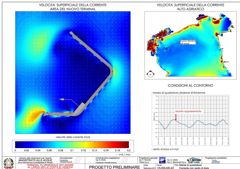
Figura 54: velocità della corrente con vento di bora – marea di quadratura
