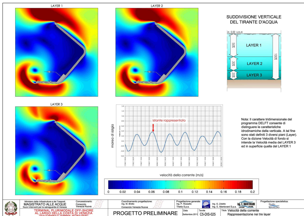
Figura 46: velocità nei tre layer
