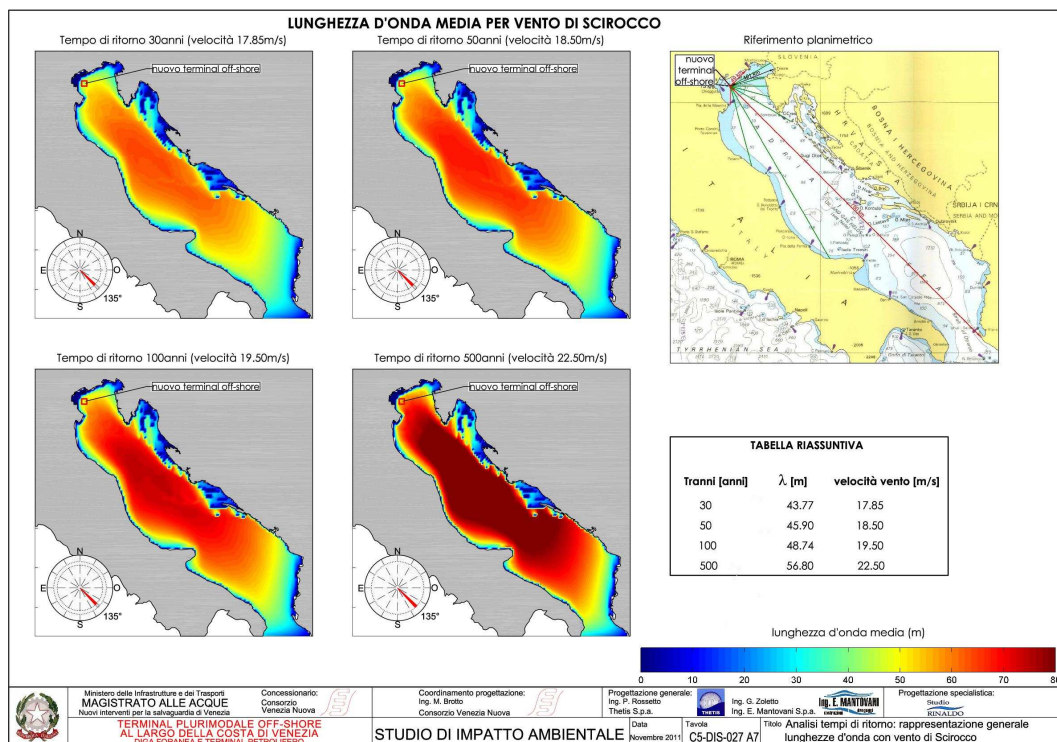
Figura 34: lunghezze d'onda in relazione al tempo di ritorno con vento di scirocco – mare Adriatico
