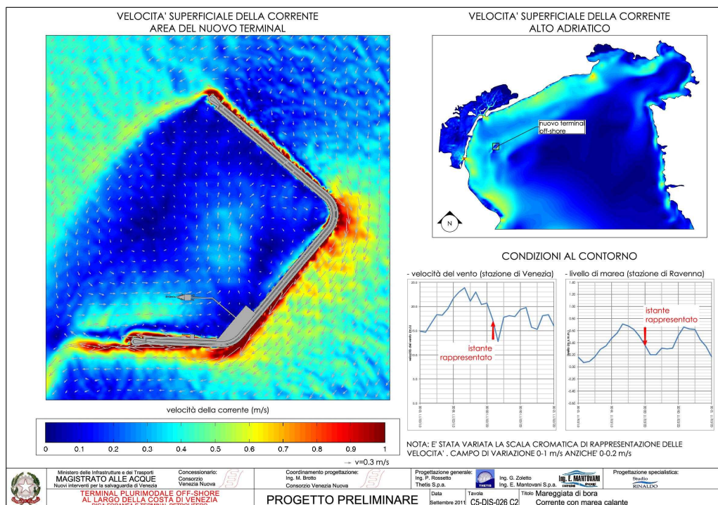
Figura 62: velocità della corrente con mareggiata di bora – marea calante
