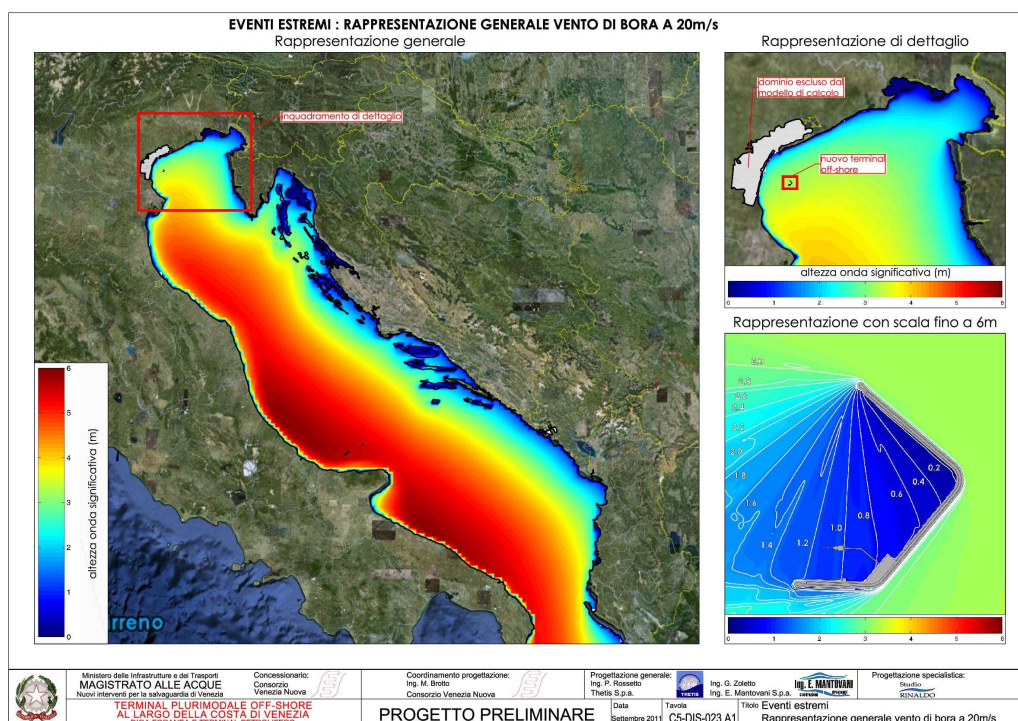
Figura 35: vento di Bora a 20 m/s - rappresentazione generale delle altezze d'onda
