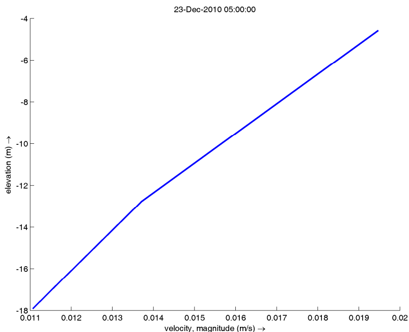
Figura 49: andamento della velocità lungo la verticale nel punto 1
