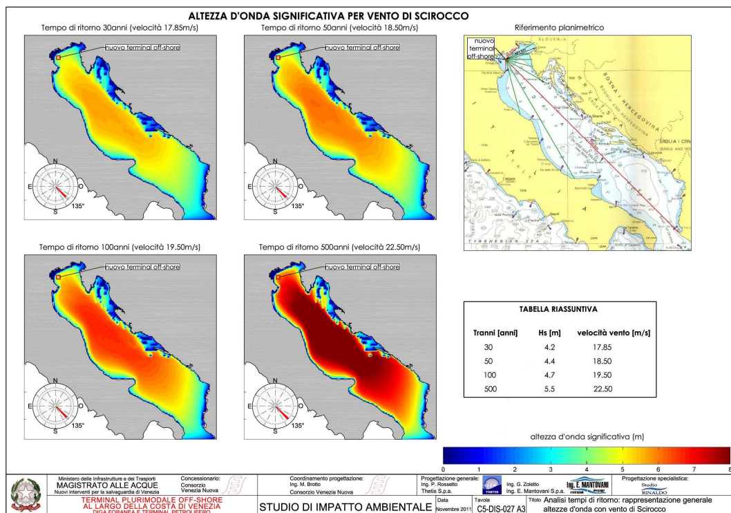
Figura 32: altezze d'onda significative in relazione al tempo di ritorno con vento di scirocco – mare Adriatico
