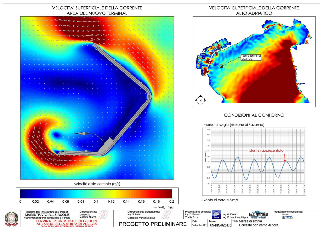
Figura 56: velocità della corrente con vento di bora – marea di sizigia
