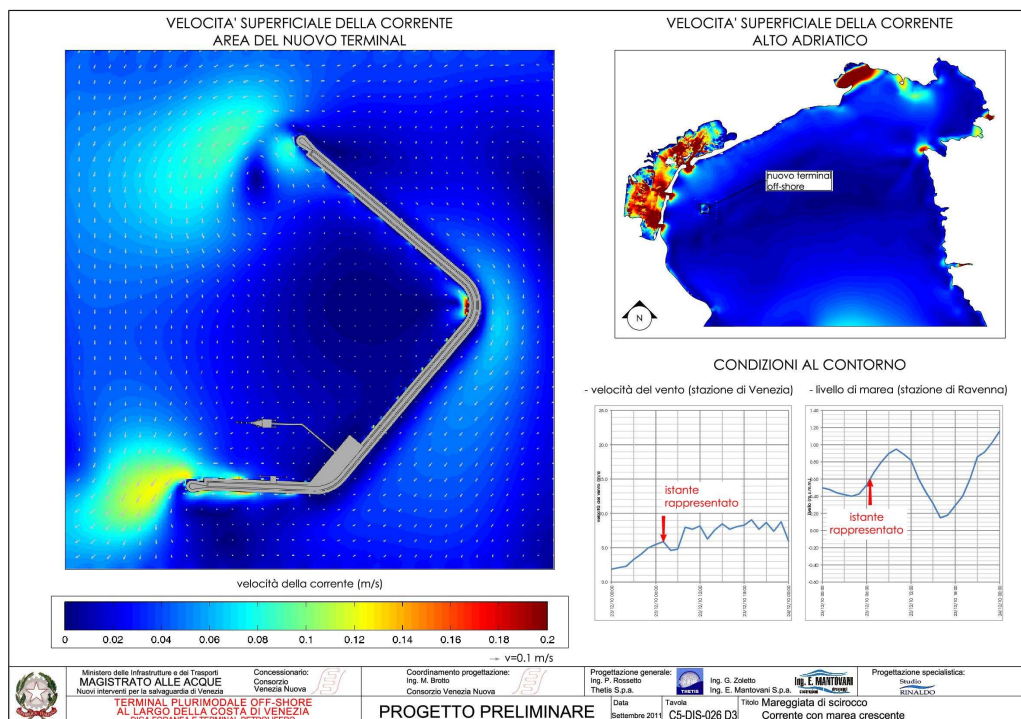
Figura 68: velocità della corrente con mareggiata di scirocco – marea crescente
