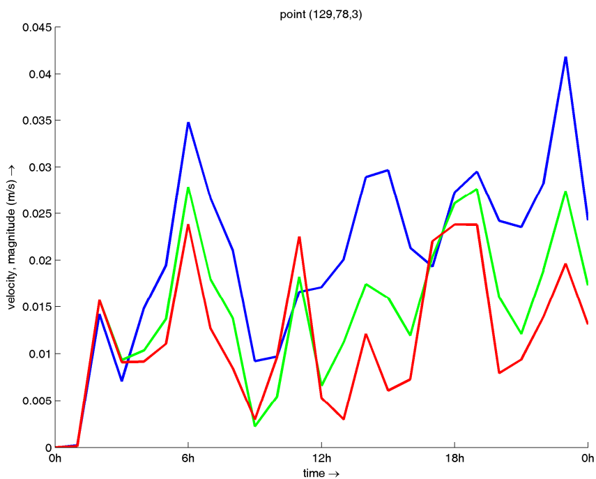
Figura 48: andamento temporale della velocità nel punto 1 per i 3 layer
