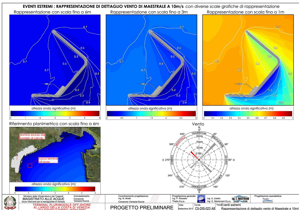
Figura 40: vento di Maestrale a 10 m/s - rappresentazione di dettaglio delle altezze d'onda
