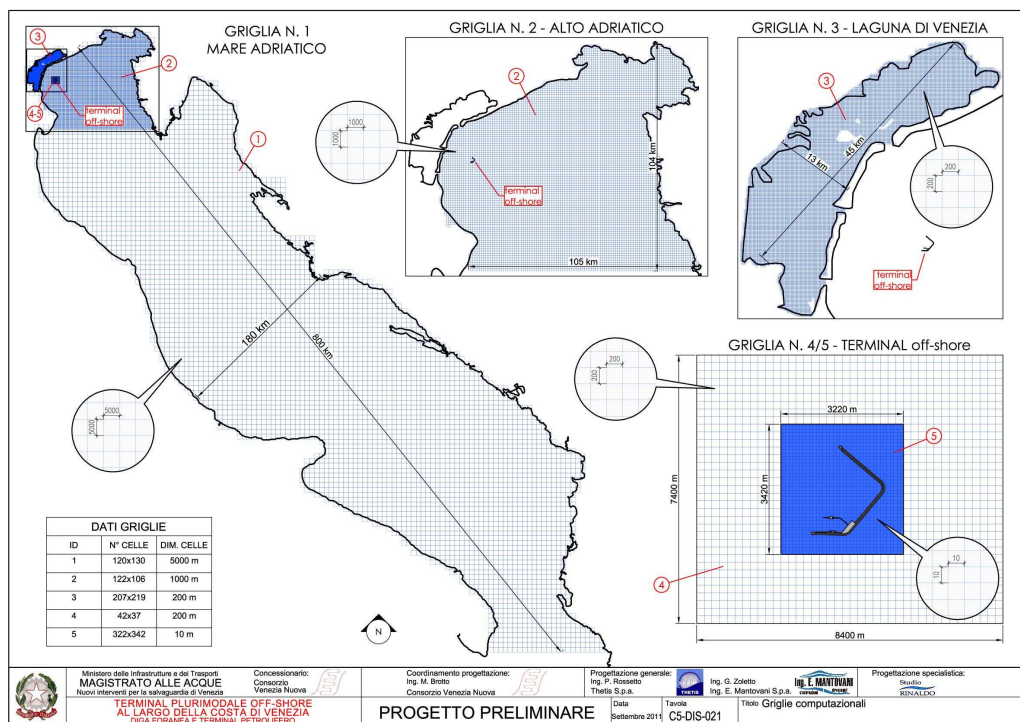
Figura 7: griglie computazionali
