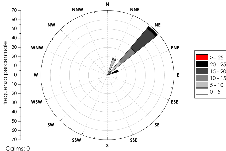
Figura 59: frequenza dei venti registrati dalla stazione mareografica di Venezia 28/02/2011 - 03/03/2011
