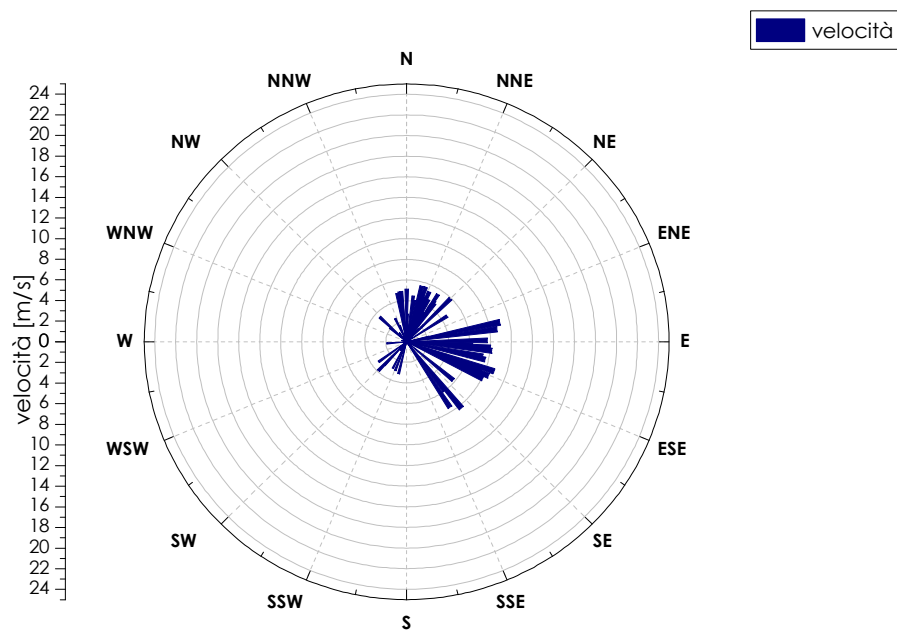
Figura 64: intensità e direzione dei venti registrati dalla stazione mareografica di Venezia 22/12/2010 - 25/12/2010
