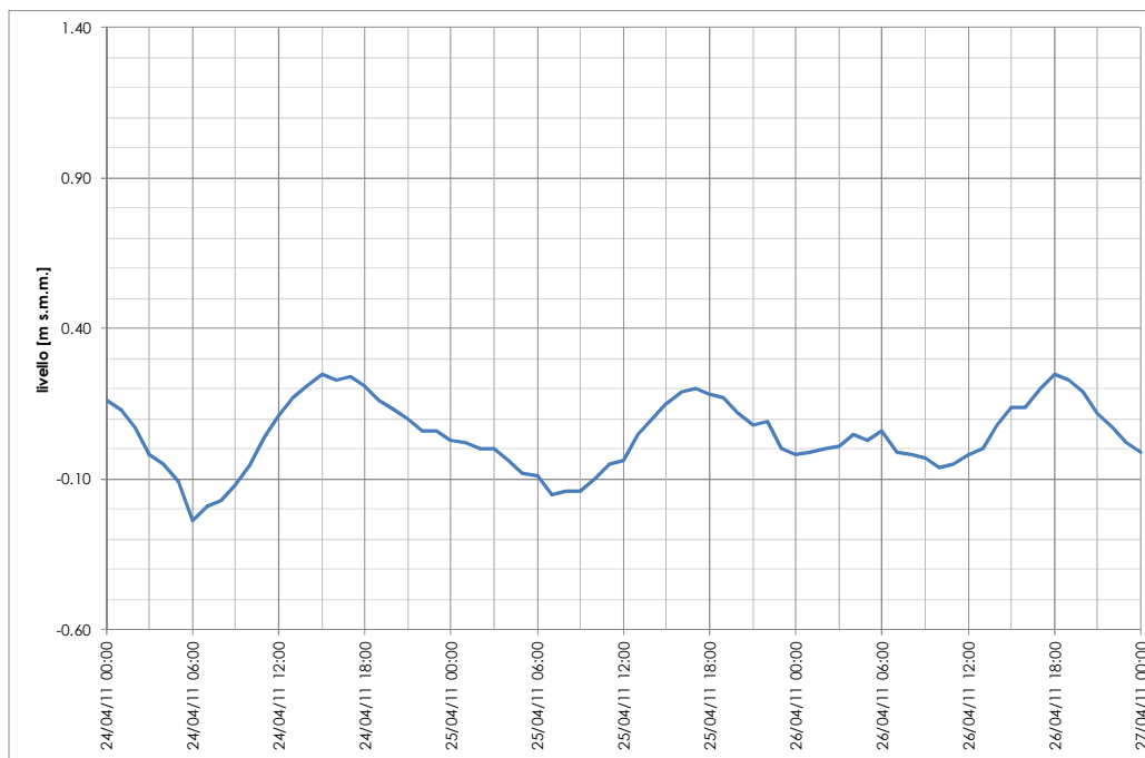
Figura 52: livelli di marea per la stazione mareografica di Ravenna nel periodo 24/04/2011 - 27/04/2011
