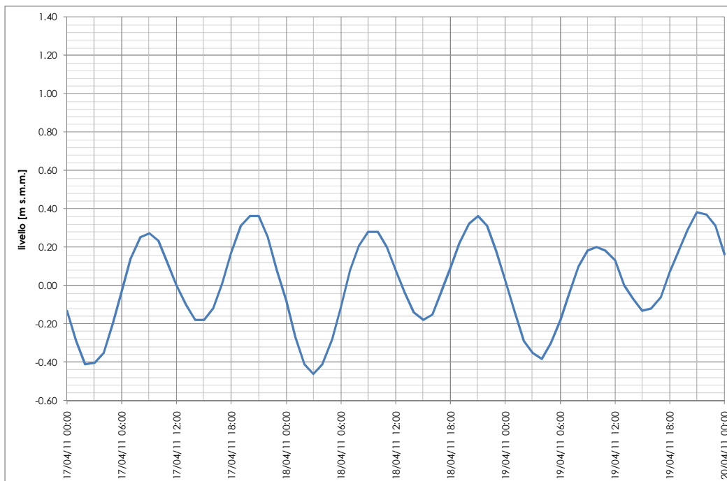
Figura 55: livelli di marea per la stazione mareografica di Ravenna nel periodo 17/04/2011 - 20/04/2011
