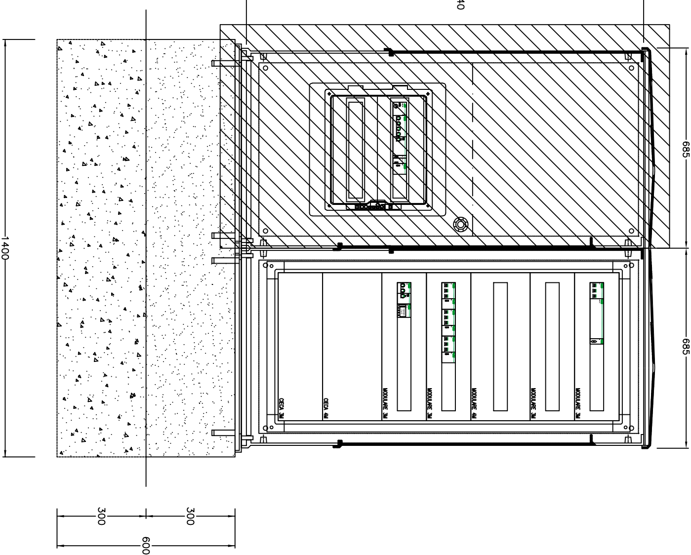
Quadro elettrico svincolo Petrosino (Q3)
