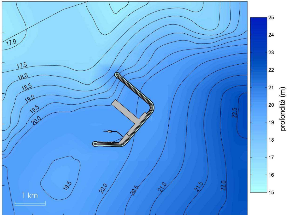
Figura 2-4 Batimetrie dell'area del nuovo Terminal Off-shore.
