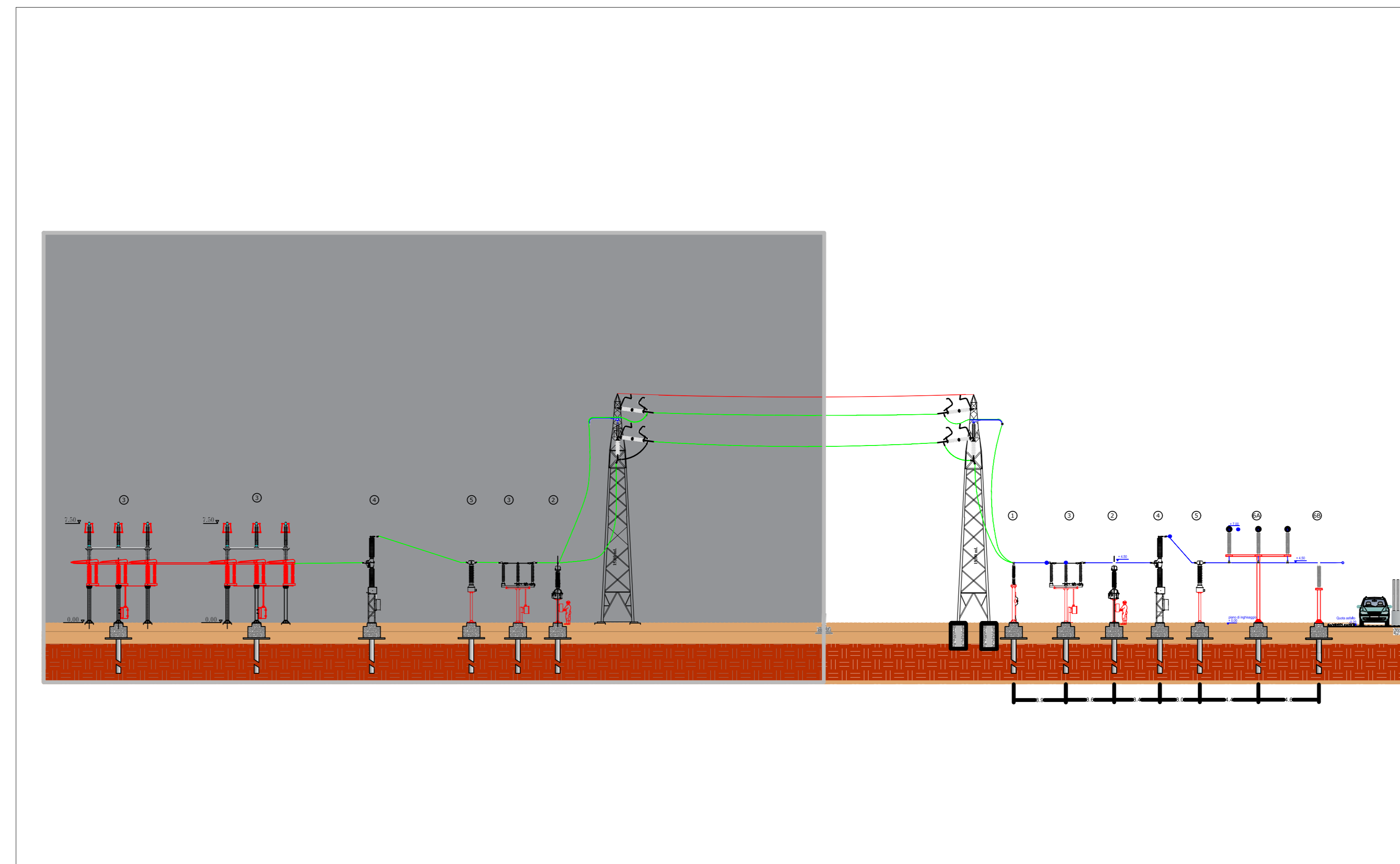
Profilo elettromeccanico LONGITUDINALE STALLO COMUNE AI PRODUTTORI
