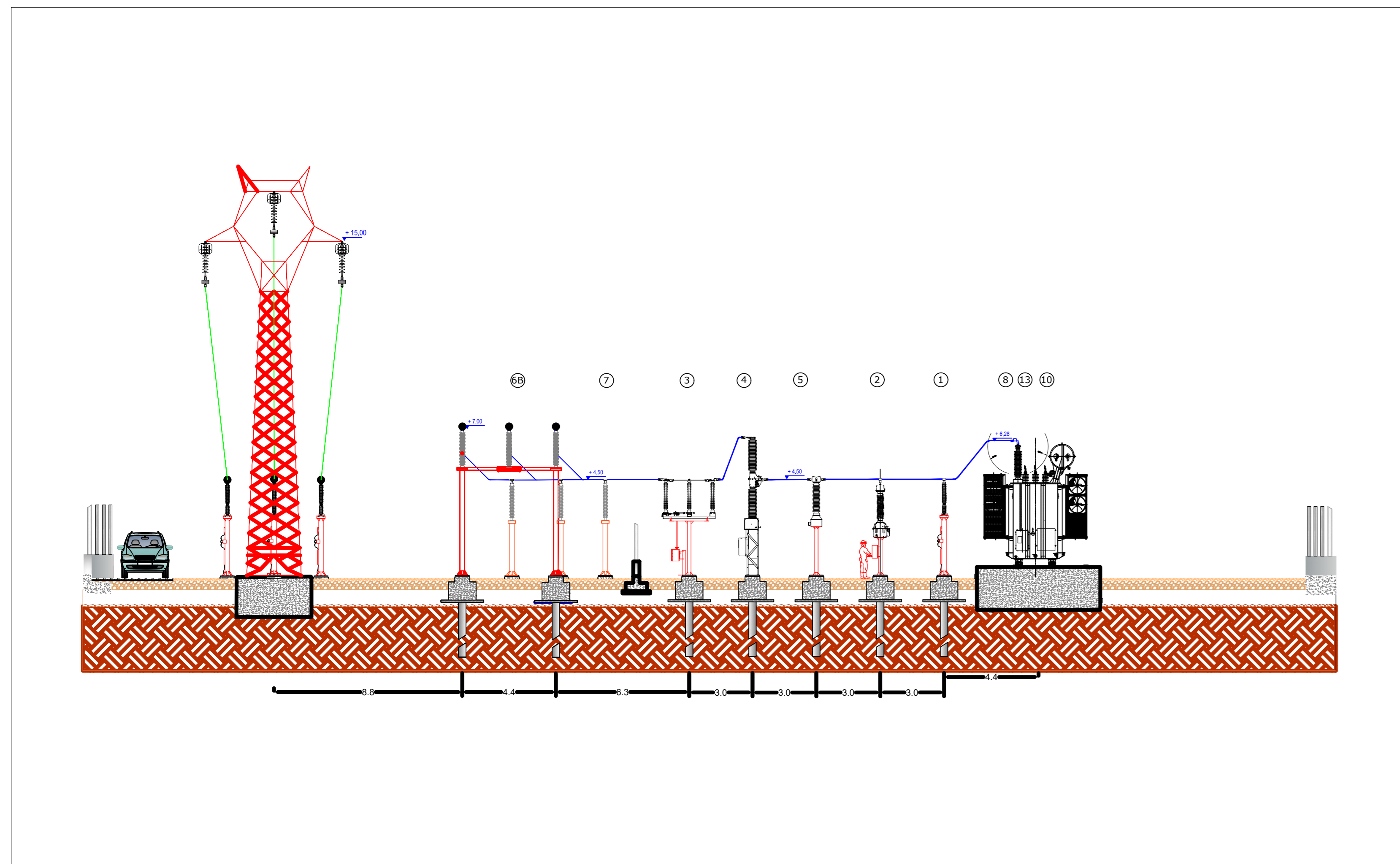
Profilo elettromeccanico LONGITUDINALE
