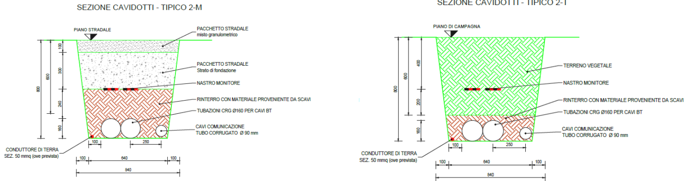
Figura 29 - Particolare sezione tipo cavo interrato BT
