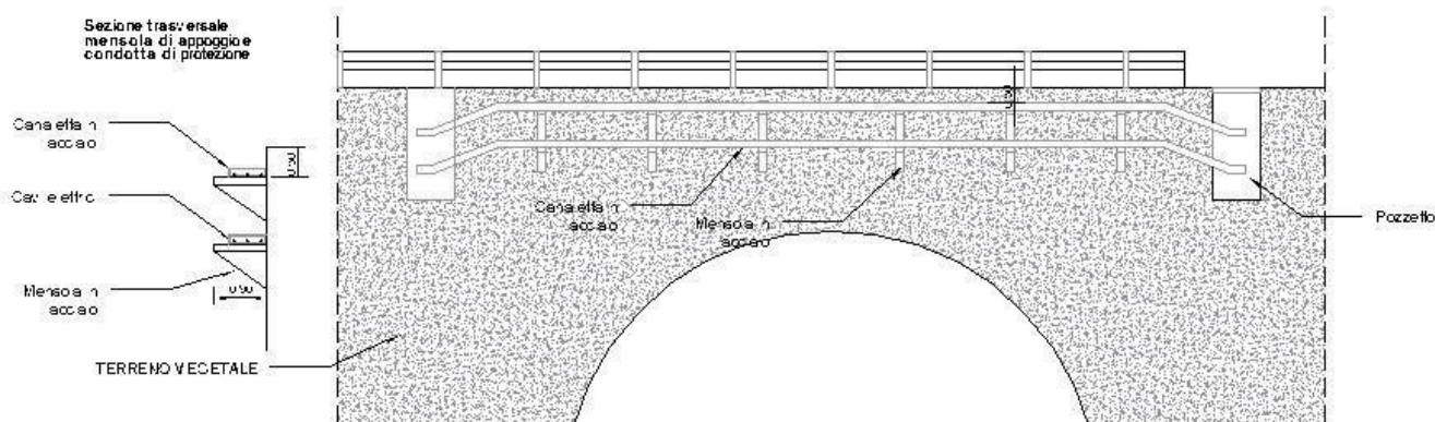
Figura 33 - Particolare attraversamento trasversale in prossimità di interferenza con condotta in cemento o in acciaio e di interferenza con ponte stradale.
