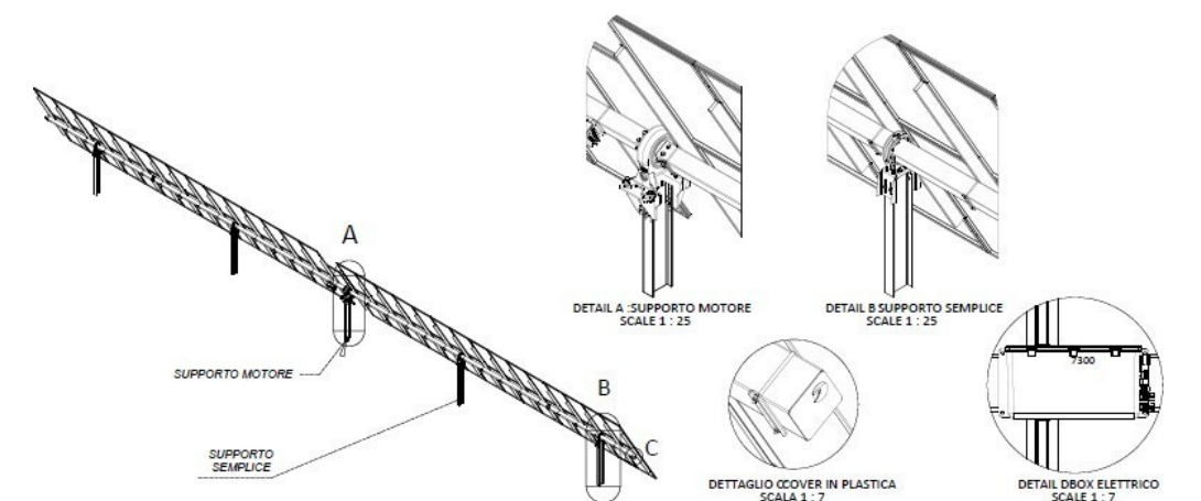
Figura 25 - Particolari costruttivi degli inseguitori installati
