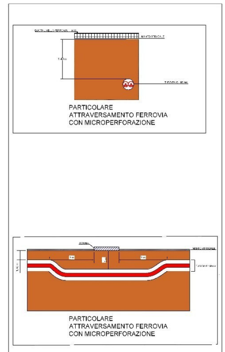
Figura 35 - Particolare attraversamento trasversale in prossimità di interferenza con ferrovia.
