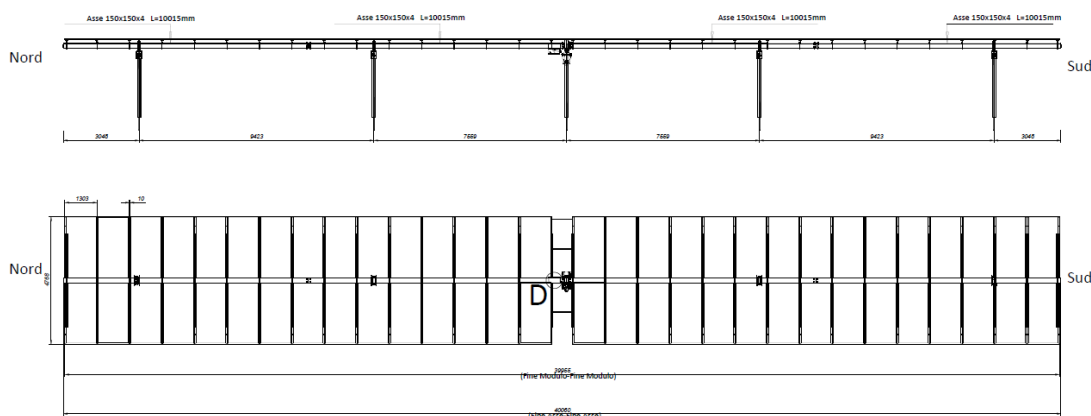
Figura 26 - Particolare vista in sezione e in planimetria delle strutture
