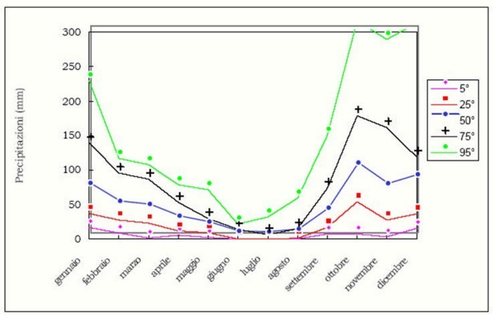
Figura 16 - Andamento delle precipitazioni nella stazione di Catania (4 m s.l.m.)
