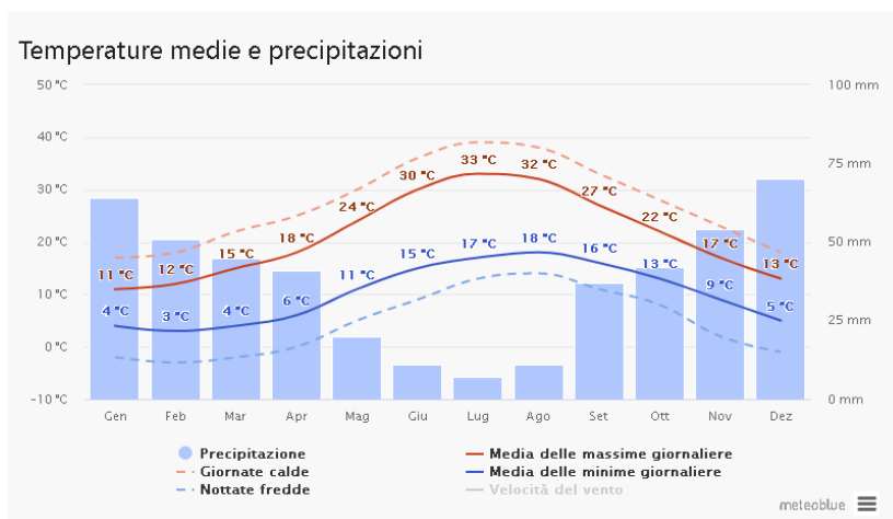
Figura 42 - Temperature medie e precipitazioni
