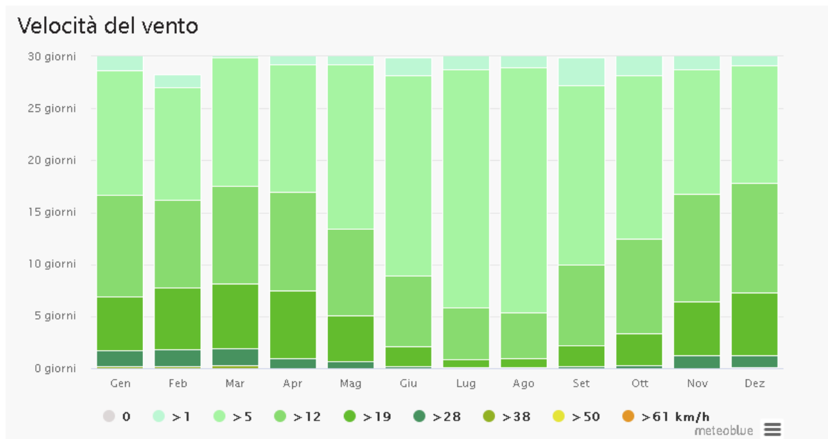
Figura 46 - Velocità del vento.
