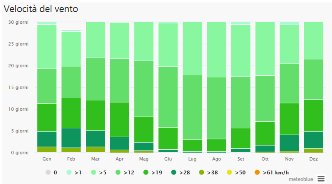
Figura 41 - Velocità del vento.
