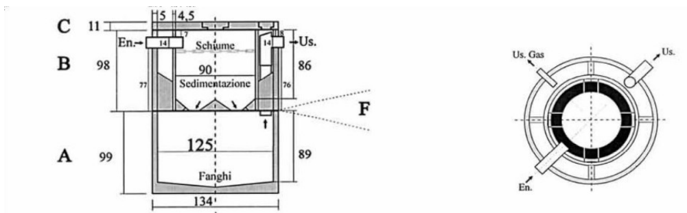
Figura 27 - Fossa IMHOFF
