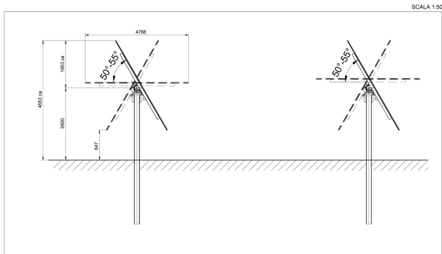
Figura 20 - Profilo longitudinale struttura
