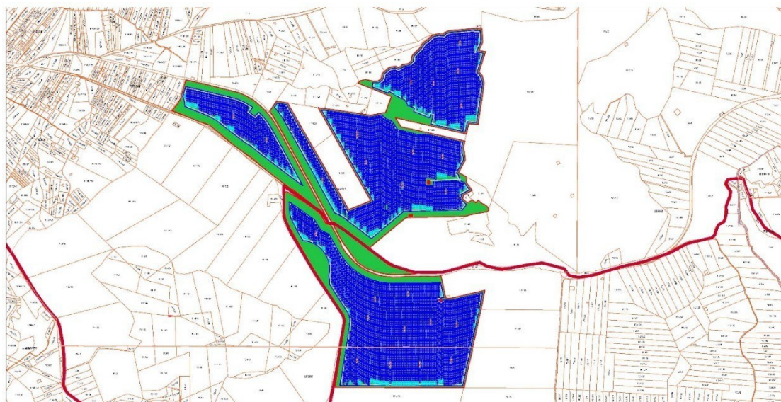
Figura 17 - Layout dell'area d'impianto FV_Ramione ricadente nel territorio di Caltagirone (CT) su base catastale.
