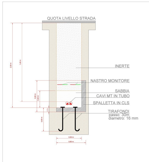
Figura 30 - Particolare sezione tipo cavo interrato MT su strada
