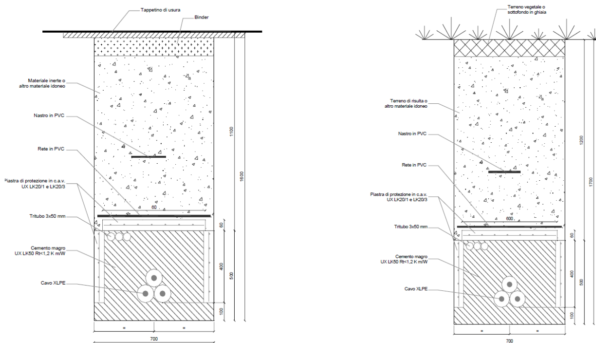
Figura 32 - Particolare sezione tipo cavo interrato AT
