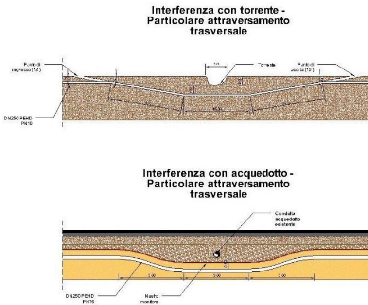
Figura 34 - Particolare attraversamento trasversale in prossimità di interferenza con torrente e di interferenza con acquedotto.
