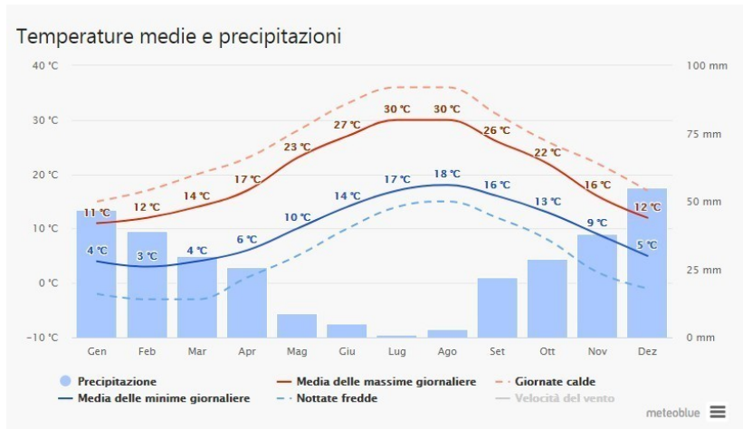
Figura 37 - Temperature medie e precipitazioni
