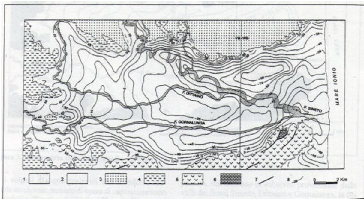
Figura 15 - Carta geologica schematica della Piana di Catania. 1) Depositi alluvionali attuali; 2) Depositi alluvionali recenti e terrazzati; 3) Depositi sabbioso-conglomeratici delle Terreforti; 4) Termini prevalentemente argillosi; 5) Complesso vulcanico-calcarenitico; 6) Termini carbonatici della serie iblea; 7) Faglia; 8) Isoipsa del tetto del substrato e relativa quota assoluta (Ferrara V., 1999).
