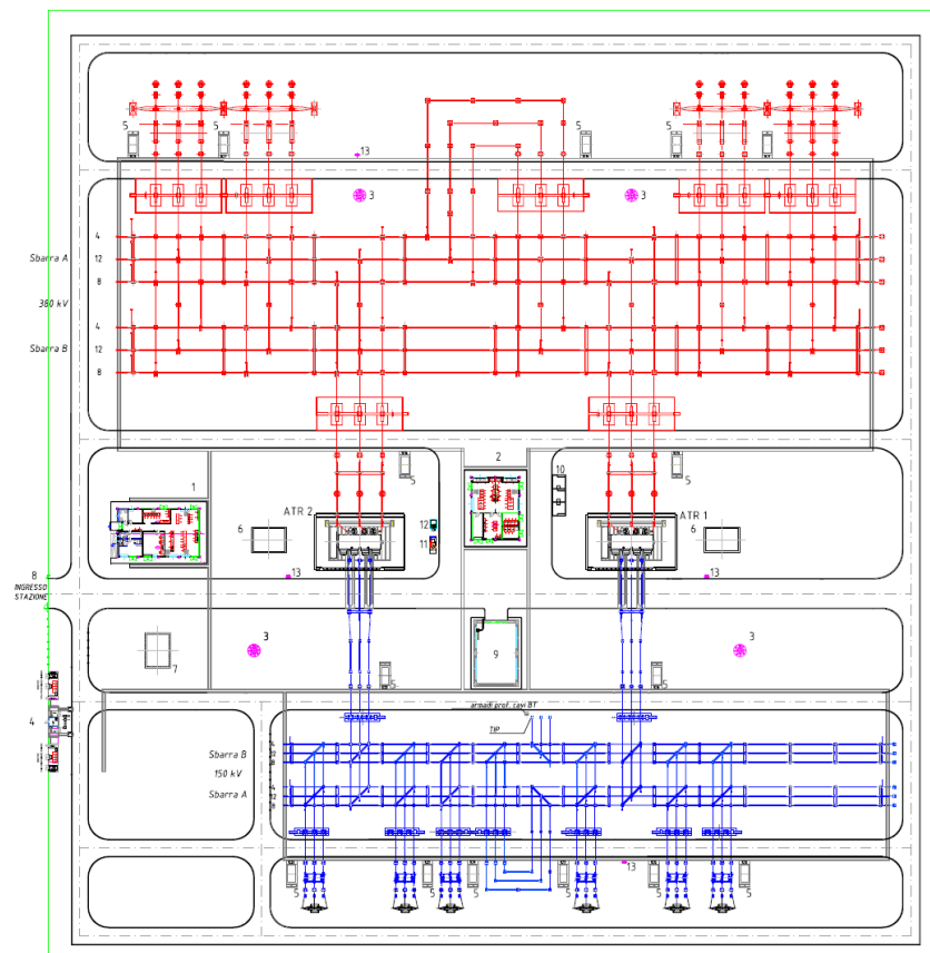
Figura 3 - Planimetria generale Stazione di Rete
