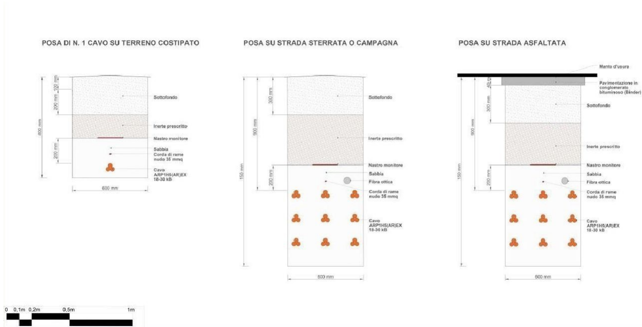
Figura 7 - Sezione tipica di posa della linea in cavo
