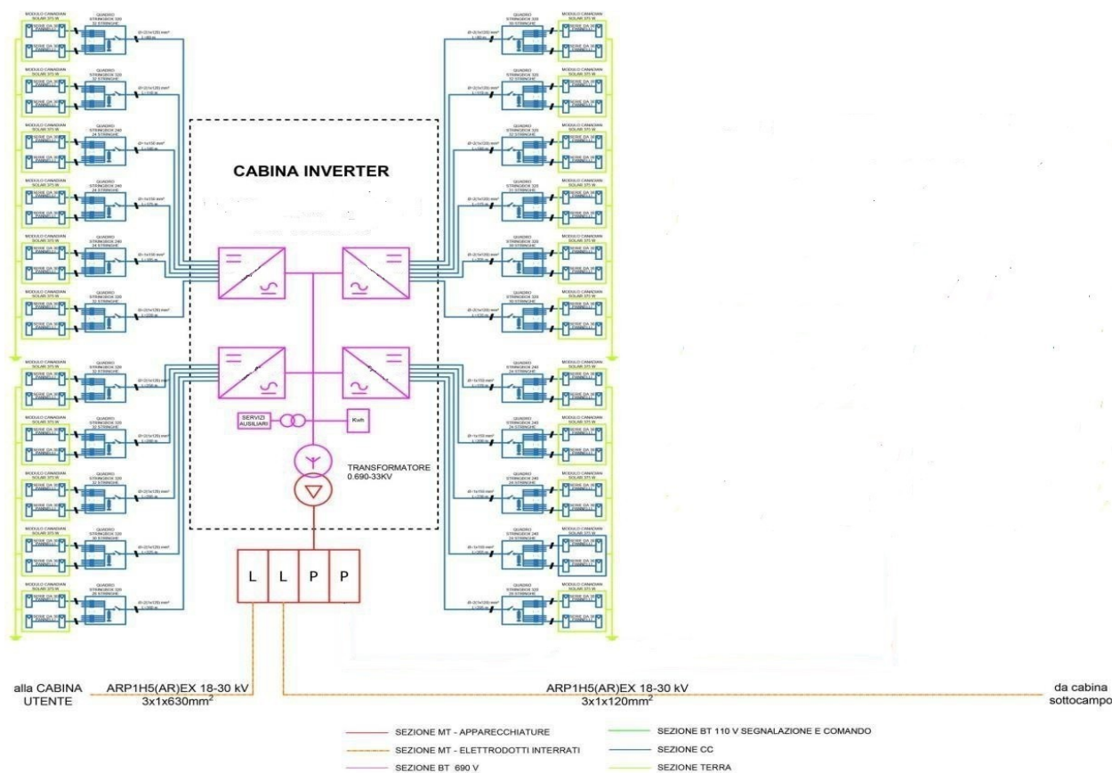
Figura 5 - Schema unifilare di principio dell'impianto fotovoltaico
