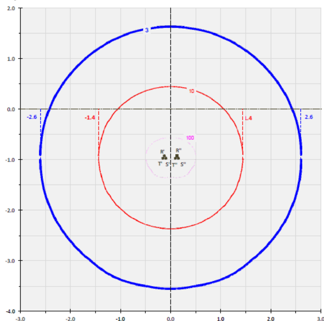
Figura 10 - Curve di equilivello per il campo di induzione magnetica generato da una linea MT posata a trifoglio ( I_{max}=710 \text{ A} ; formazione (3 \times 1 \times 630) )
