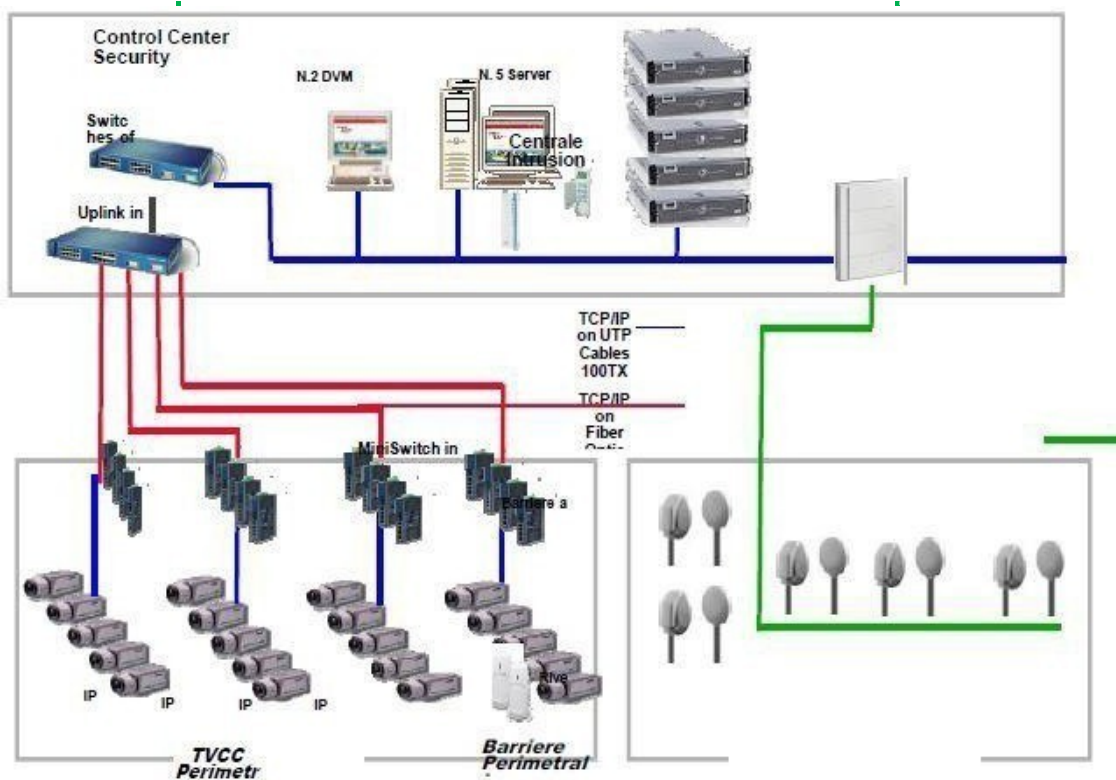
Figura 2 - Schema del Sistema di sorveglianza
