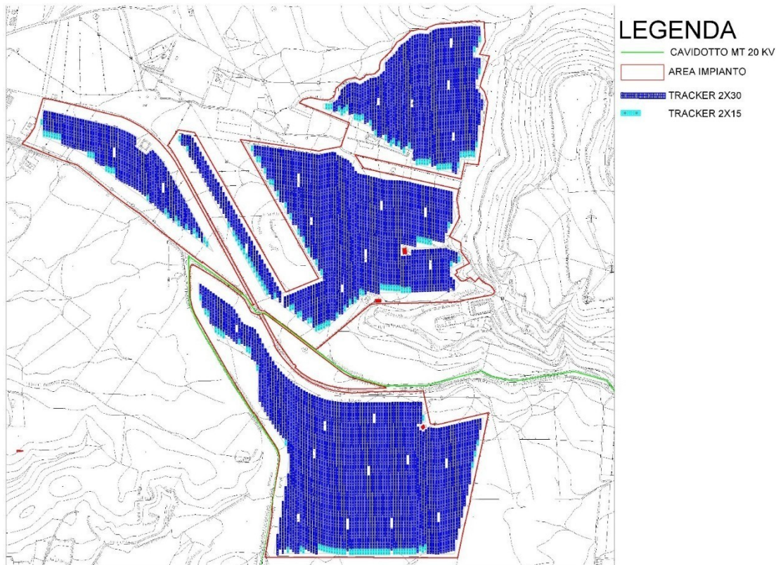
Figura 6 B - Layout dell'area d'impianto su C.T.R. ricadente sul territorio di Licodia Eubea (CT) - località Marineo.
