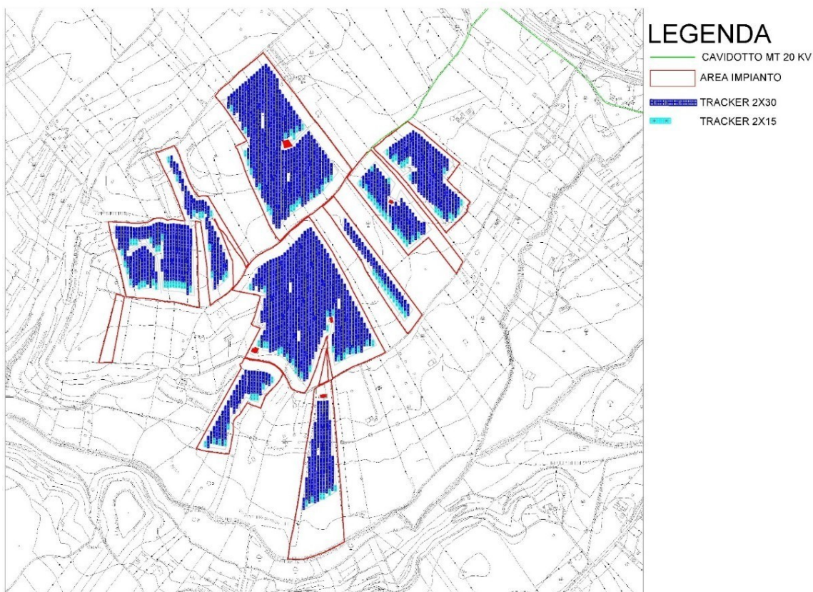
Figura 6 A - Layout dell'area d'impianto su C.T.R. ricadente sul territorio di Caltagirone (CT) - località Ramione.
