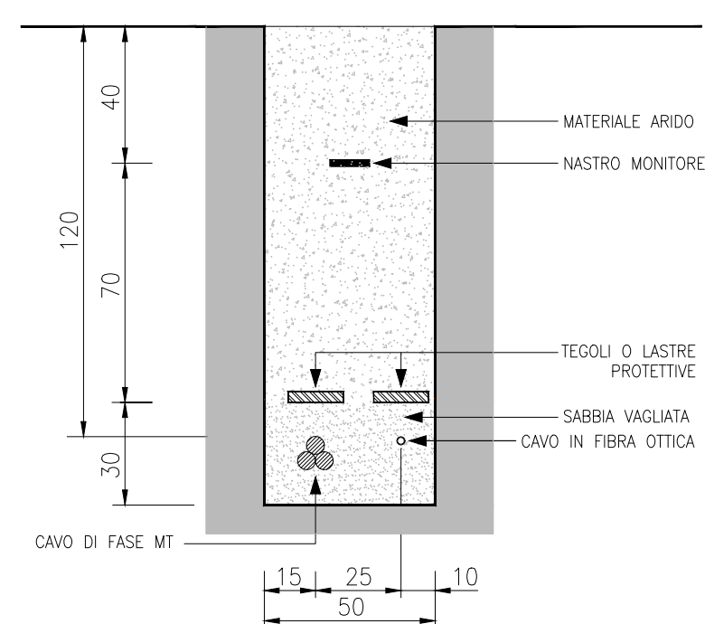
SEZIONI TIPO CAVIDOTTI MT SU PISTA
