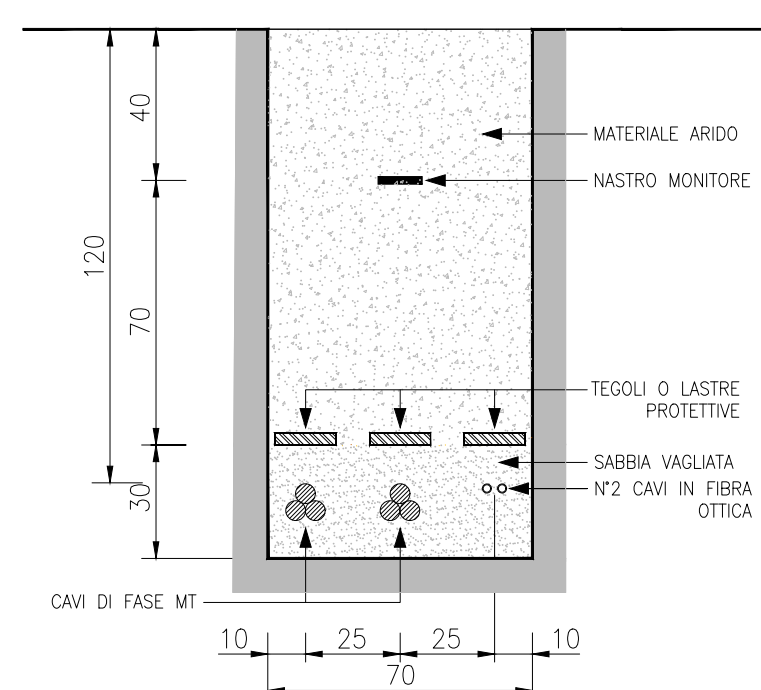
SEZIONI TIPO CAVIDOTTI MT SU PISTA
