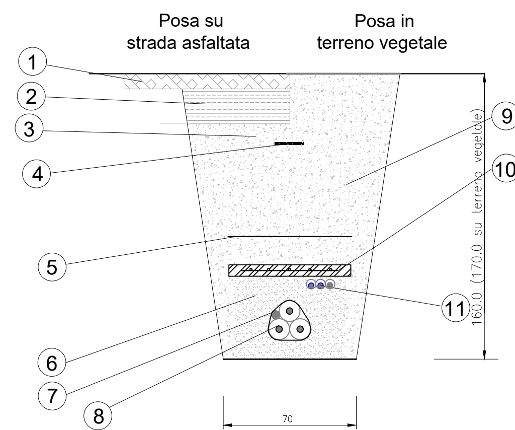
SEZIONE CAVIDOTTO AT
