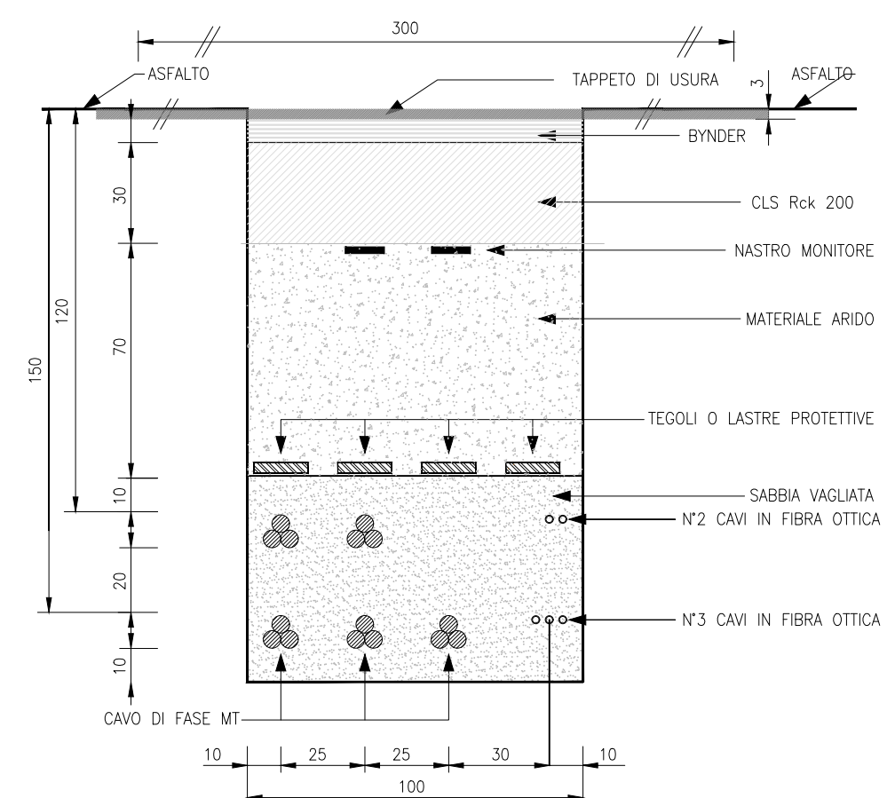
SEZIONI TIPO CAVIDOTTI SU STRADE ASFALTATE
