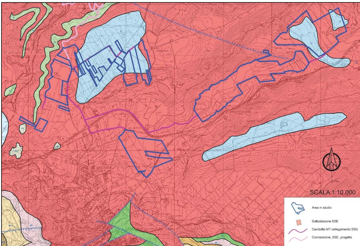
Figura 6 Carta Geologica
