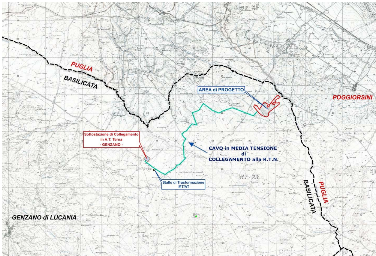
Fig. 1 – Planimetria generale dell'impianto fotovoltaico su CTR.
