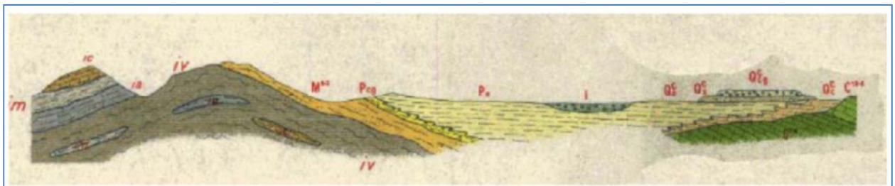
Figura 8: Rapporti stratigrafici
