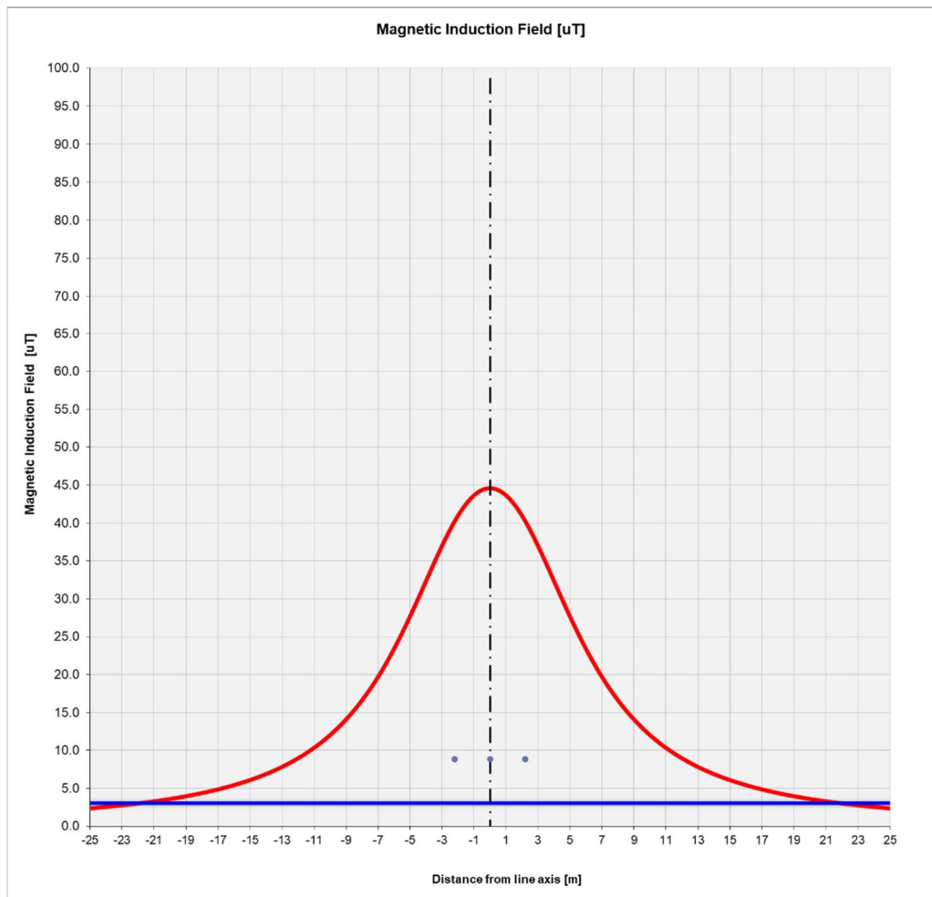
Figura 7: Andamento del campo di induzione magnetica per I = 2000 A
