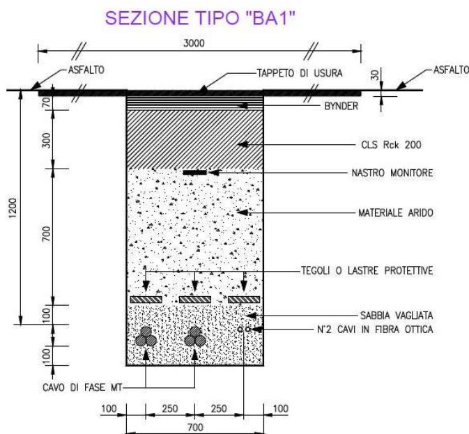
Figura 2: Sezione tipica di posa della linea in cavo su sede stradale
