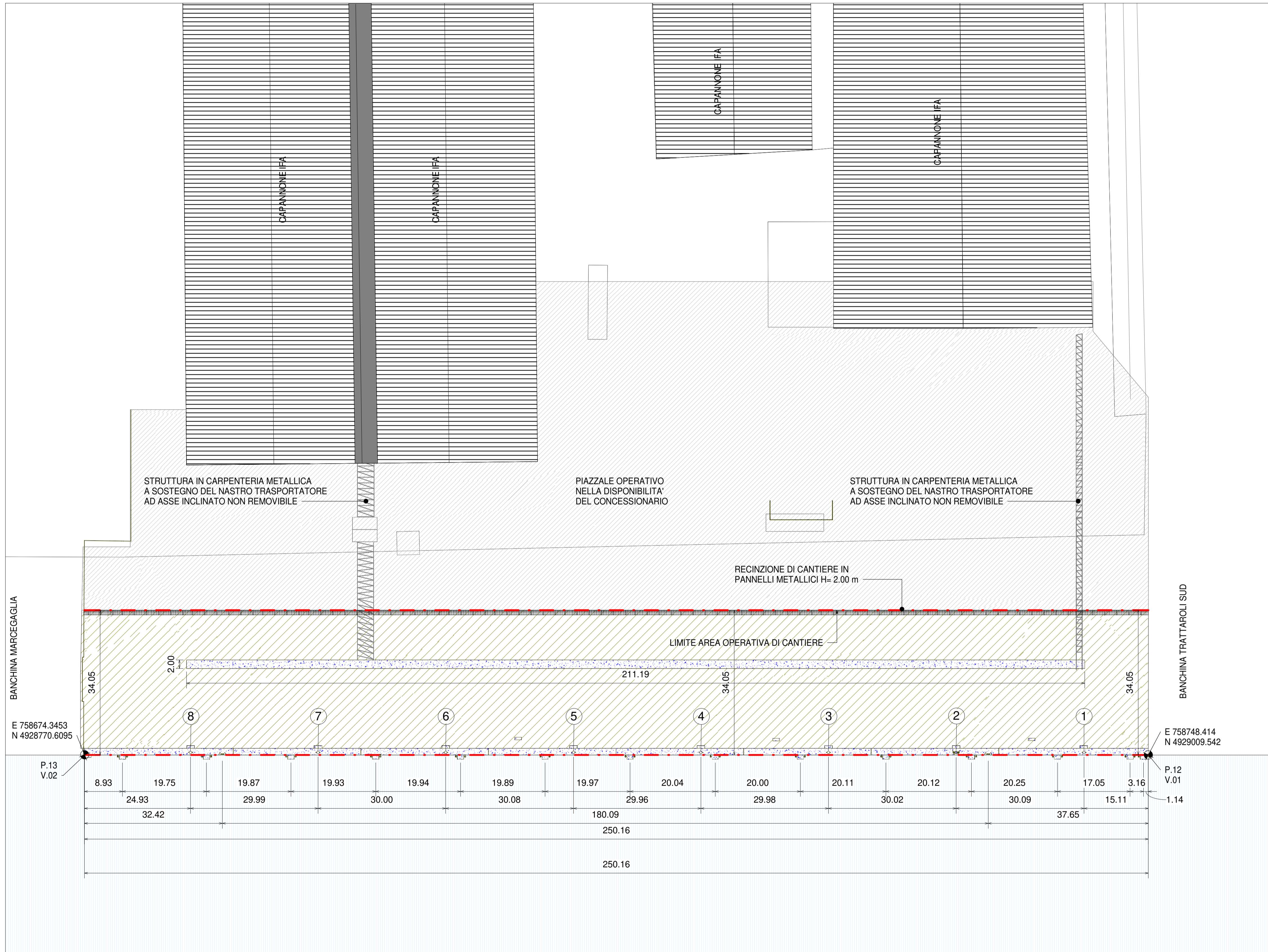
Planimetria generale delle demolizioni e degli scavi 1 : 500
