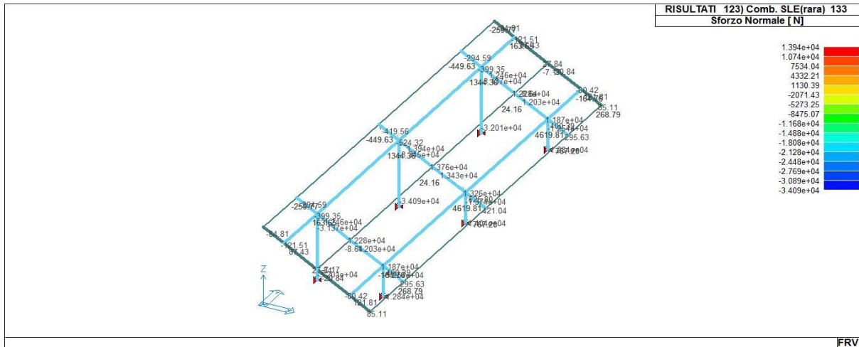
43_RIS_N_123_Comb. SLE(rara) 133
