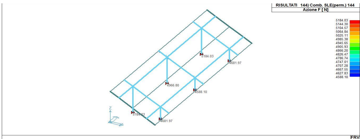
42_RIS_REAZIONI_144_Comb. SLE(perm.) 144
