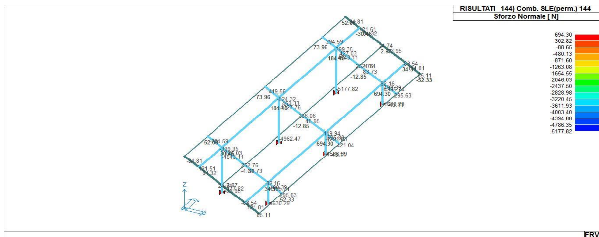
43_RIS_N_144_Comb. SLE(perm.) 144
