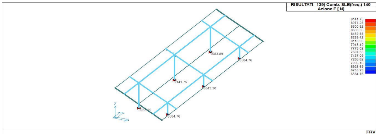
42_RIS_REAZIONI_139_Comb. SLE(freq.) 140
