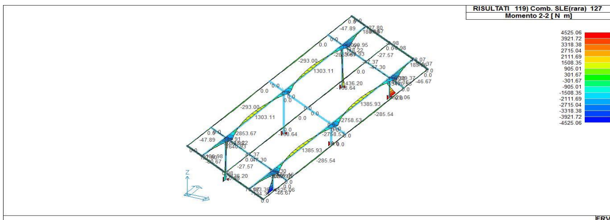
43_RIS_M2_119_Comb. SLE(rara) 127
