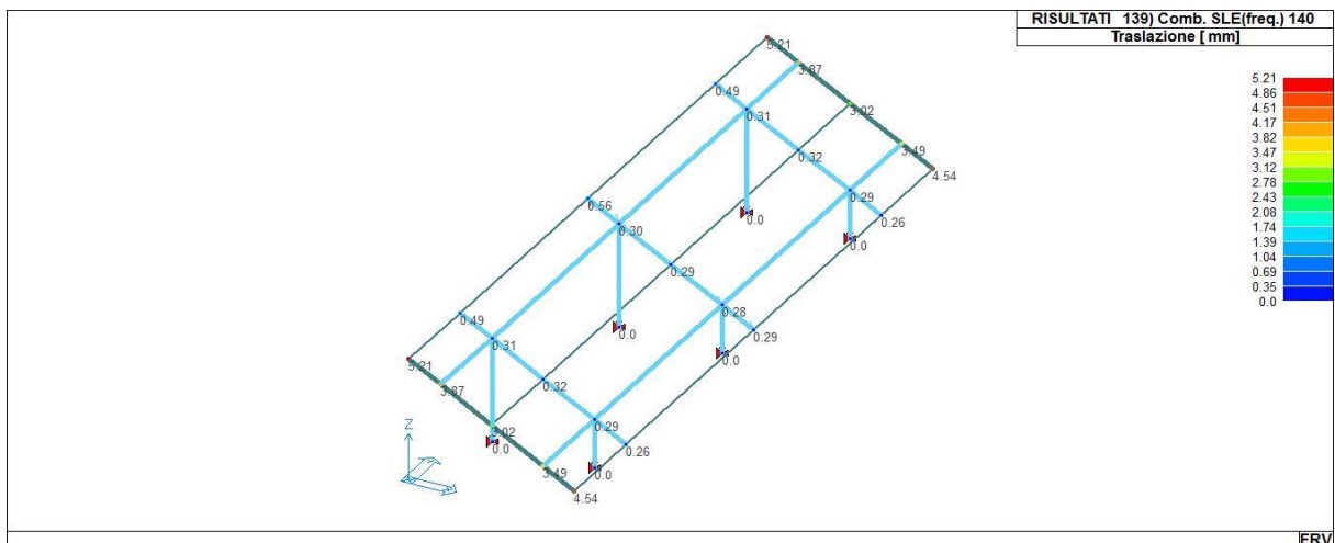
41_RIS_SPOSTAMENTI_139_Comb. SLE(freq.) 140
