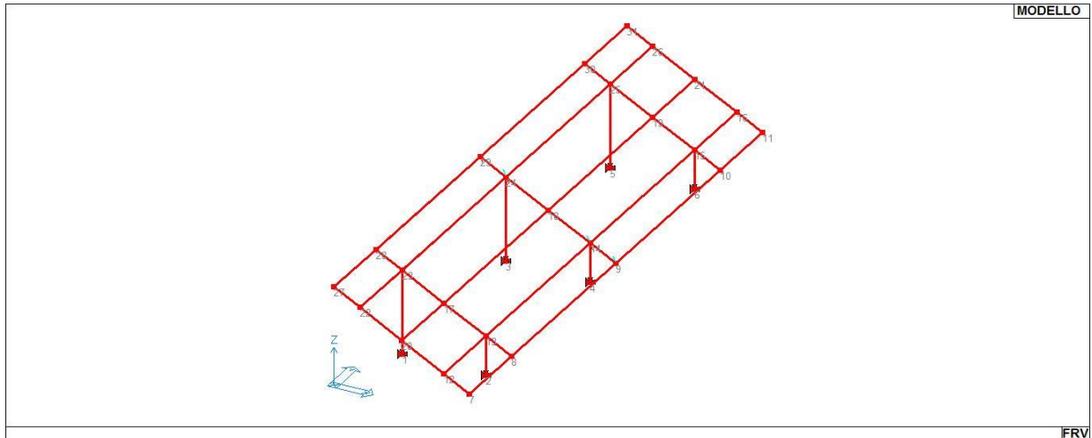
14_MOD_NUMERAZIONE_NODI
