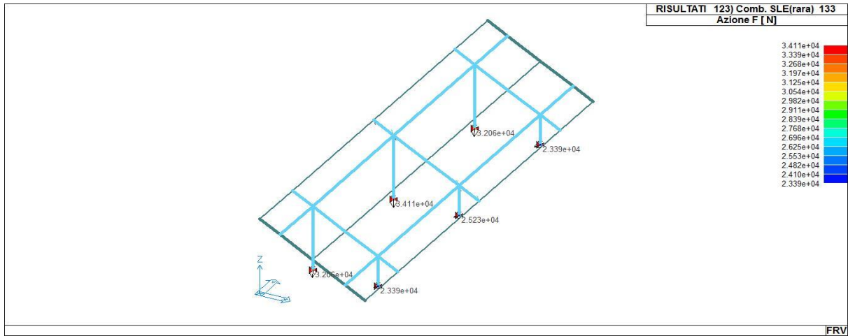
42_RIS_REAZIONI_123_Comb. SLE(rara) 133
