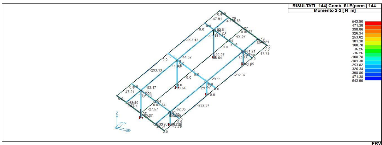
43_RIS_M2_144_Comb. SLE(perm.) 144
