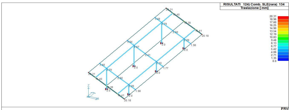
41_RIS_SPOSTAMENTI_124_Comb. SLE(rara) 134
