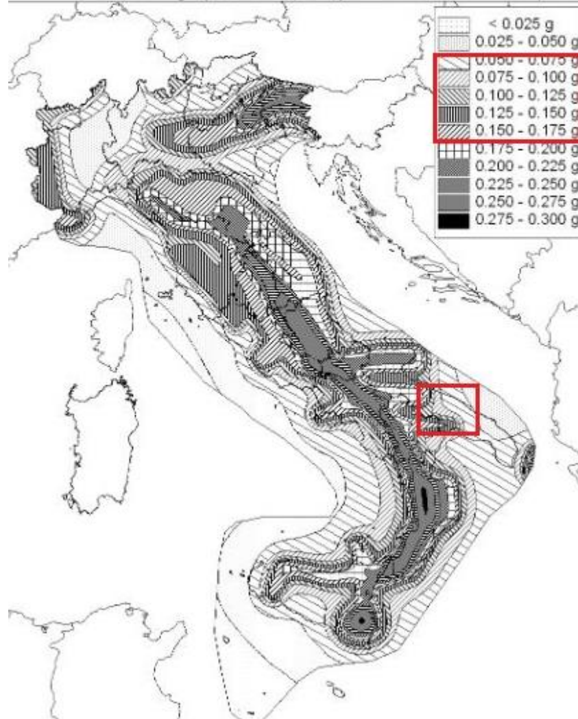
Figura 2 Mappa sismica OPCM 3519 del 28 aprile 2006
