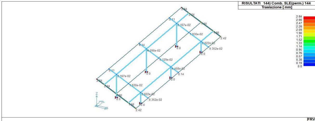
41_RIS_SPOSTAMENTI_144_Comb. SLE(perm.) 144
