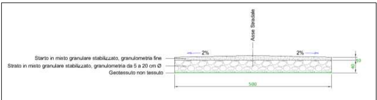
Fig.: Tipico della sezione stradale
