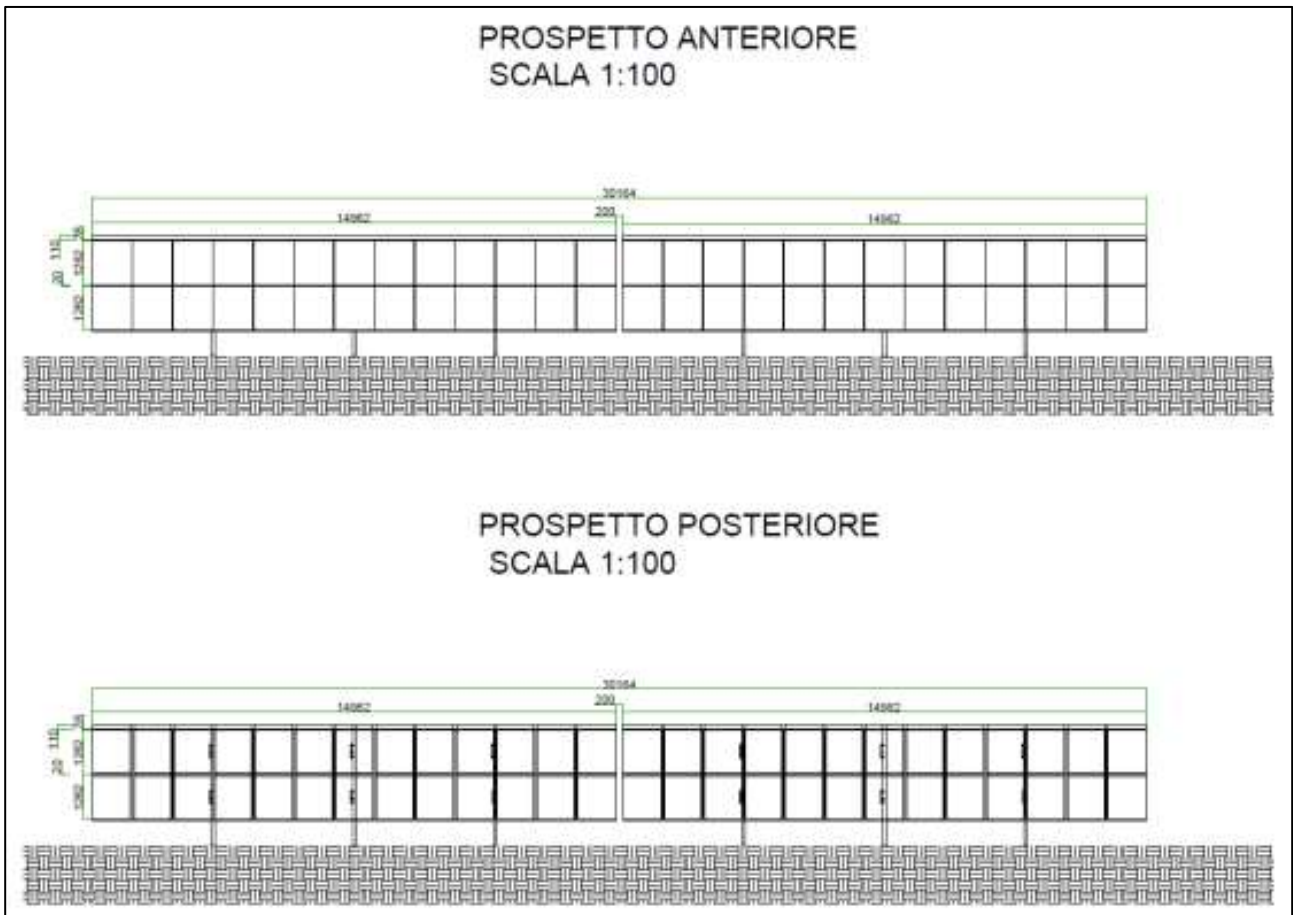
Fig.: Disegno costruttivo strutture fisse - vista frontale
