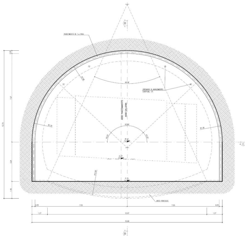
FIGURA 2-13 - SEZIONE TIPO A1B-BIS
