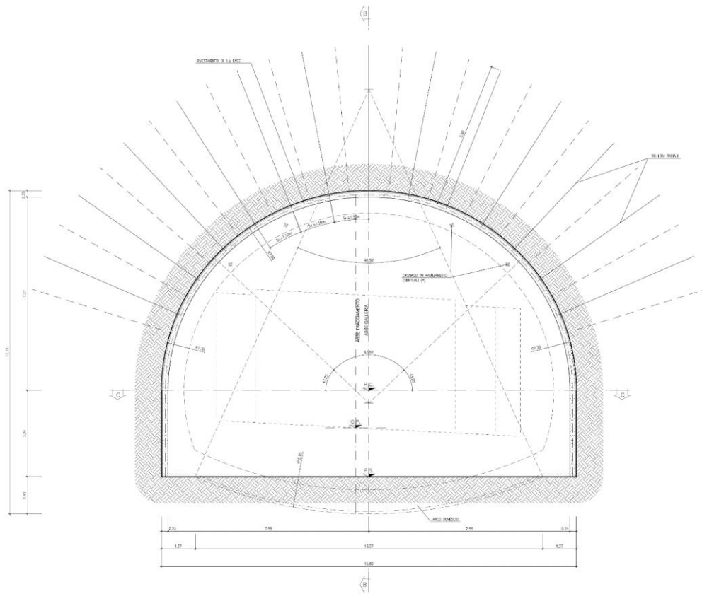
FIGURA 2-12 - SEZIONE TIPO A2B
