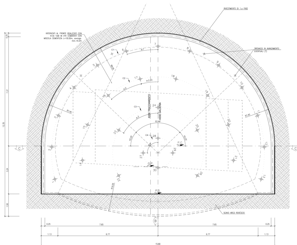
FIGURA 2-17 - SEZIONE TIPO B2*B
