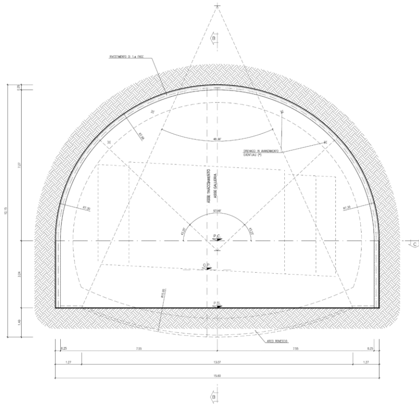
FIGURA 2-14 - SEZIONE TIPO A2B-BIS
