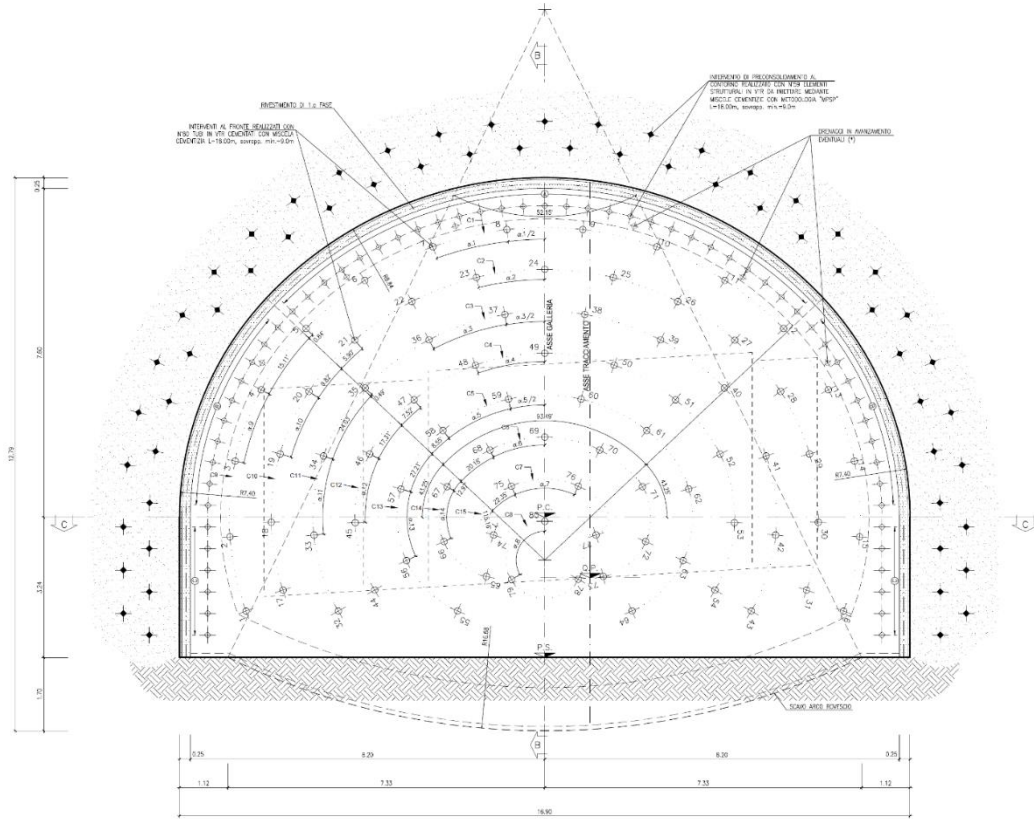
FIGURA 2-20 - SEZIONE TIPO C1A – GALLERIA MOLINELLO
