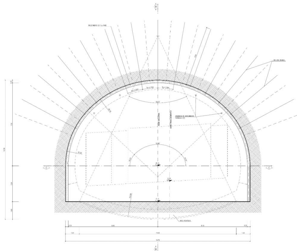
FIGURA 2-11 - SEZIONE TIPO A1A
