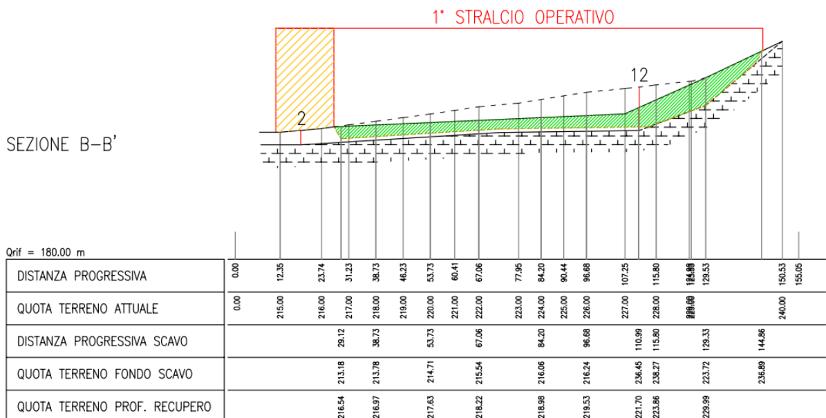
FIGURA 4-10 – PLANIMETRIA E SEZIONE DI RECUPERO CAVA IL PIANO DI SMIRRA POLO GH005-2
