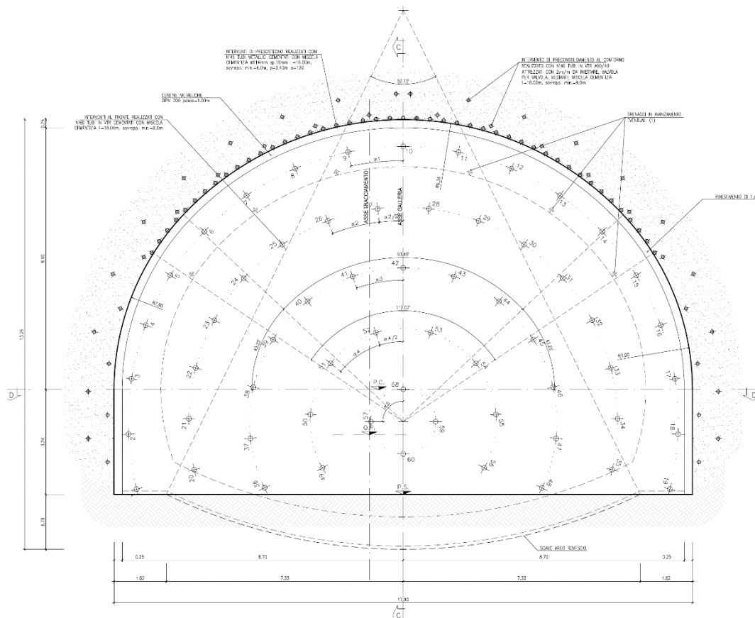
FIGURA 2-24 - SEZIONE TIPO C1*A - GALLERIA MOLINELLO
