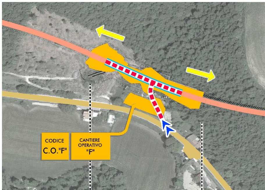
FIGURA 6-5 - VIABILITÀ PER IL COLLEGAMENTO ALLA ZONA DEGLI IMBOCCHI "PIETRALUNGA 2" EST E "MOLINELLO" OVEST (ESTRATTO DALL'ELABORATO T00CA01CANPL01)
