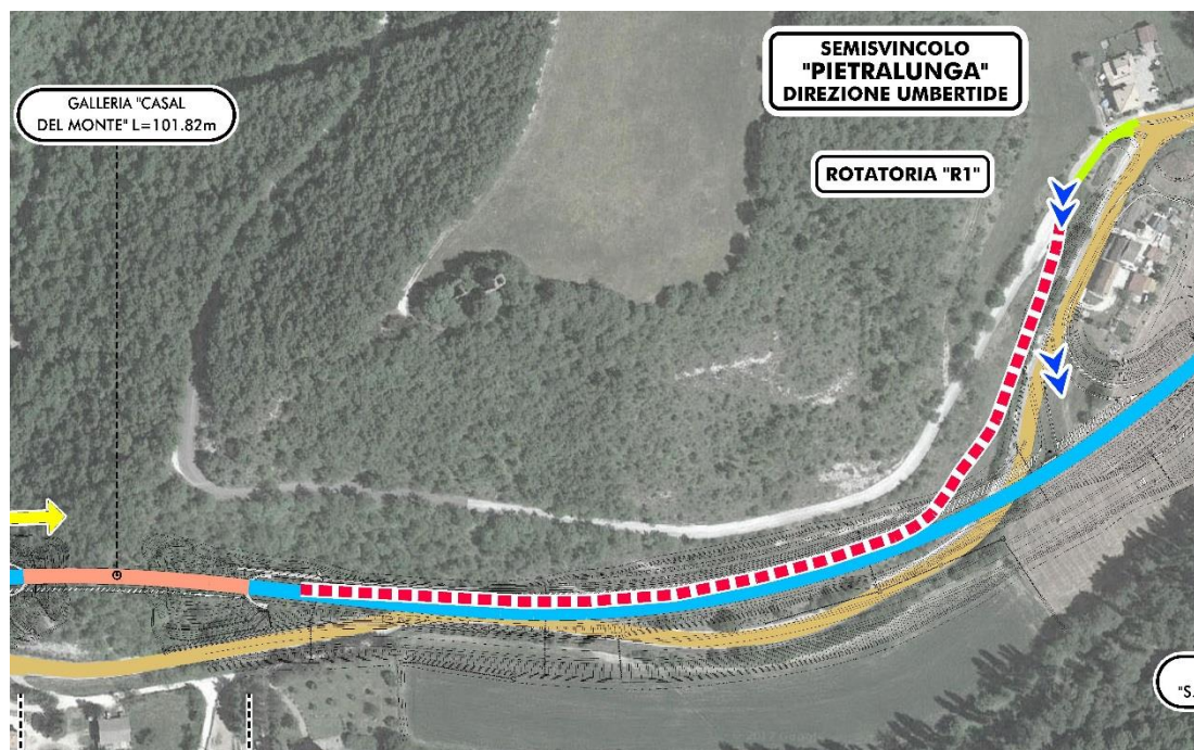
FIGURA 6-2 PISTA DI CANTIERE PER IL COLLEGAMENTO DELL'AREA DI LAVORO PRESSO L'IMBOCCO EST DELLA GALLERIA MOLINELLO (ESTRATTO DALL'ELABORATO T00CA01CANPL01)
