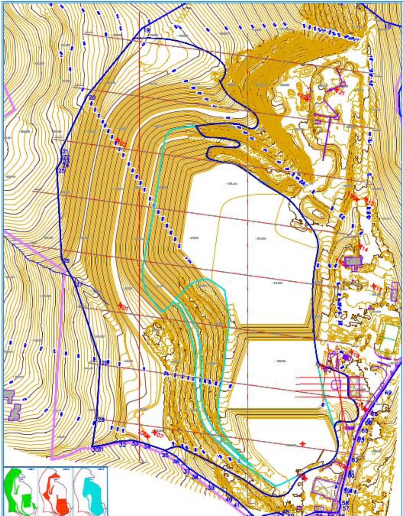
FIGURA 4-4 – CAVA SAN MARCO - PIANO DI SISTEMAZIONE FINALE
