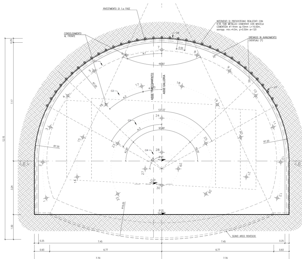
FIGURA 2-19 - SEZIONE TIPO B2B
