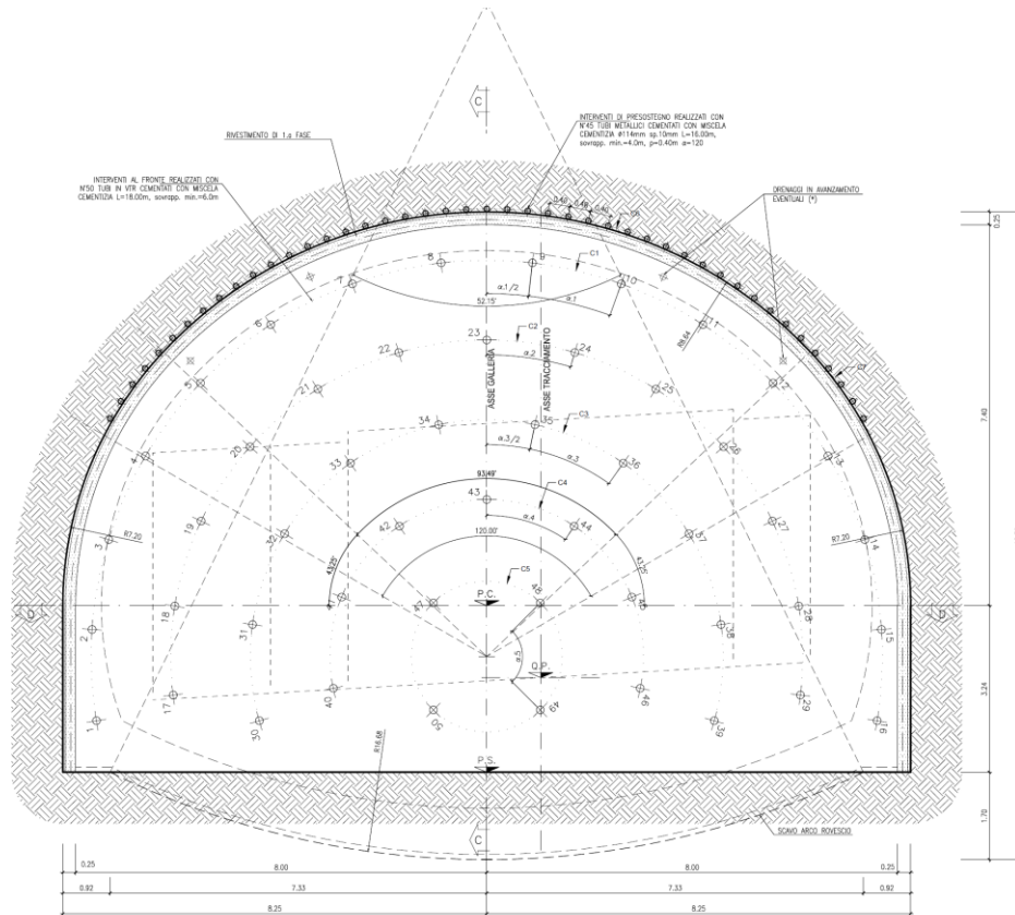
FIGURA 2-18 - SEZIONE TIPO B2A
