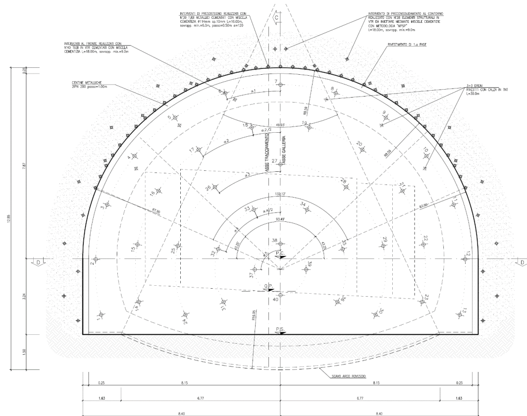
FIGURA 2-25 - SEZIONE TIPO C1*B
