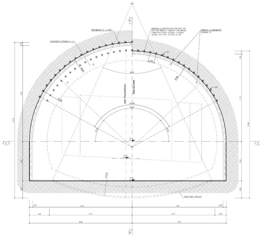
FIGURA 2-15 - SEZIONE TIPO B1B
