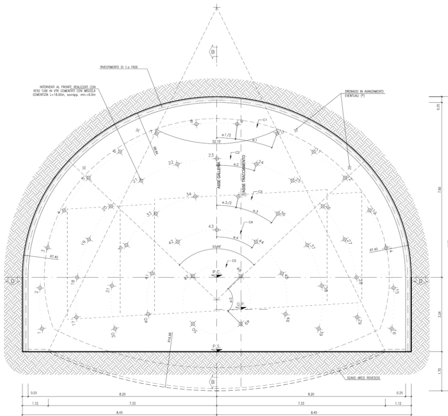
FIGURA 2-16 - SEZIONE TIPO B2*A
