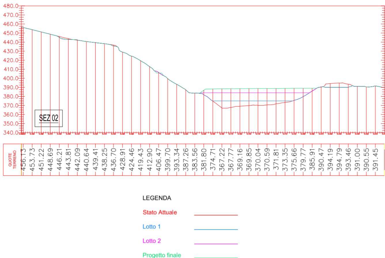
FIGURA 4-5 – CAVA SAN MARCO – SEZIONE DI PROGETTO
