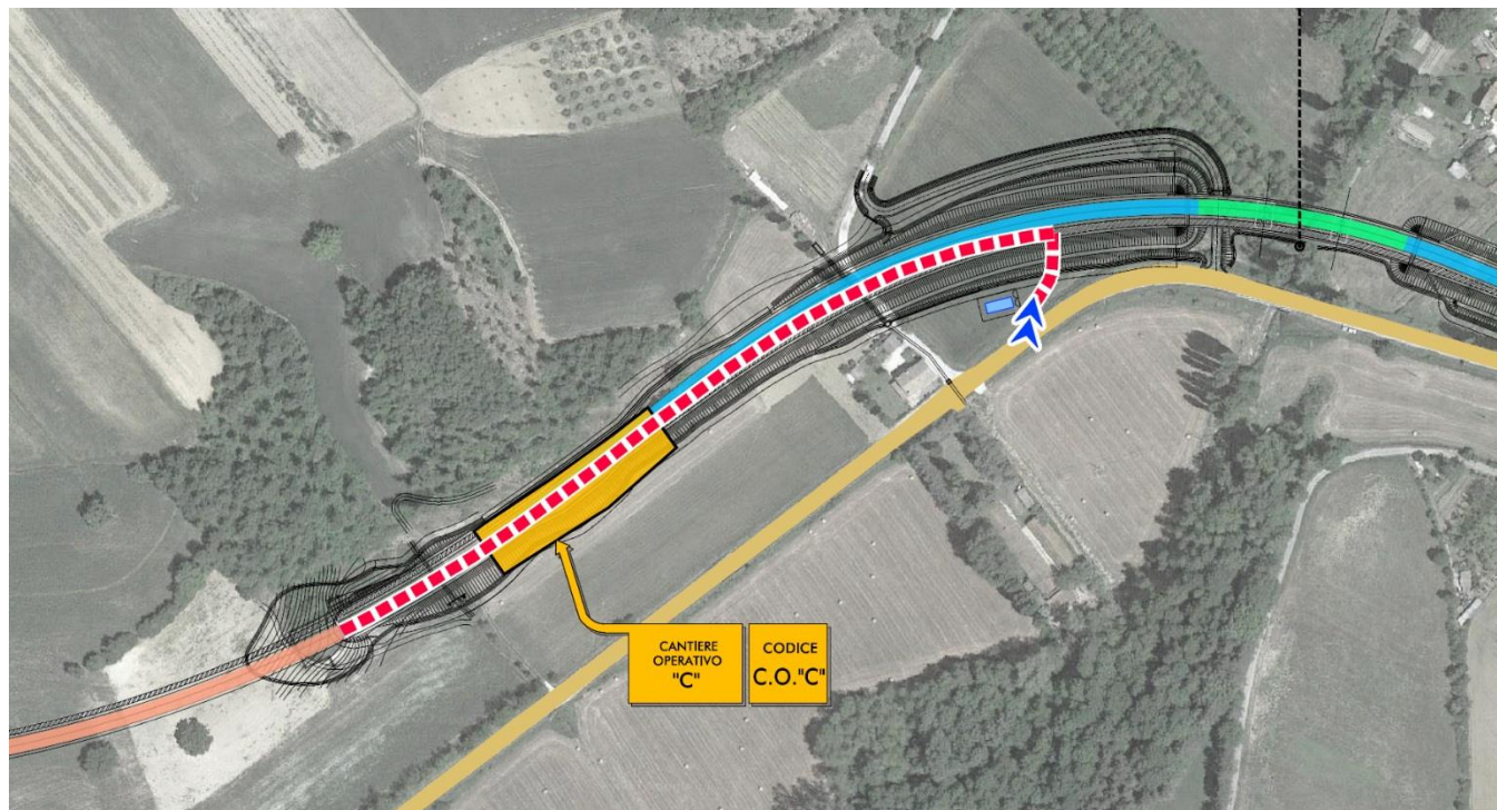
FIGURA 6-6 PISTA DI CANTIERE PER IL COLLEGAMENTO ALL'IMBOCCO "MOLINELLO" EST (ESTRATTO DALL'ELABORATO T00CA01CANPL01)
