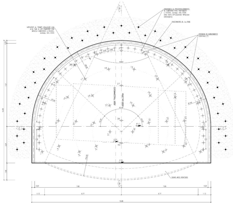
FIGURA 2-22 - SEZIONE TIPO C1B
