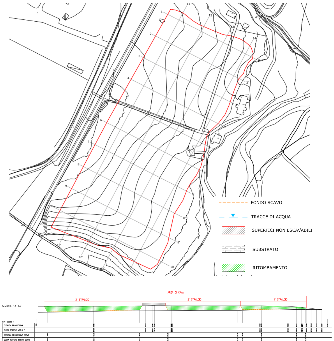
FIGURA 4-9 – PLANIMETRIA E SEZIONE DI RECUPERO CAVA IL PIANO POLO GH005-1
