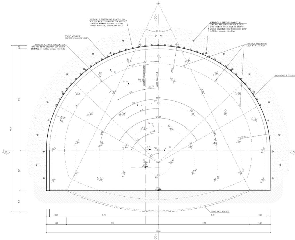
FIGURA 2-23 - SEZIONE TIPO C1*A – GALLERIA CASAL DEL MONTE
