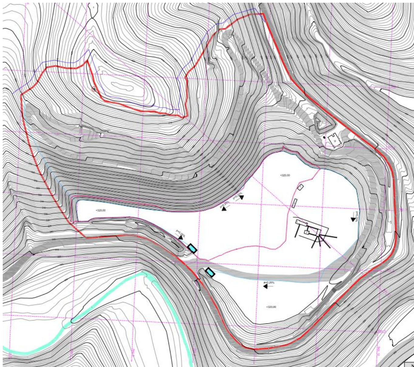
FIGURA 4-2 – PLANIMETRIA DI SISTEMAZIONE FINALE CAVA SCANNATA
