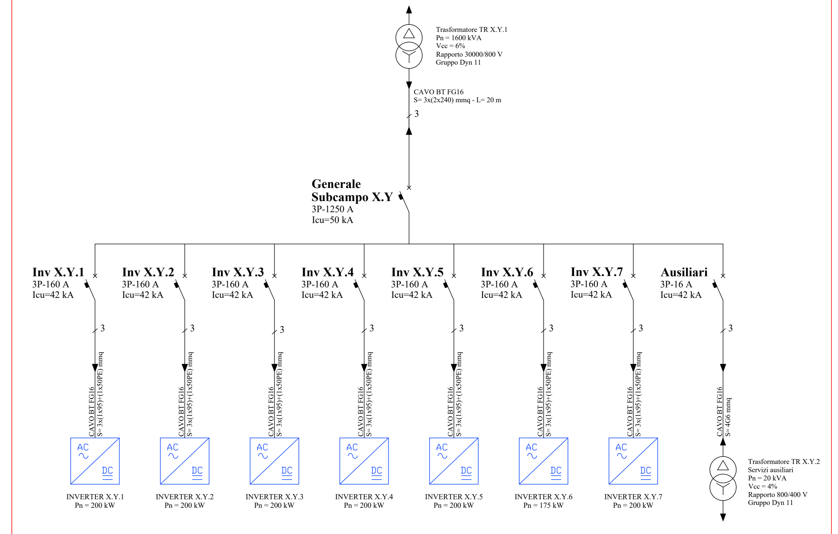
CABINA CT X.Y da 1,6 MVA
