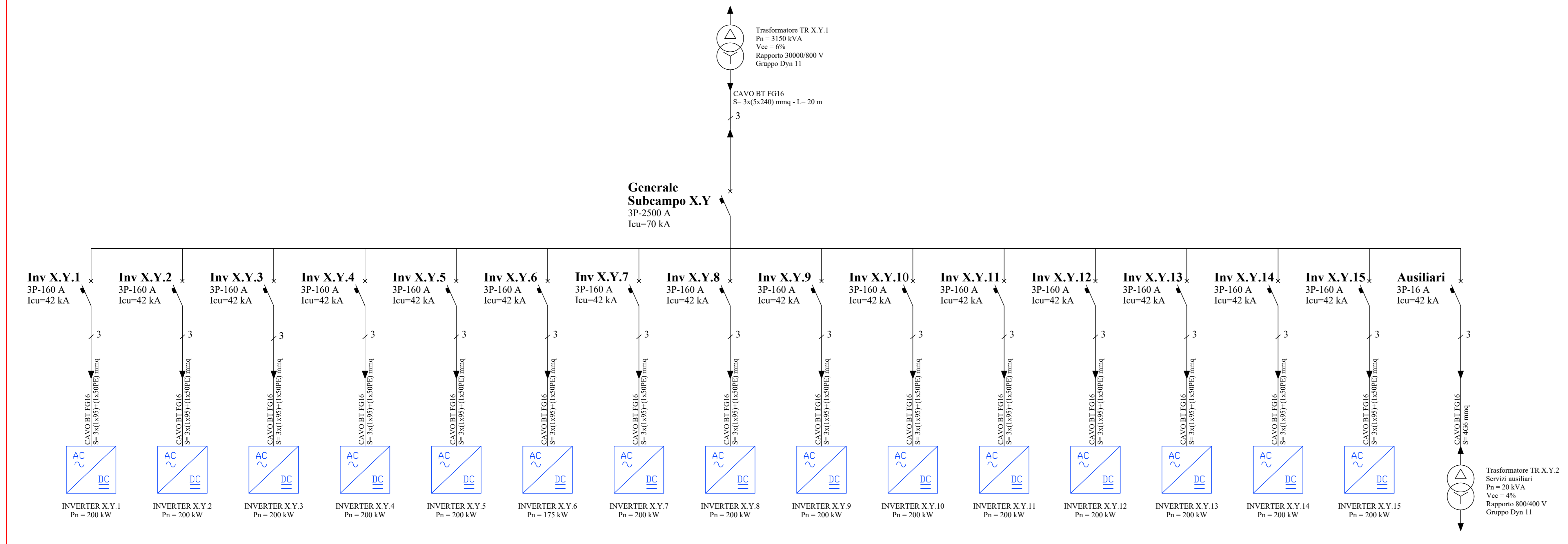
CABINA CT X.Y da 2,5 MVA
