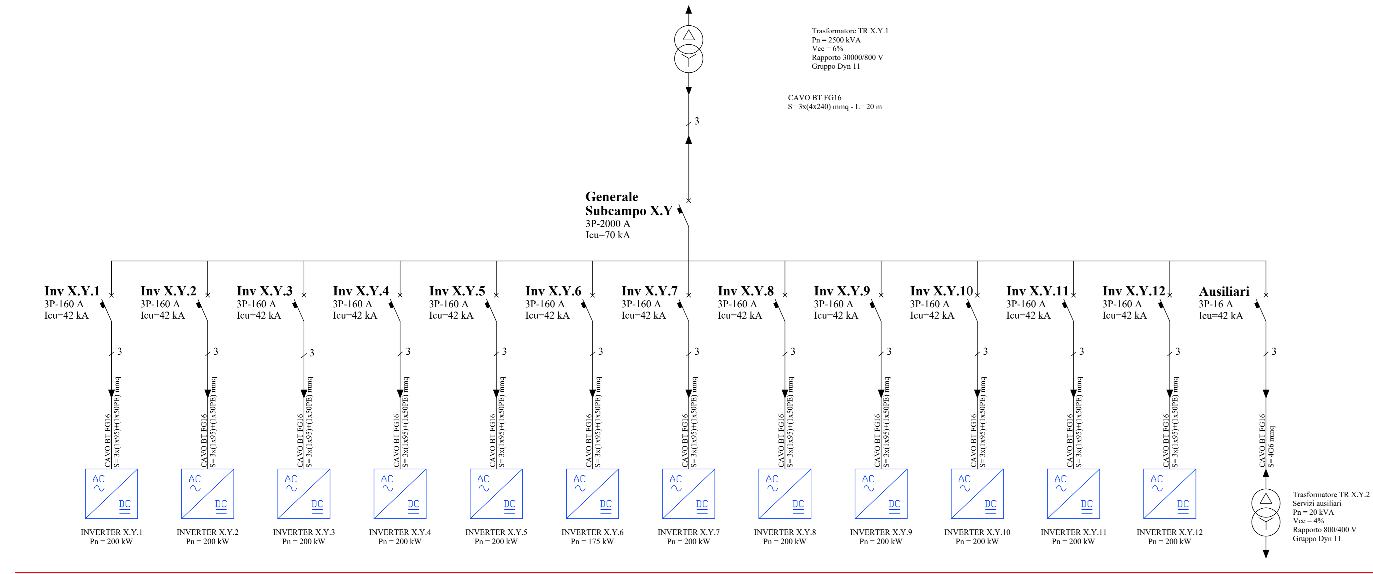
CABINA CT X.Y da 2,5 MVA
