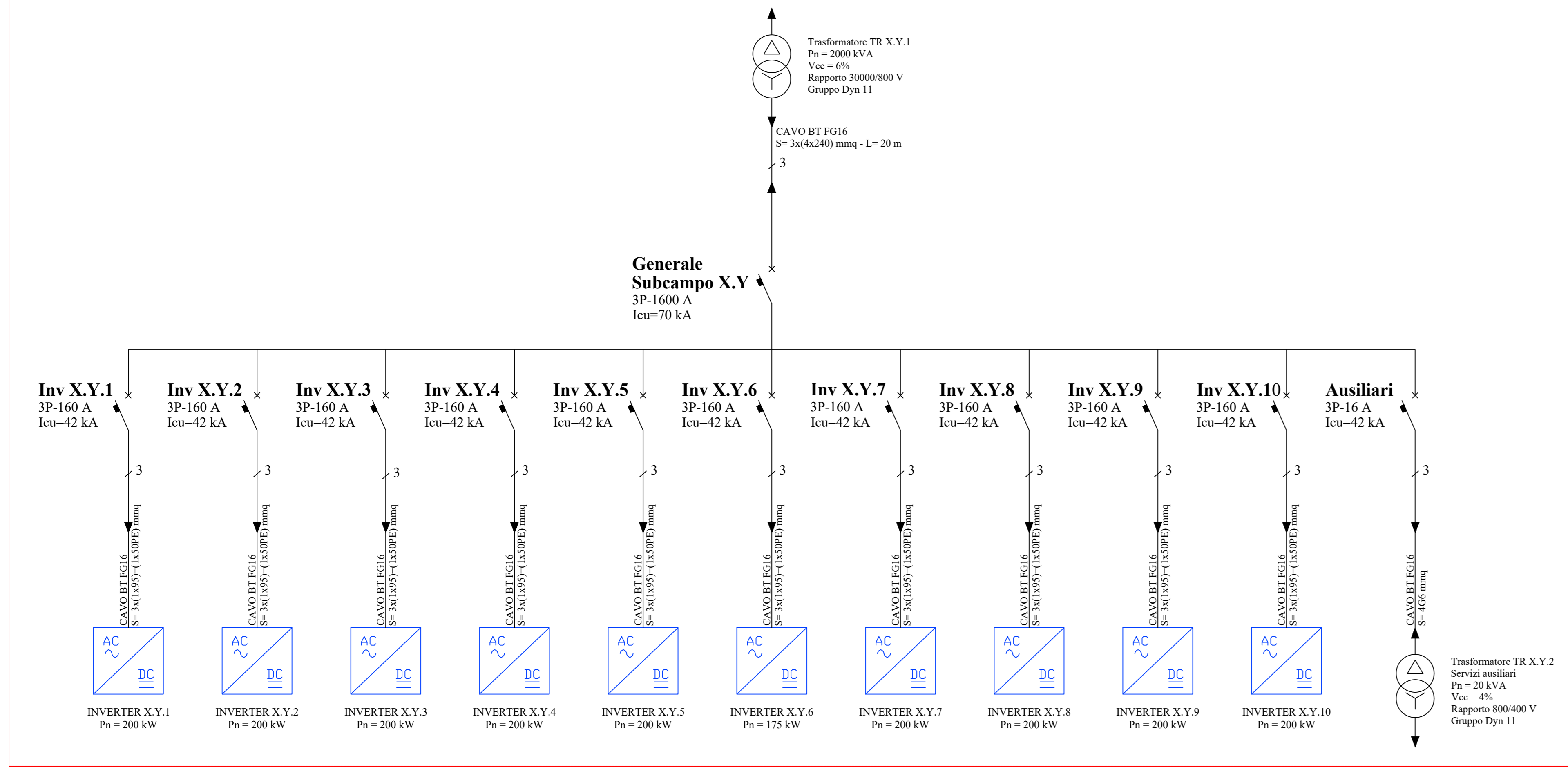
CABINA CT X.Y da 2 MVA
