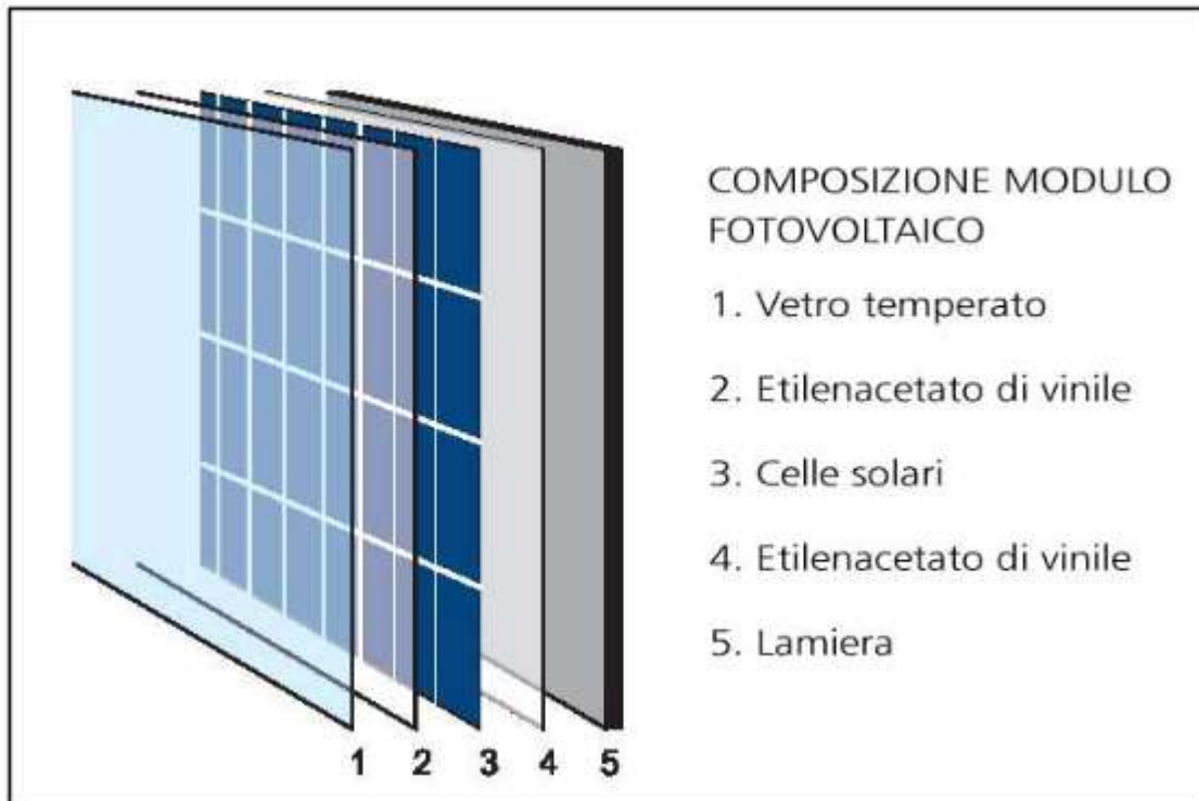
Composizione di un pannello fotovoltaico
