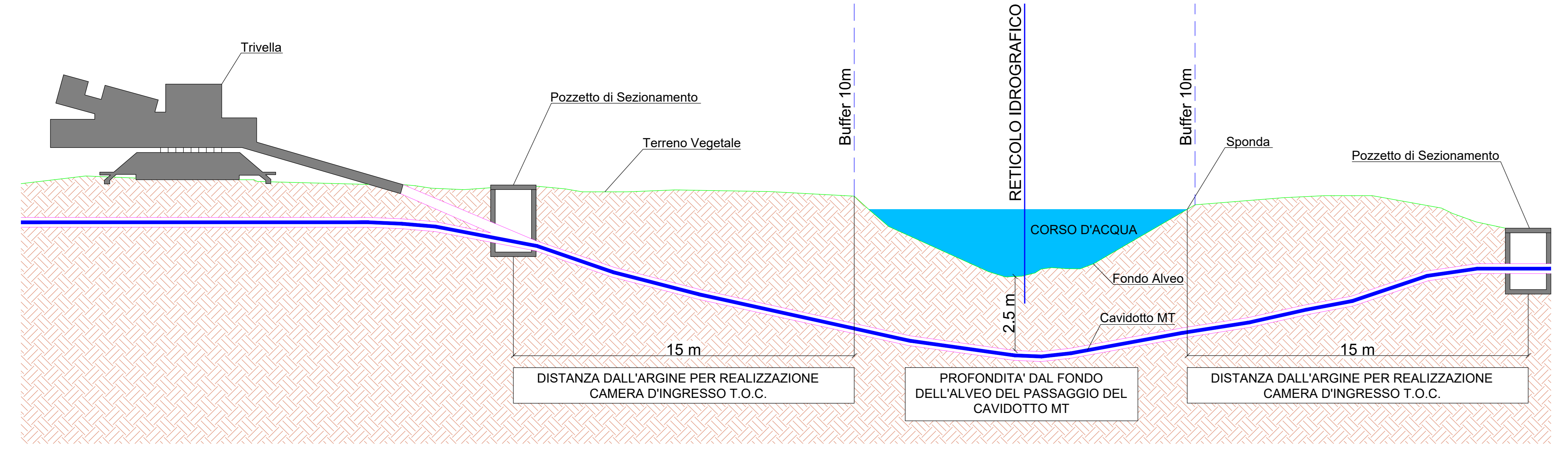
SEZIONE LONGITUDINALE ATTRAVERSAMENTO CON T.O.C. - Scala 1:100
