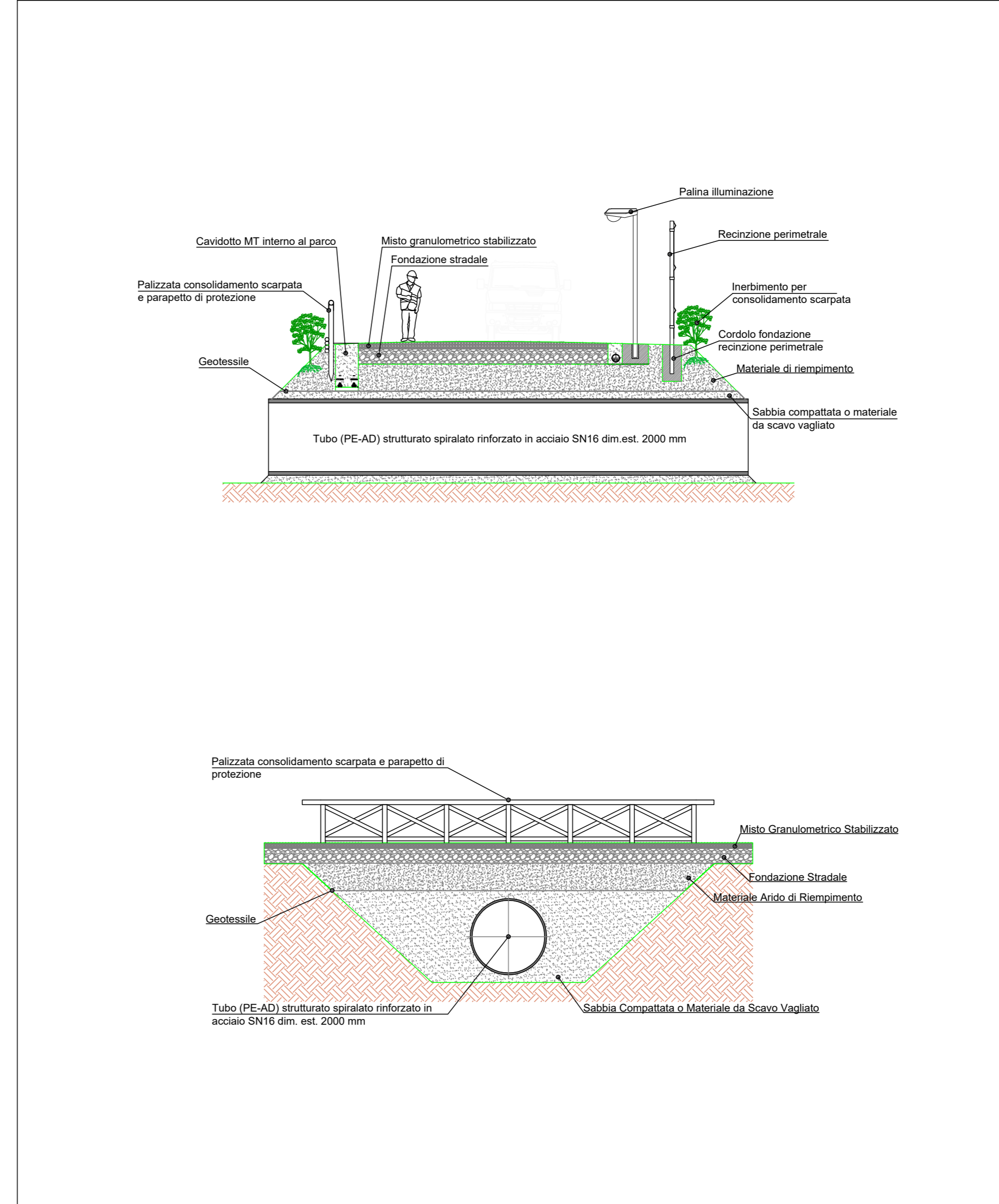
ATTRAVERSAMENTI INTERNI ALL'IMPIANTO SU RETICOLO IDROGRAFICO - Scala 1:100
