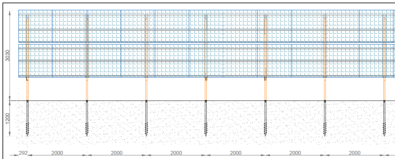
Figure 3: stralcio prospetto struttura di supporto
