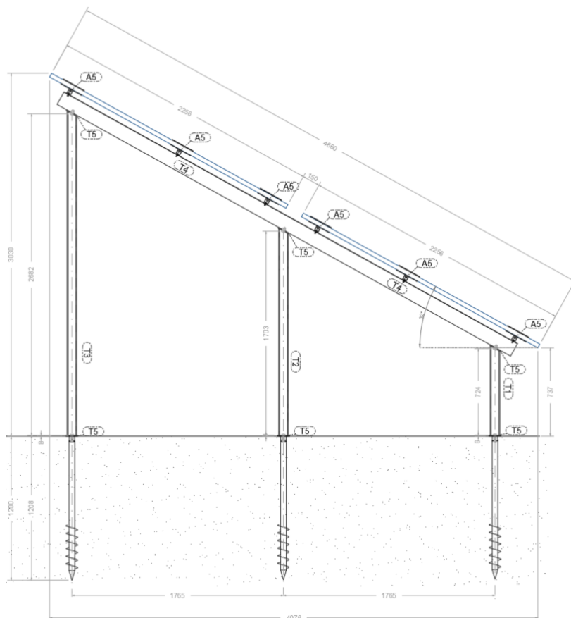
Figure 1: Sezione trasversale
