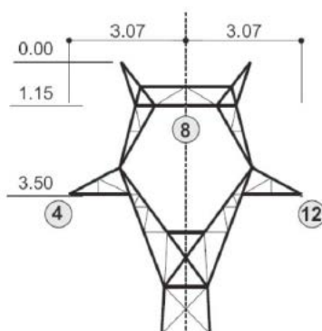
Geometria del palo gatto
