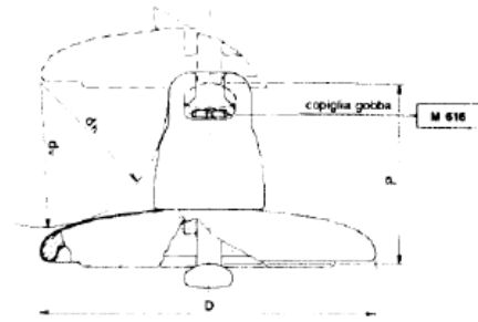
Isolatore
