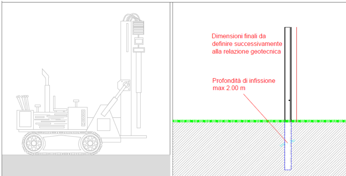
Figura 6-particolare costruttivo infissione pali
