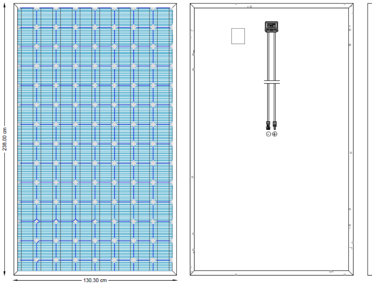
Figura 7- Particolare costruttivo pannello fotovoltaico
