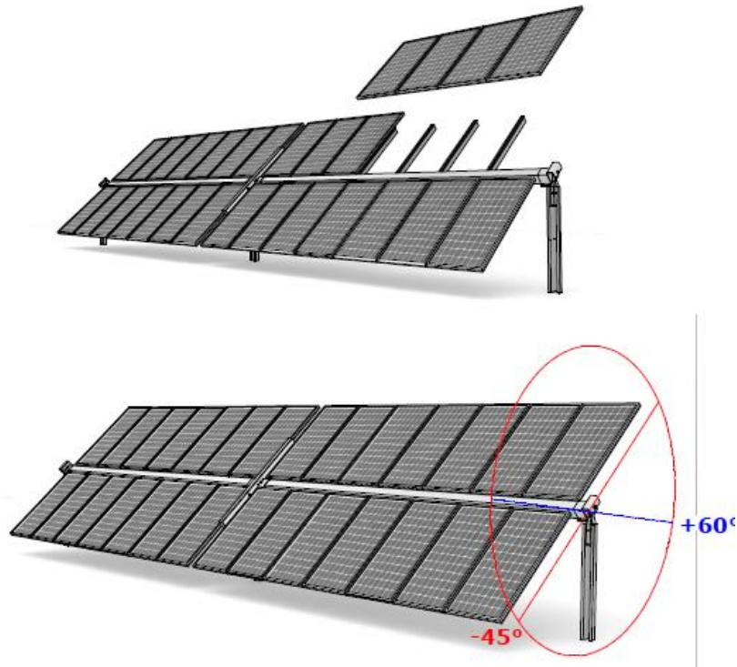
Figura 4- Componenti strutturali dell'impianto
