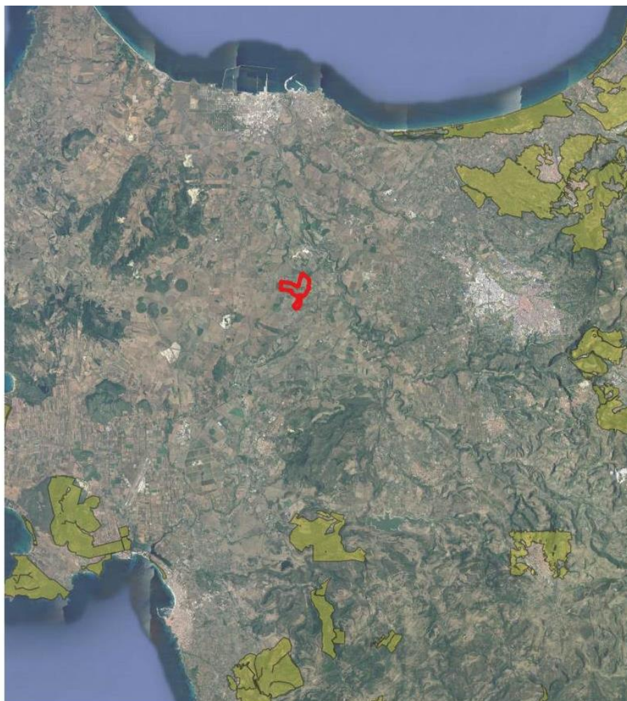
Figura 13 - Vincolo idrogeologico RD 3267
