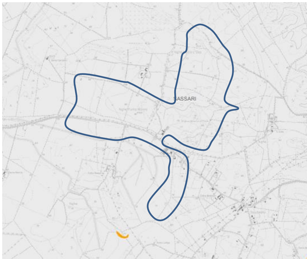
Figura 20 -Figura 21 – Carta della pericolosità geomorfologica (Hg) del settore per il P.A.I. Sardegna (fonte: Geoportale della R.A.S. Sardegna)
