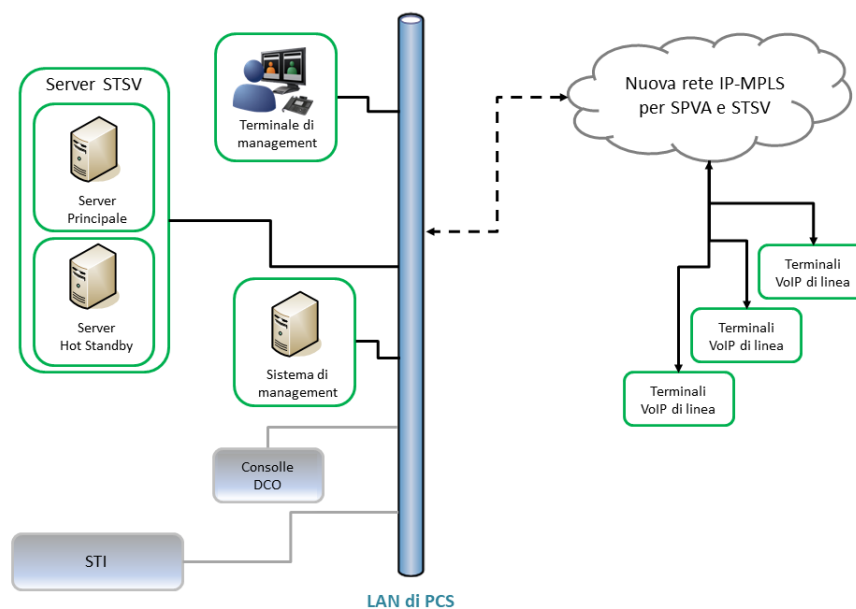
Figura 3: Architettura Sistema Telefonica Selettiva STSV
