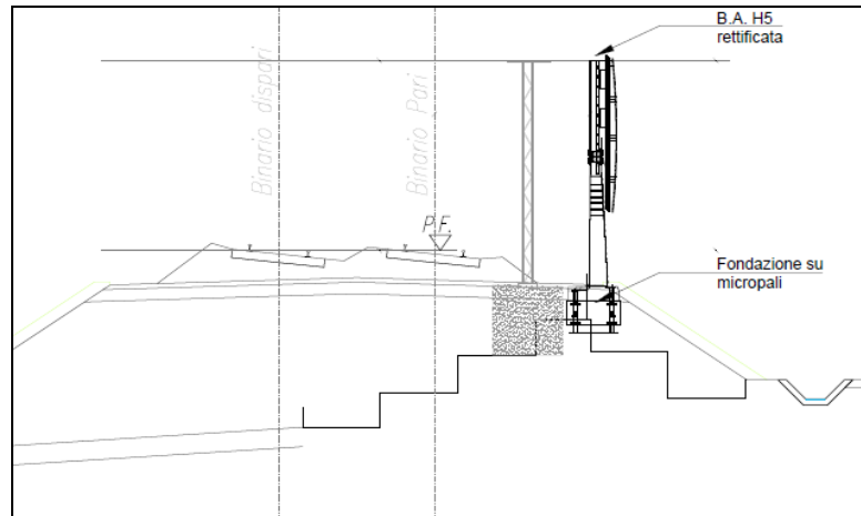
Figura 4 - Barriera acustica in assenza di muro di recinzione
