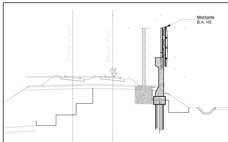
Figura 3 - Barriera acustica su muro di recinzione
