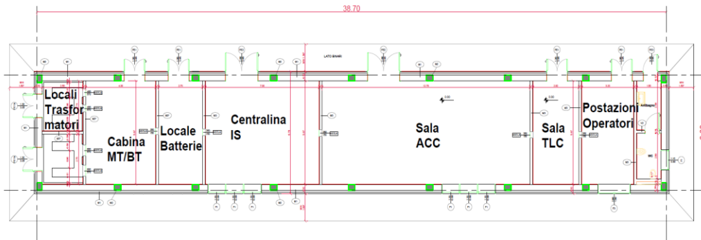
Figura 7 – Tipologico del Fabbricato Tecnologico
