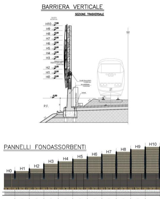
Figura 5 - Sezioni-tipo e prospetti dei moduli di barriera antirumore previsti nello Studio Acustico (evidenziati in rettangolo colore giallo)
