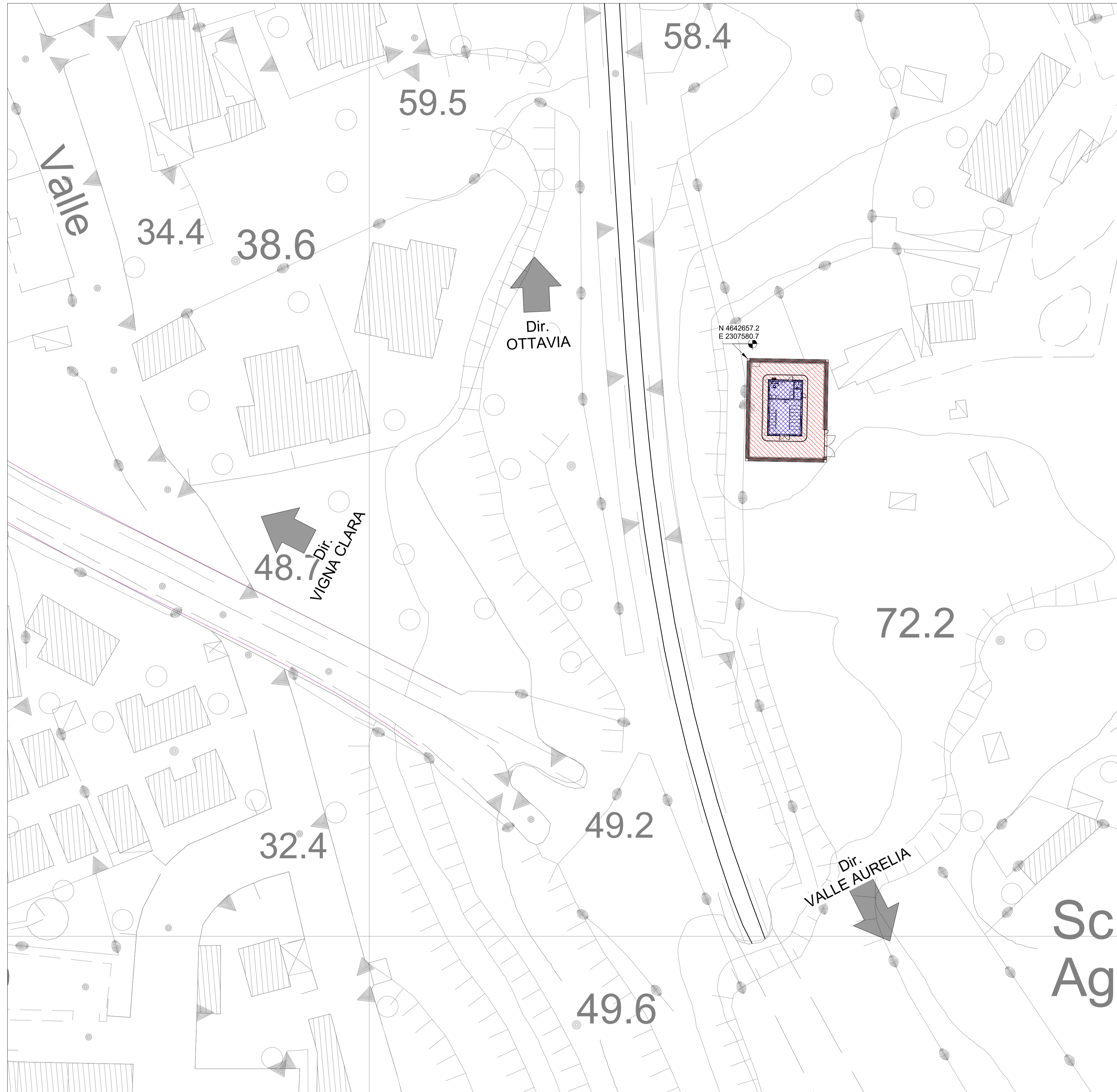
1 Ubicazione Impianto 1 : 500
