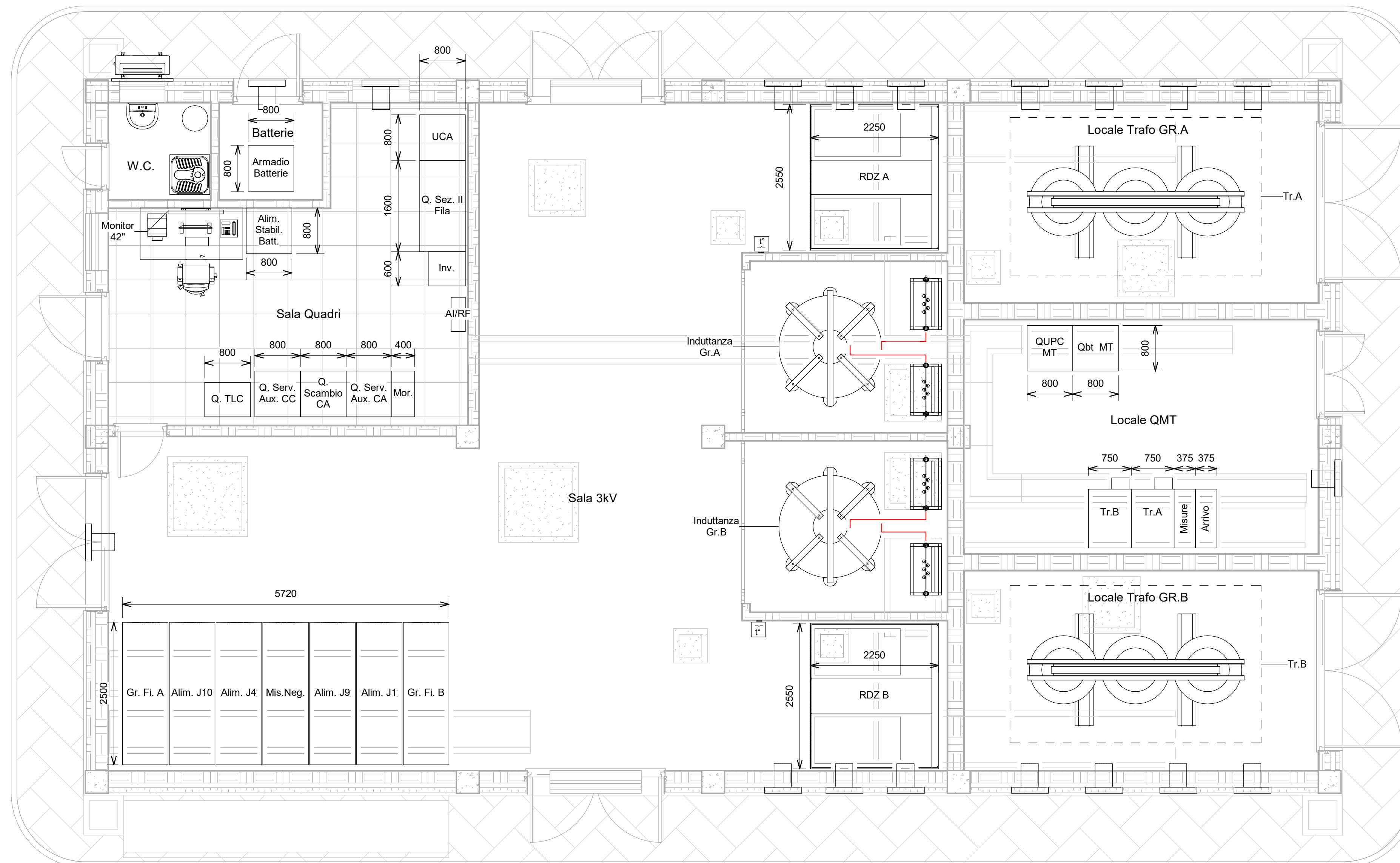
1 Disposizione apparecchiature (Layout) 1 : 50
