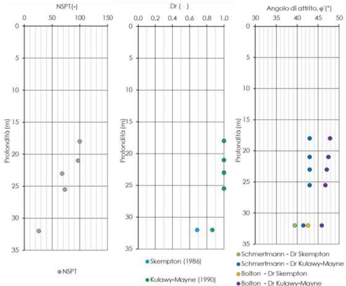
Figura 9-89. NSPT, densità relativa e angolo di attrito da prove SPT
