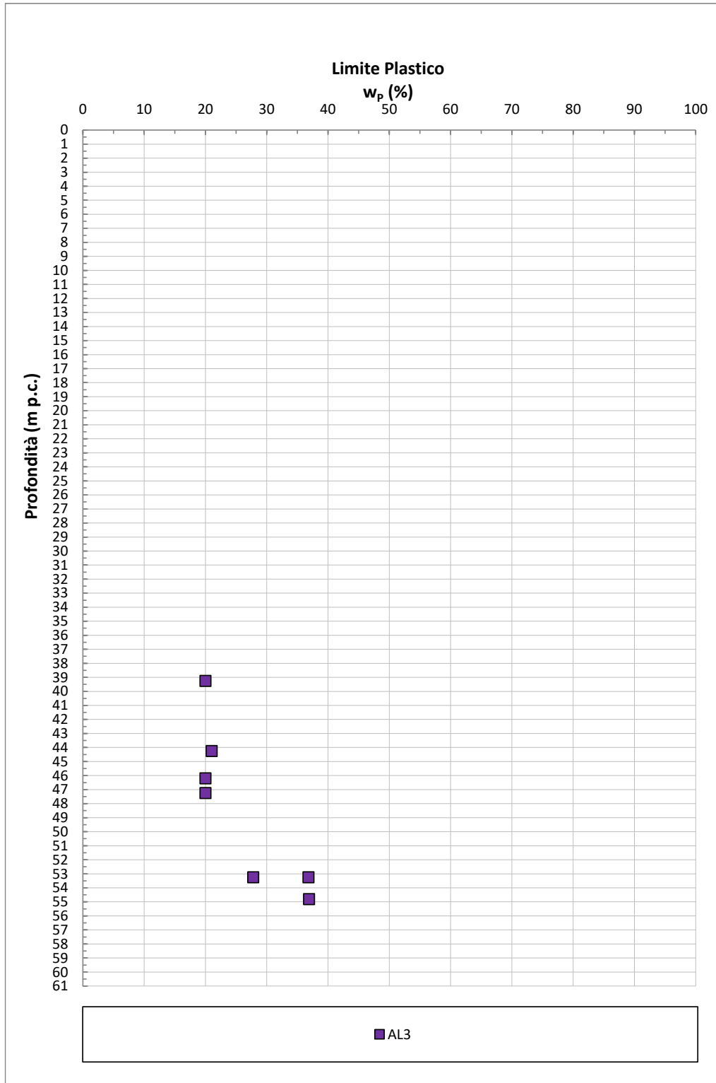
Figura 9-83: AL3 – Limite Plastico
