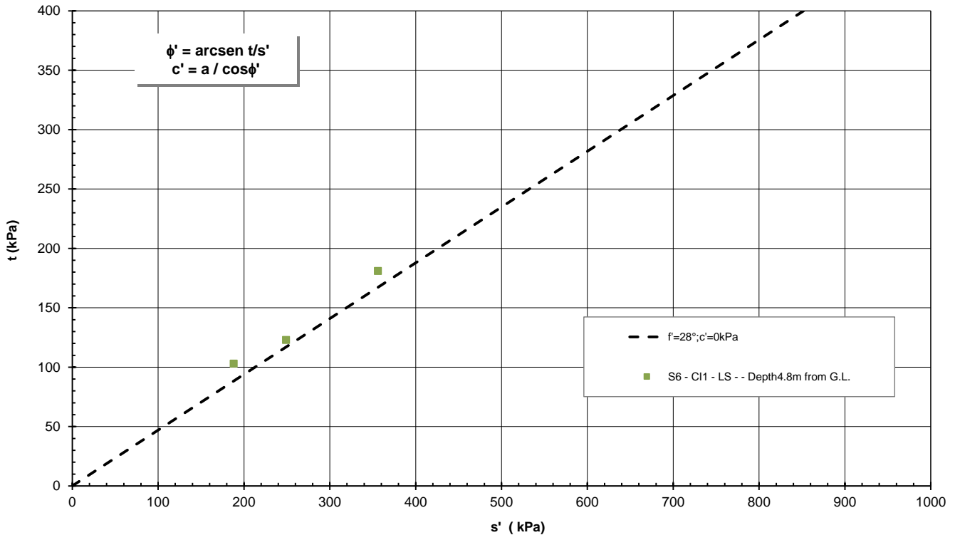
Figura 9-19: LS– Prove di triassiali TX-CIU
