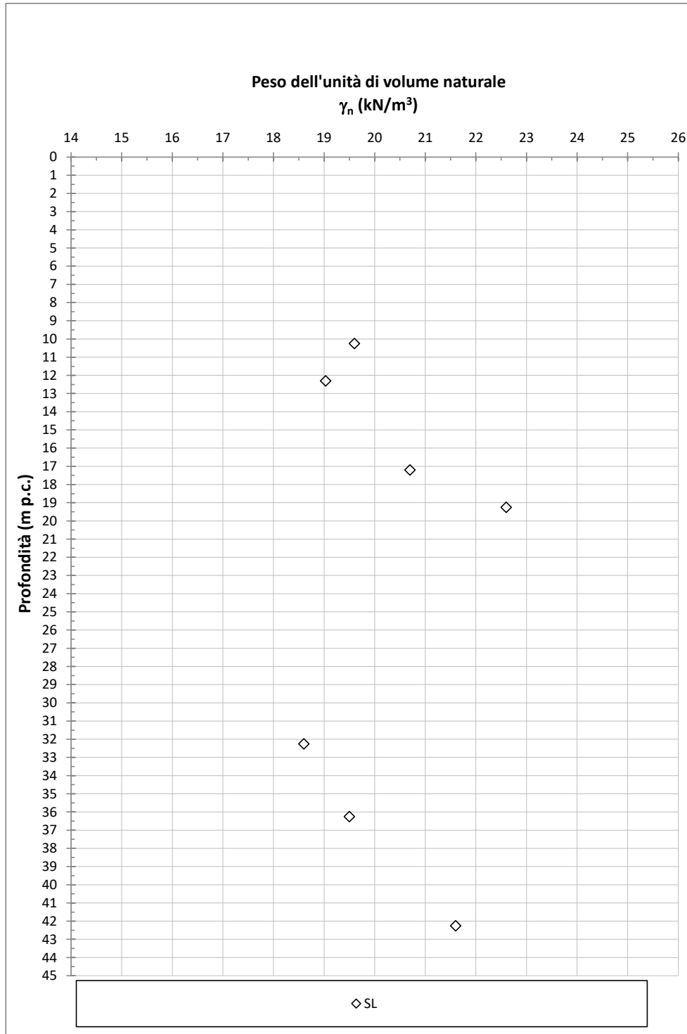
Figura 9-25: SL- Peso dell'unità di volume \gamma_t
