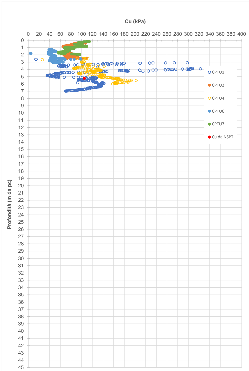
Figura 9-5: R – Coesione non drenata
