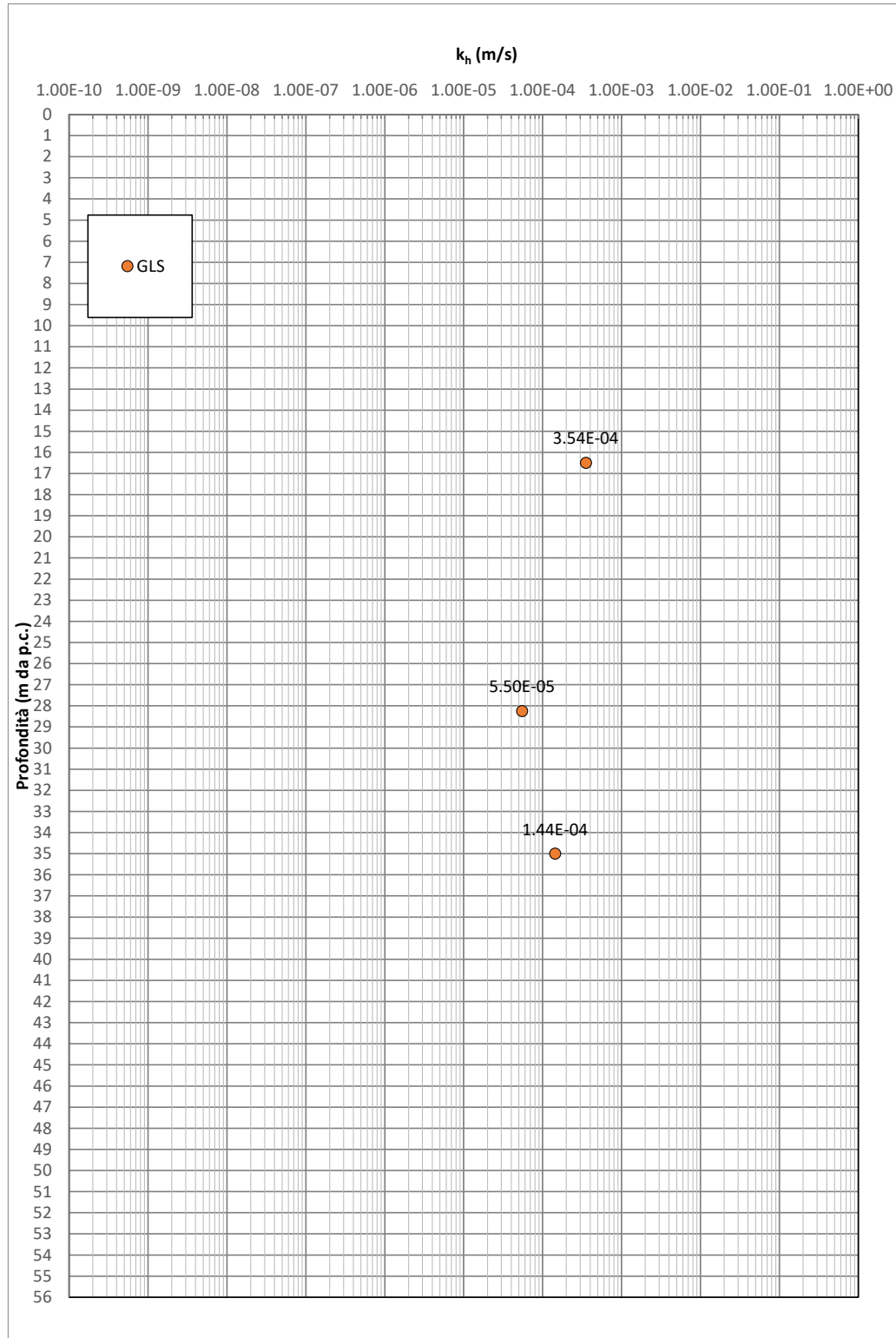
Figura 9-72: GLS – Permeabilità da prove Lefranc
