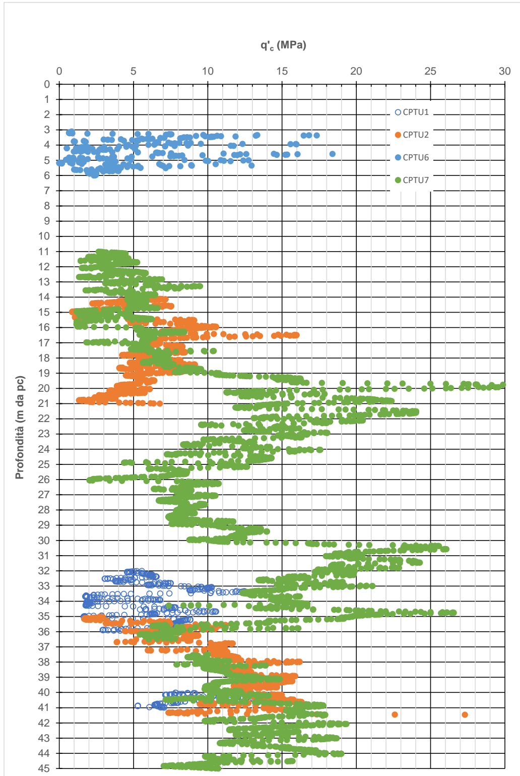
Figura 9-23: SL - q_c
