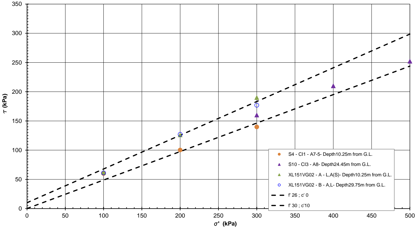
Figura 9-45: AL1 – Prove di taglio diretto TD
