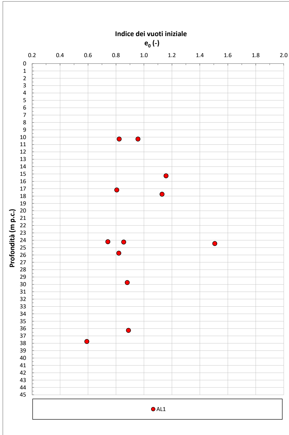
Figura 9-38: AL1 – Indice dei vuoti iniziale e_0
