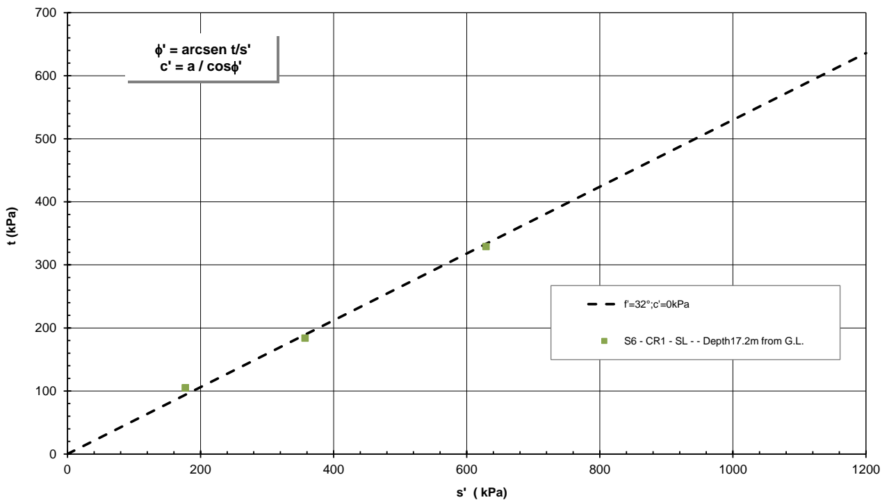
Figura 9-29: SL - Prova triassiale TX-CID
