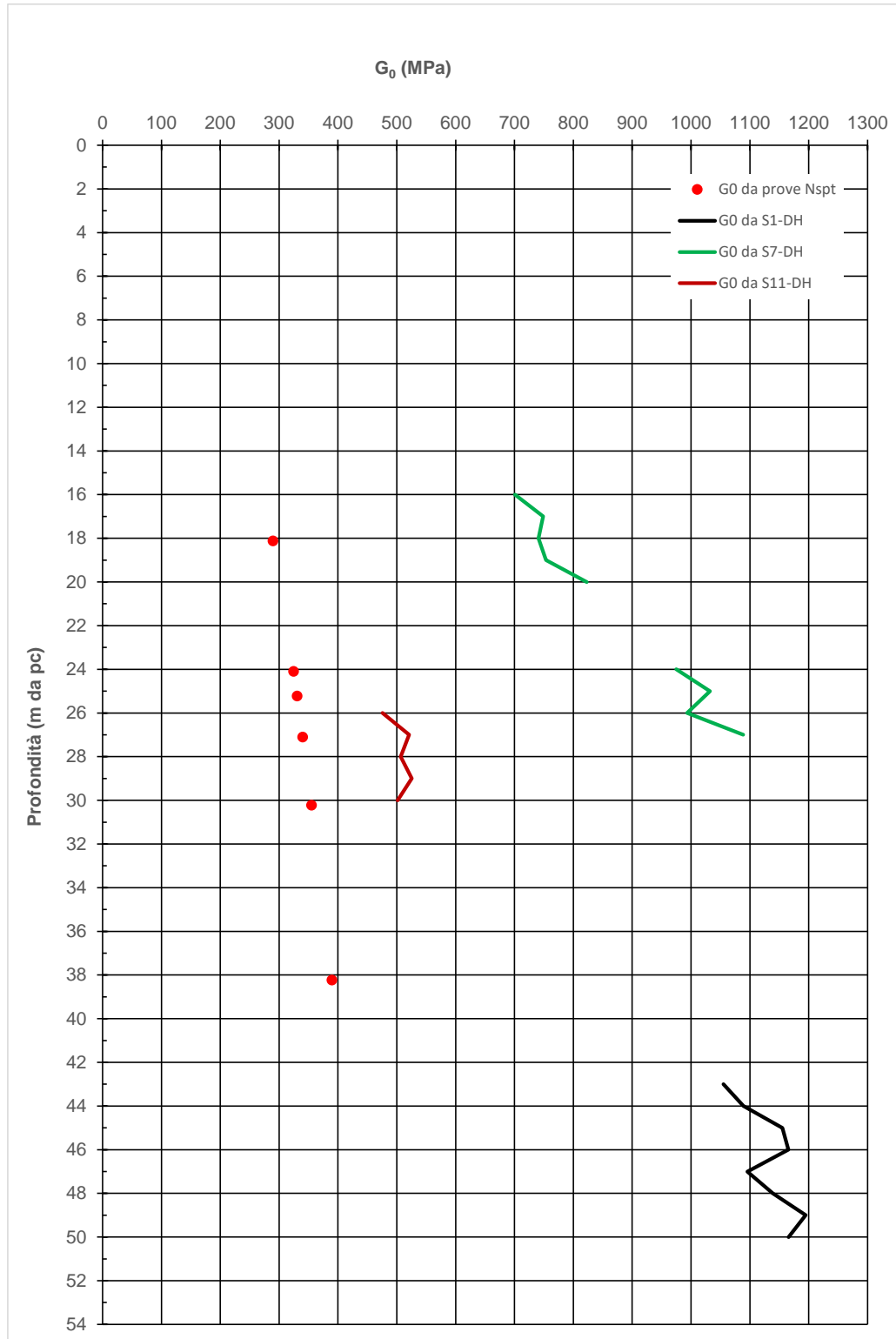
Figura 9-71: GLS - G 0 da prove in sito
