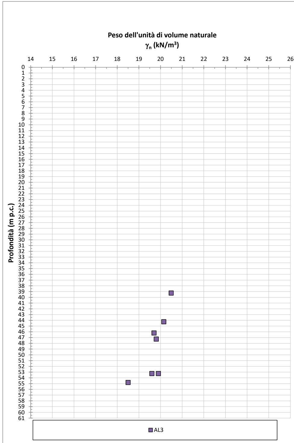
Figura 9-78: AL3 – Peso dell'unità di volume \gamma_t
