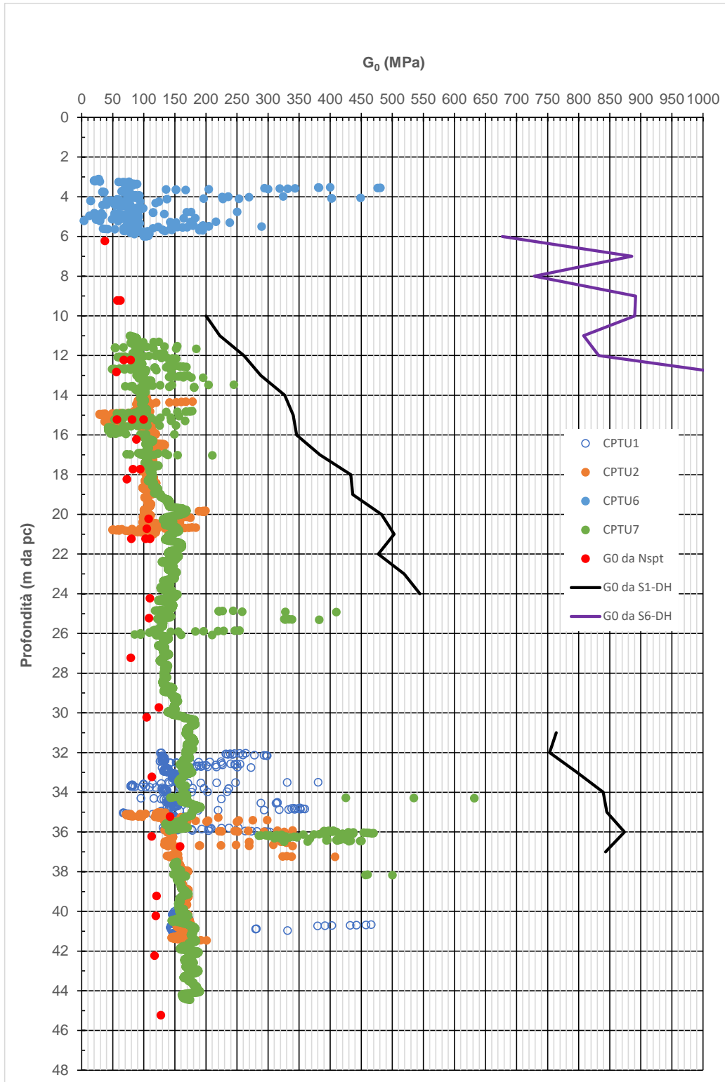
Figura 9-31: SL - G_0 da prove in sito
