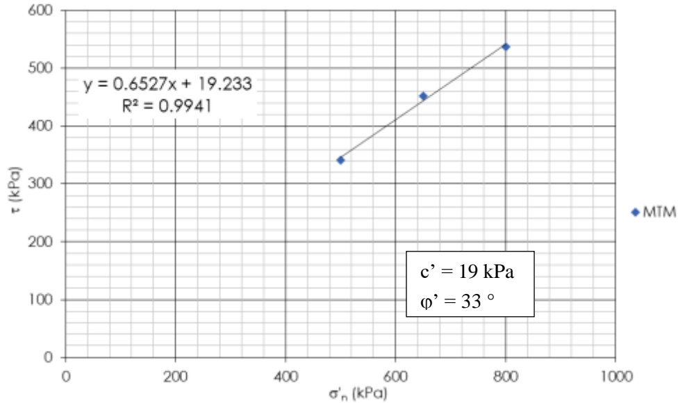
Figura 9-93. Involuppo di resistenza delle prove di taglio diretto
