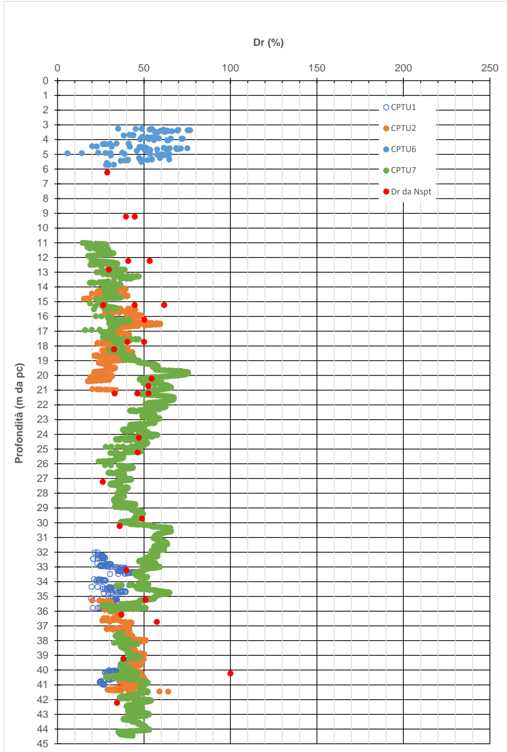
Figura 9-27: SL - Densità relativa da prove in sito
