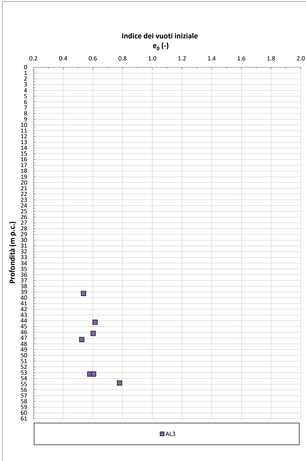
Figura 9-80: AL3 – Indice dei vuoti iniziale e_0
