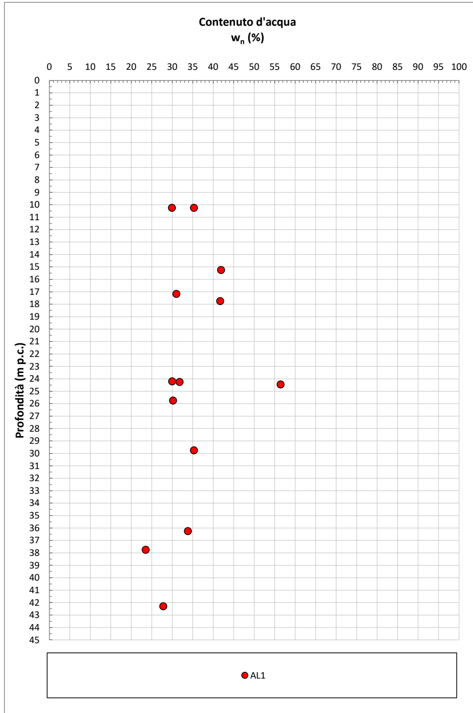
Figura 9-39: AL1 – Contenuto di acqua naturale w_n
