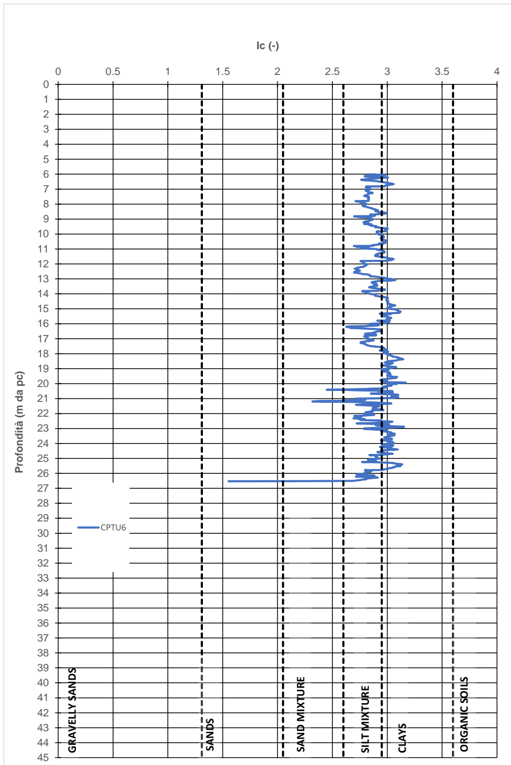
Figura 9-52: AL2 – Indice di comportamento Ic
