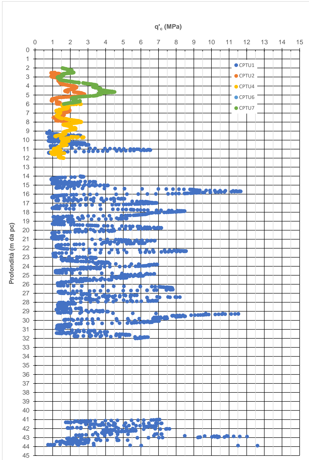
Figura 9-10: LS - q_c
