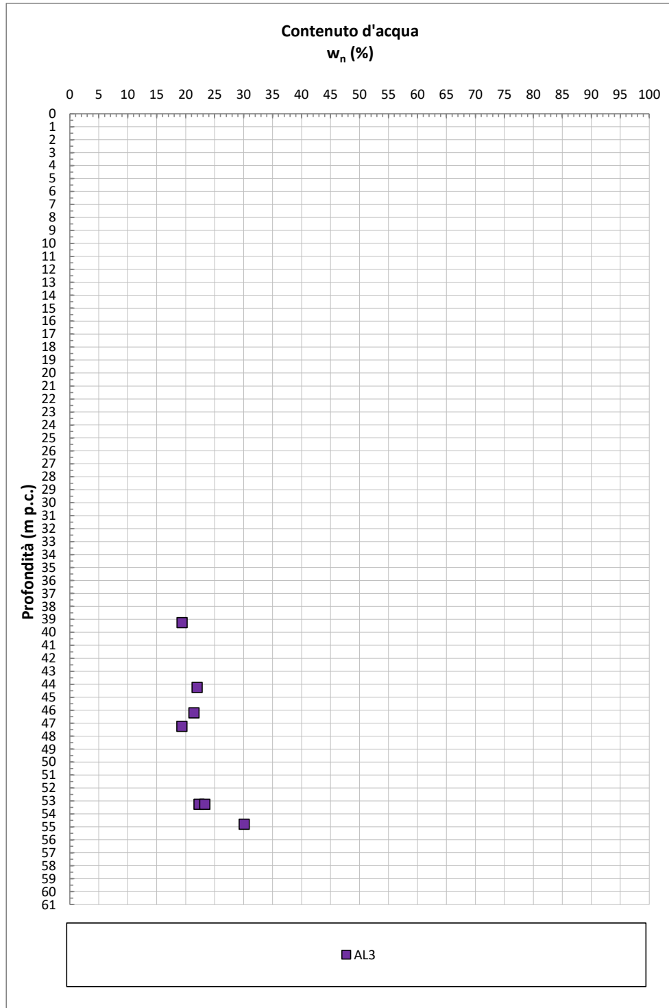
Figura 9-81: AL3 – Contenuto di acqua naturale w_n
