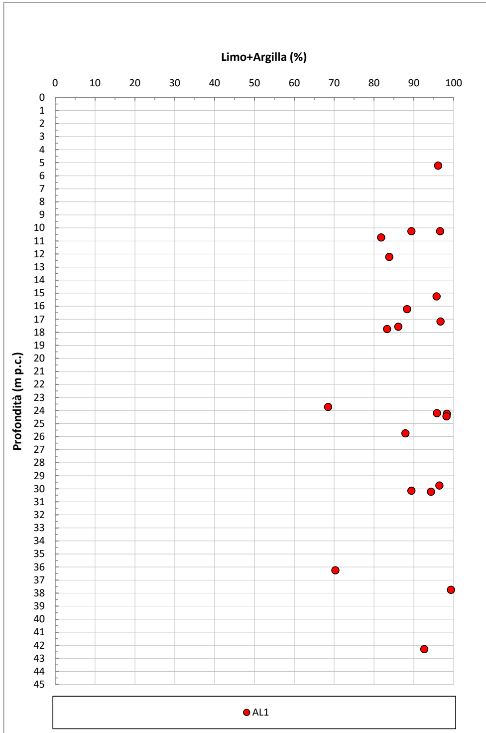
Figura 9-37: AL1 – Contenuto di Limo+Argilla
