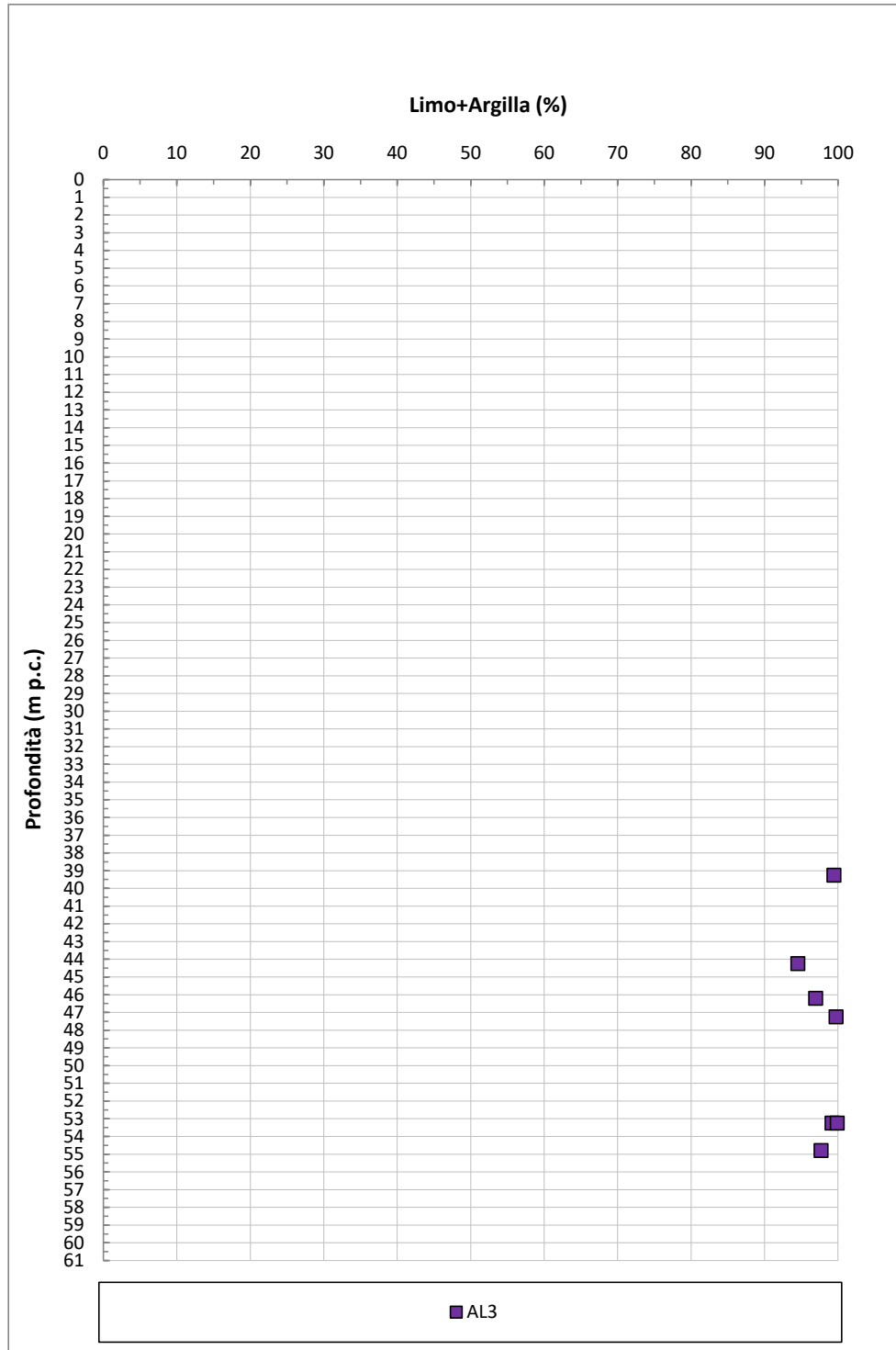
Figura 9-79: AL3 – Contenuto di Limo+Argilla
