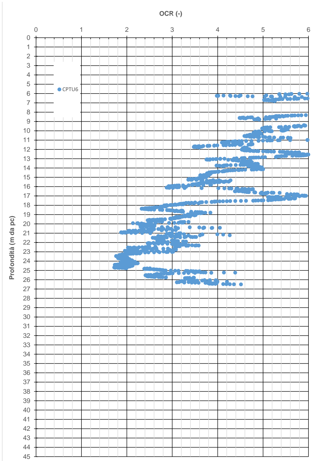
Figura 9-60: AL2 – Grado di sovraconsolidazione da prove CPTu
