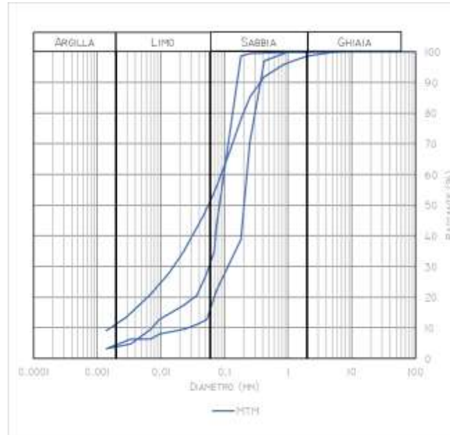
Figura 9-92. Analisi granulometrica
