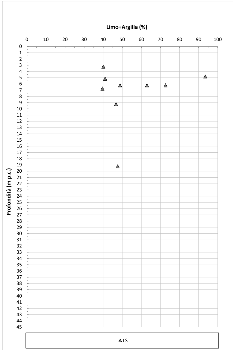
Figura 9-12: Unità LS – Contenuto percentuale di Limo + Argilla
