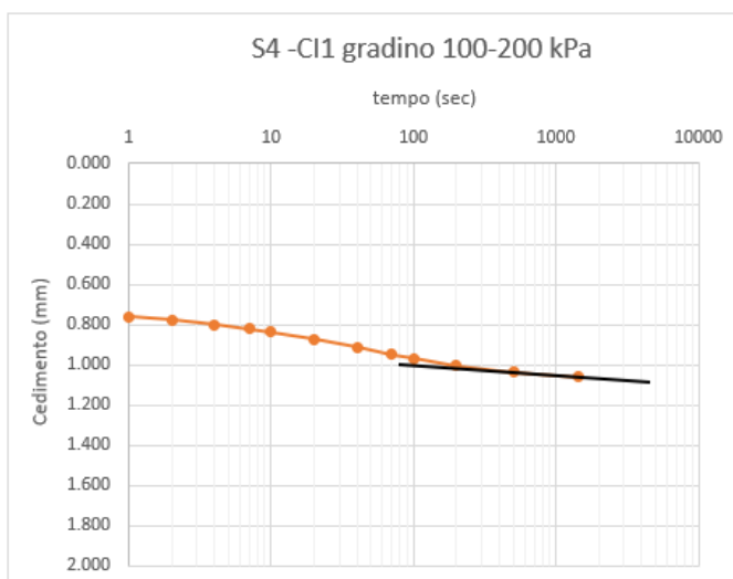
Figura 8-1: - Esempio di calcolo del coefficiente di consolidazione secondaria C_{\alpha\varepsilon} . Il coefficiente è rappresentato dalla pendenza della retta nera.
