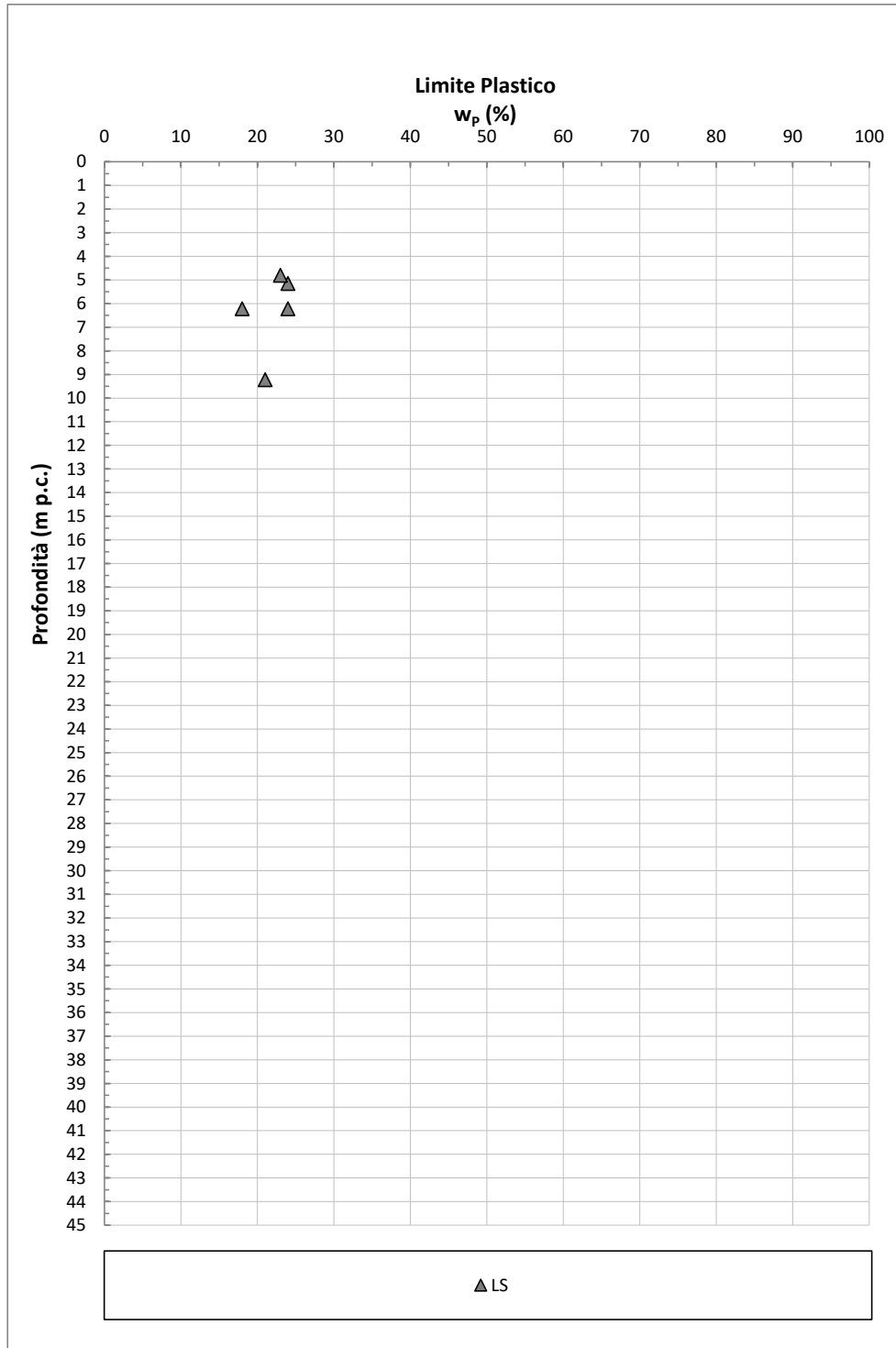
Figura 9-14: LS – Limite Plastico
