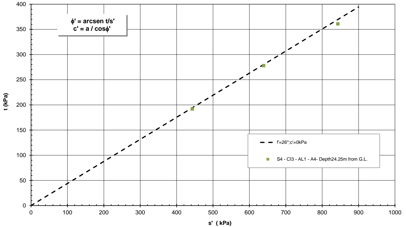
Figura 9-46: AL1 – Prove triassiali TX-CIU
