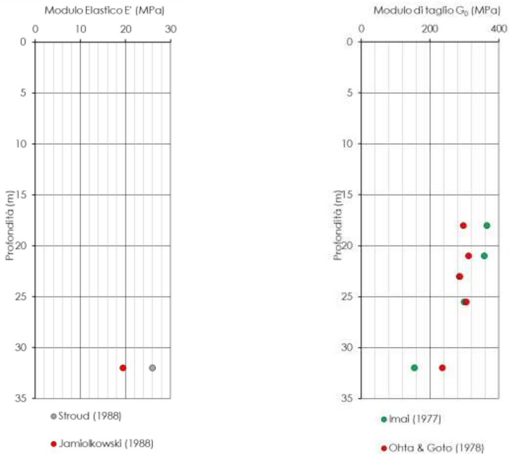
Figura 9-90. Modulo elastico E' e modulo di taglio G_0 da prove SPT
