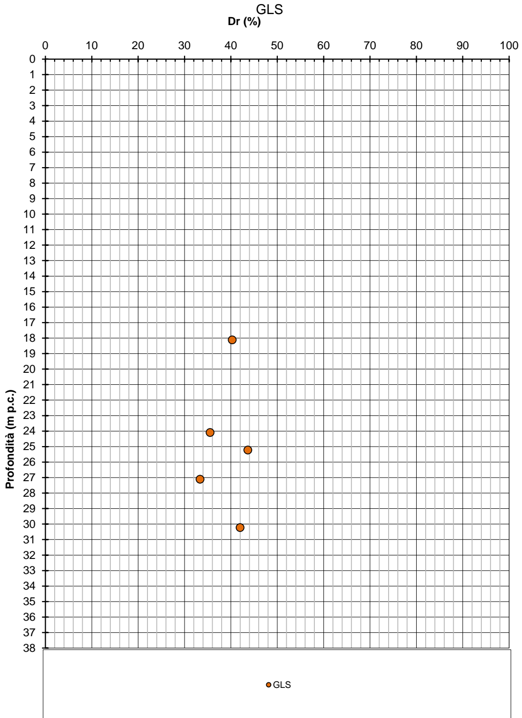
Figura 9-69: GLS - Densità relativa da prove in sito N_{SPT}
