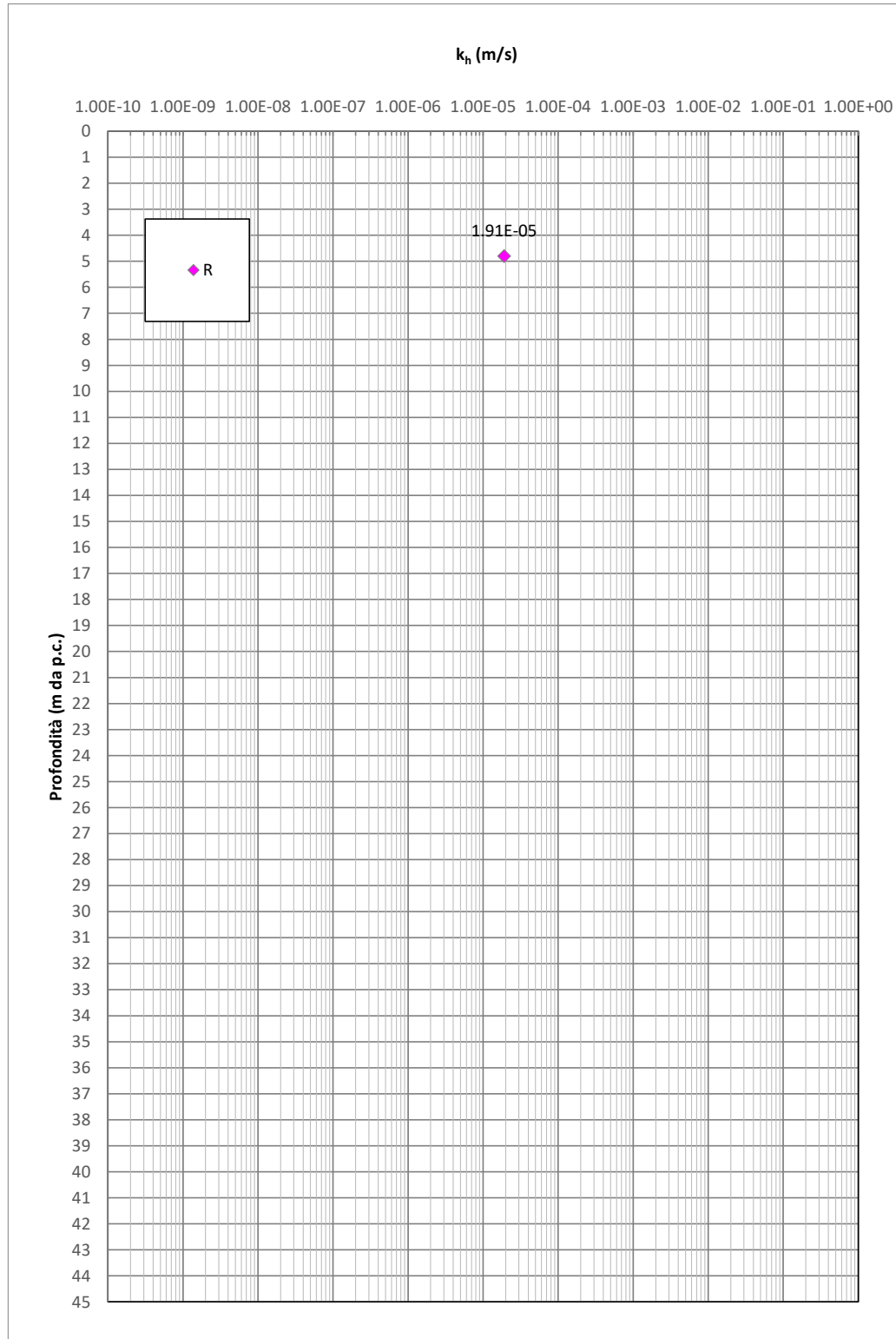
Figura 9-8: R – Permeabilità da prove Lefranc
