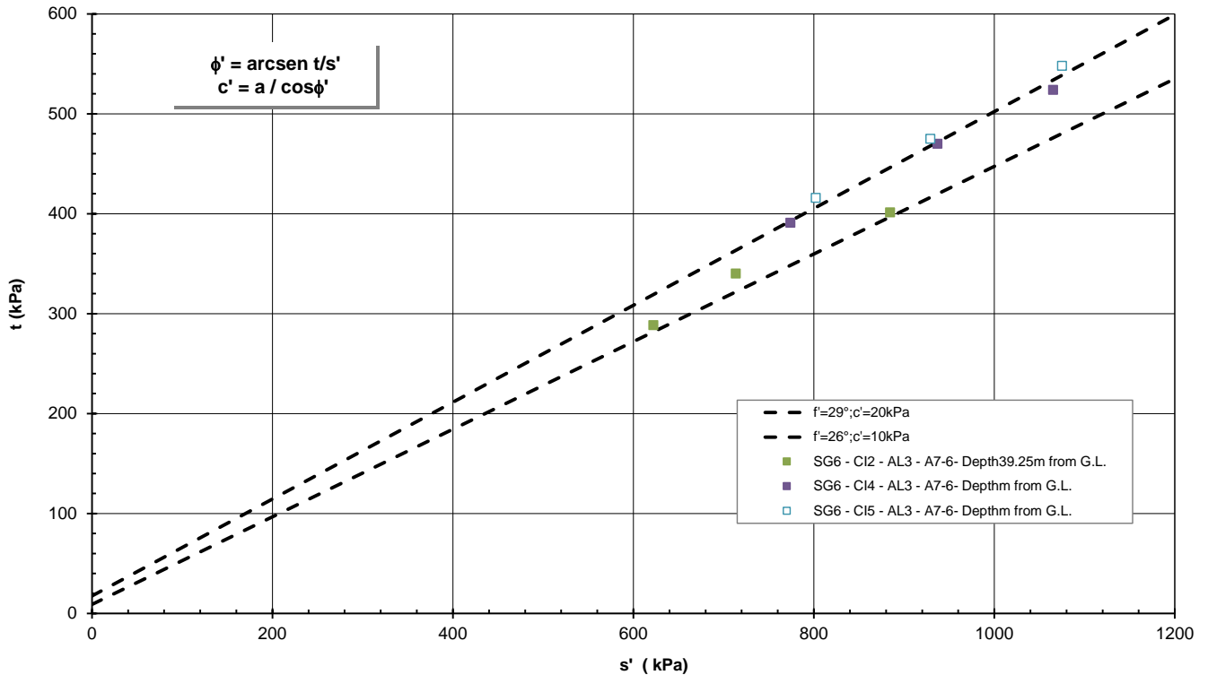
Figura 9-86: AL3 – Prove di taglio diretto TD
