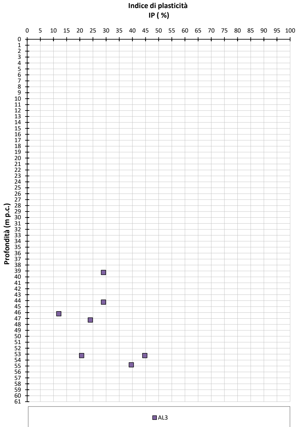
Figura 9-84: AL3 - Indice di plasticità PI
