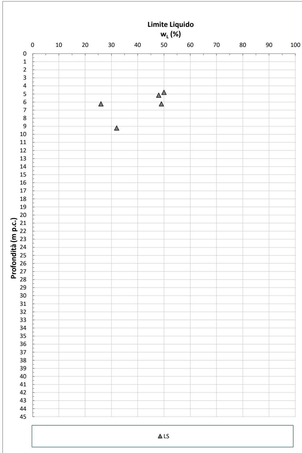
Figura 9-13: LS – Limite Liquido
