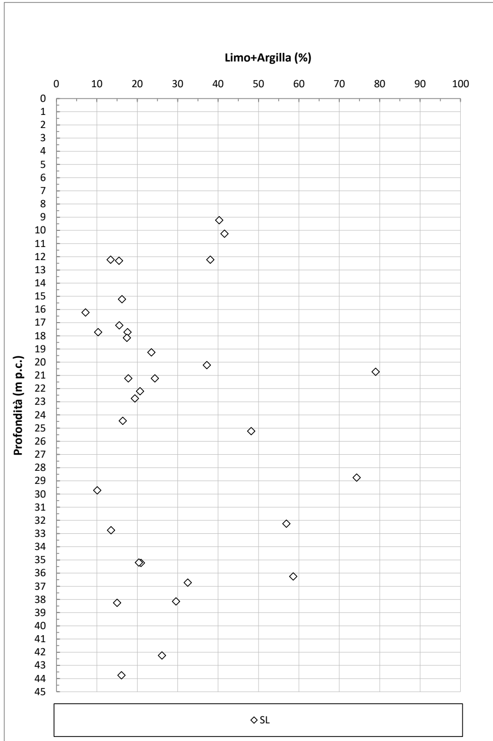
Figura 9-26 – SL - Contenuto percentuale di Limo+Argilla
