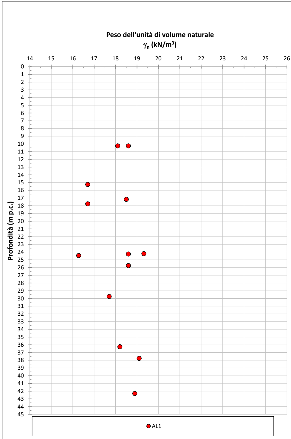
Figura 9-36: AL1 – Peso dell'unità di volume \gamma_t
