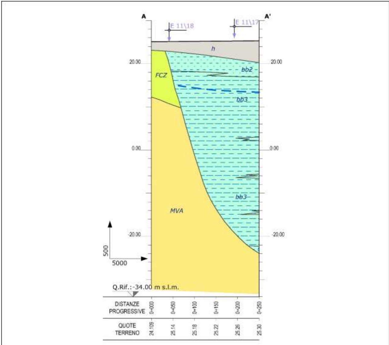
Figura 11-5: sezione geologica e geotecnica dell'area dei fabbricati tecnologici di progetto in zona Vigna Clara
