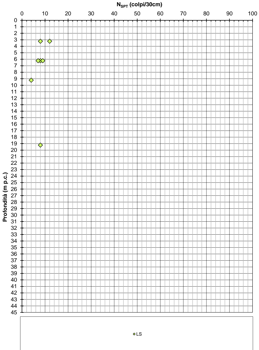
Figura 9-9: LS - N SPT
