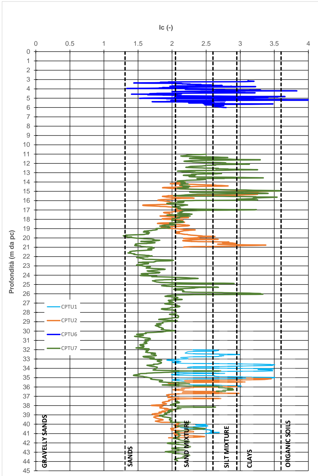
Figura 9-24: SL – Indice di comportamento Ic
