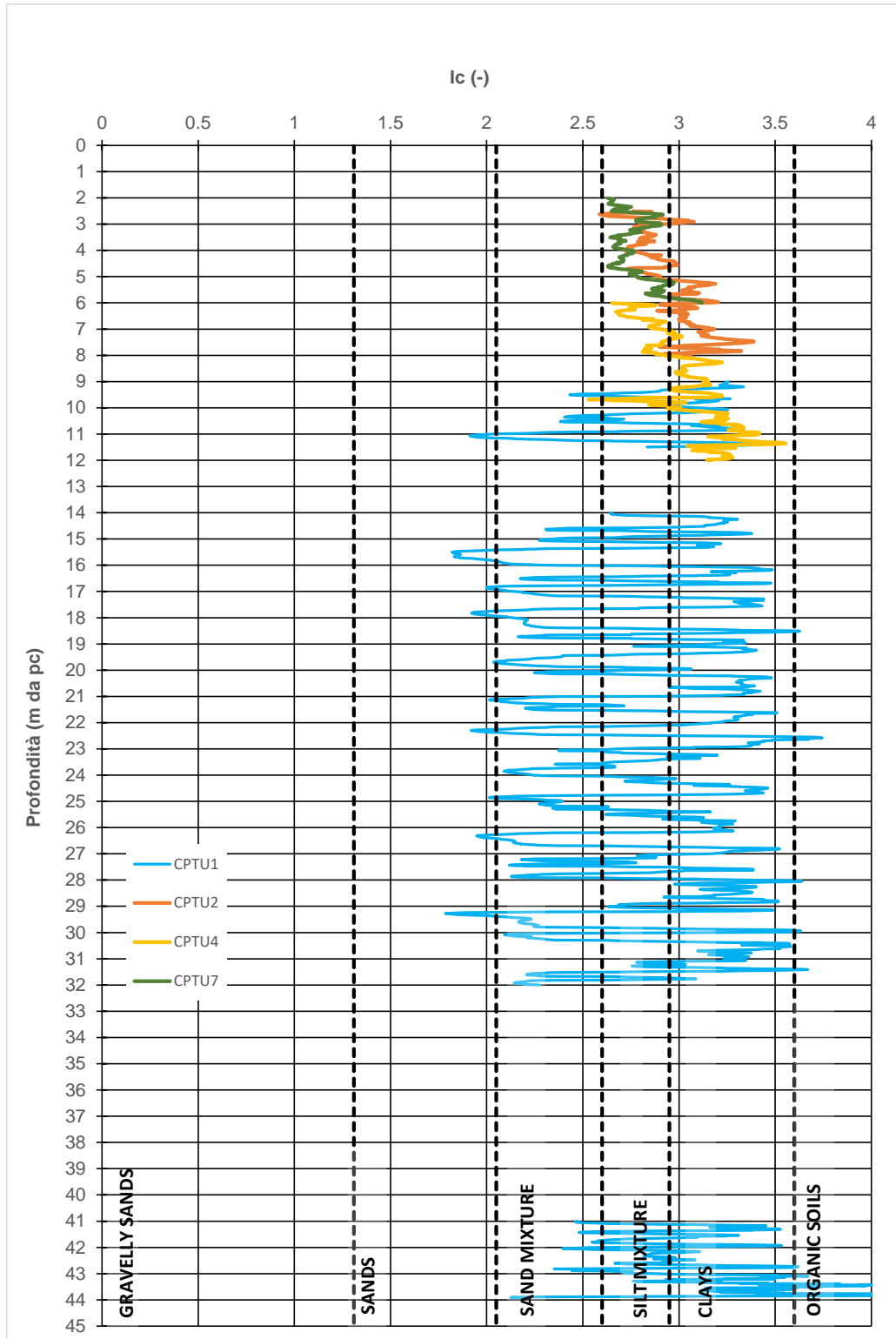
Figura 9-11: LS – Indice di comportamento Ic
