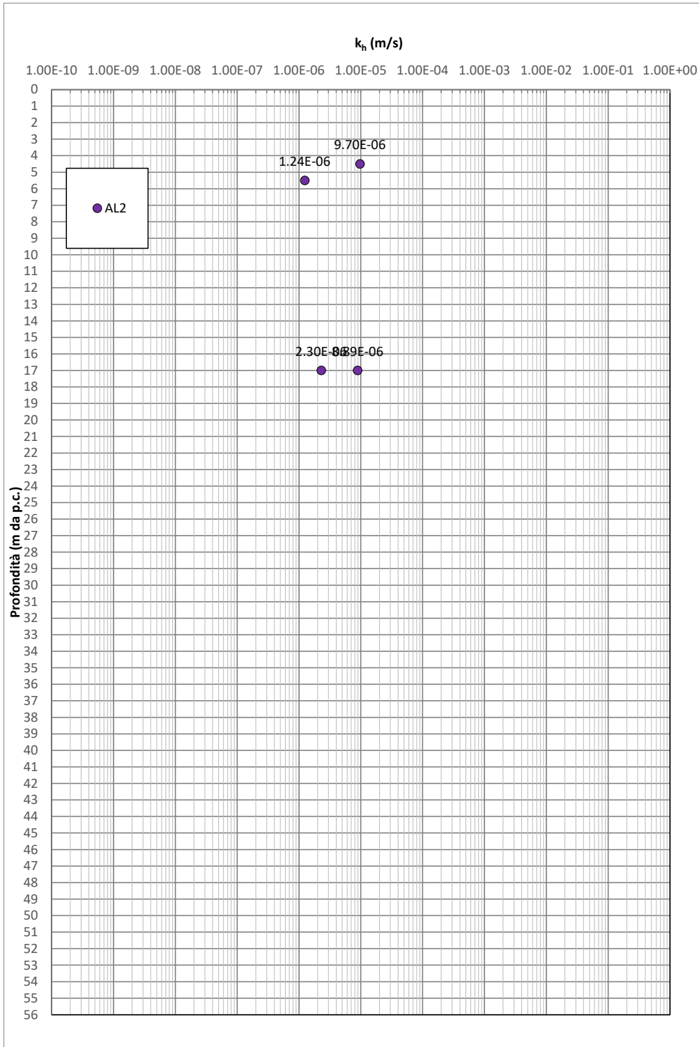
Figura 9-65: AL2 – Permeabilità da prove Lefranc
