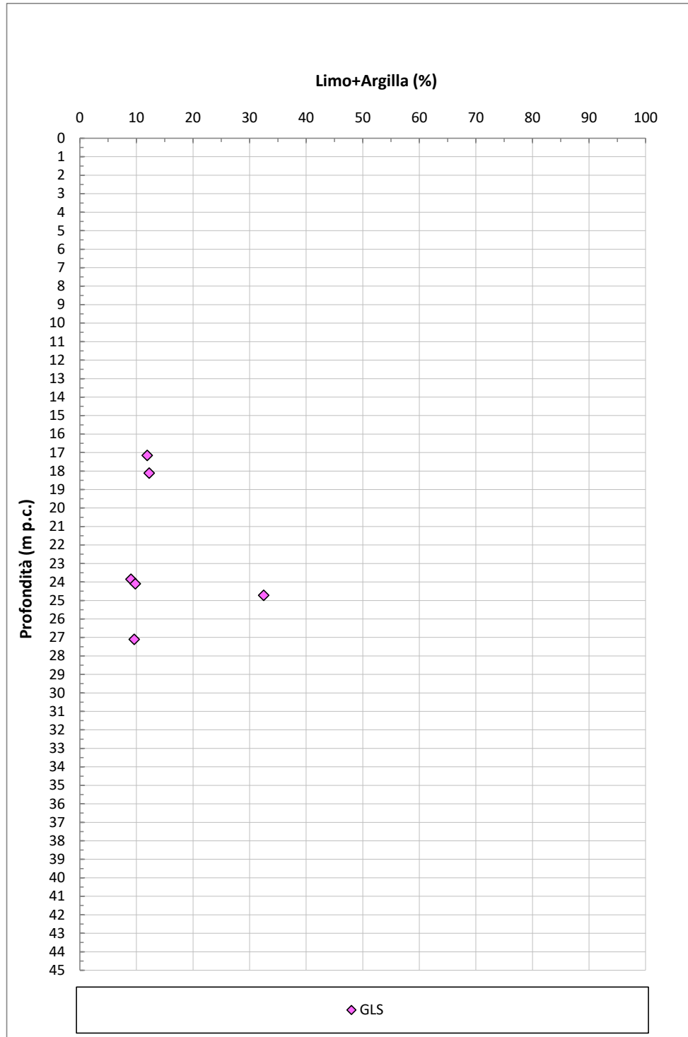
Figura 9-68: GLS - Contenuto di Limo+Argilla
