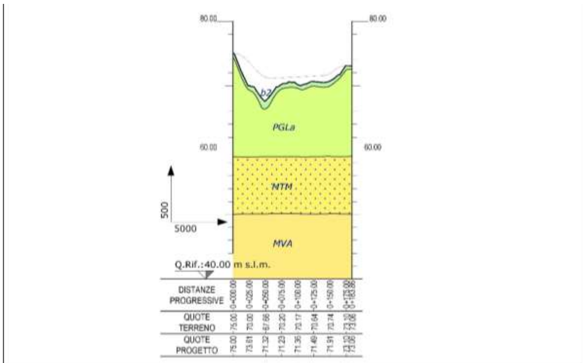
Figura 11-2: sezione geologica e geotecnica in corrispondenza di NV03
