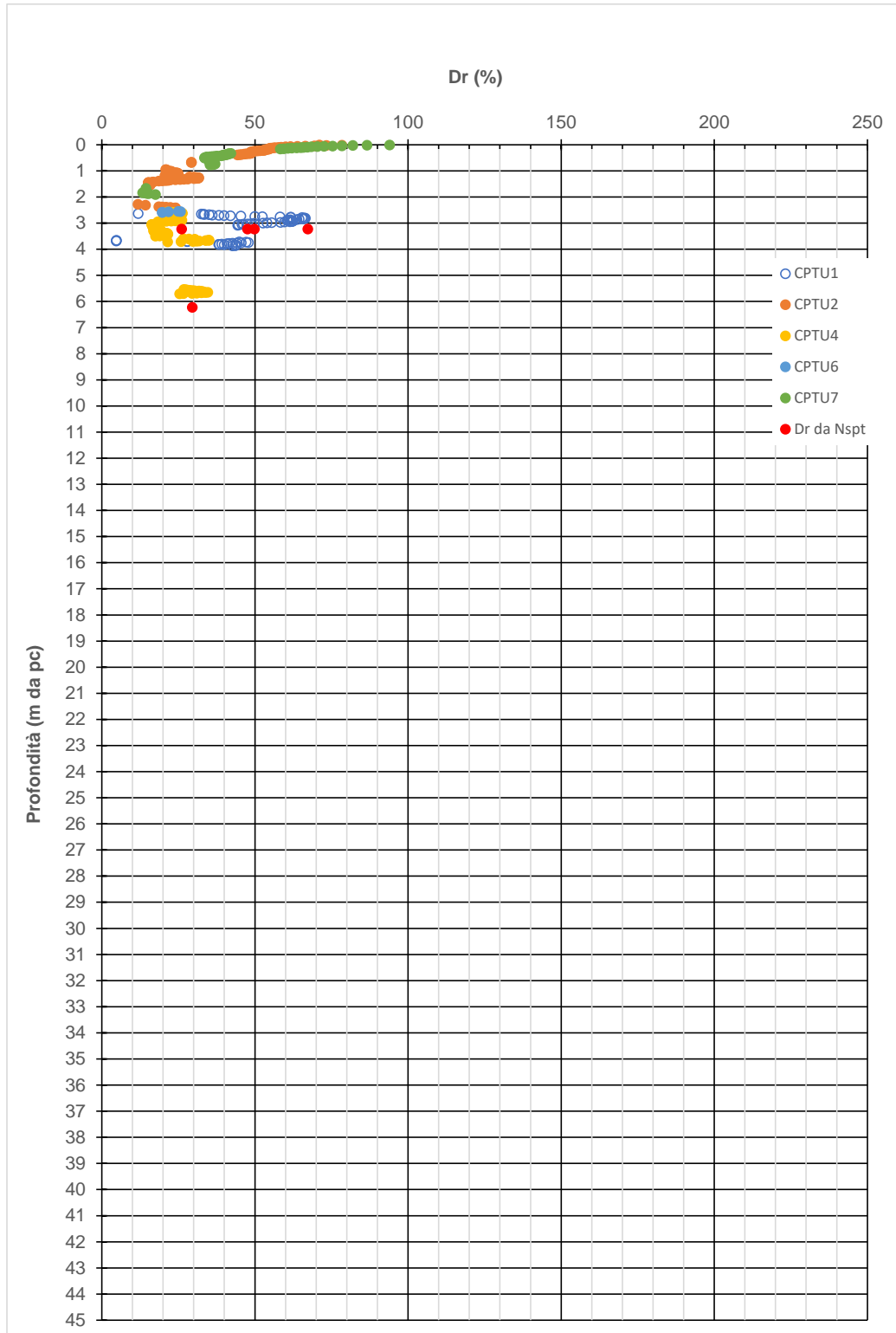
Figura 9-4: R - Densità relativa
