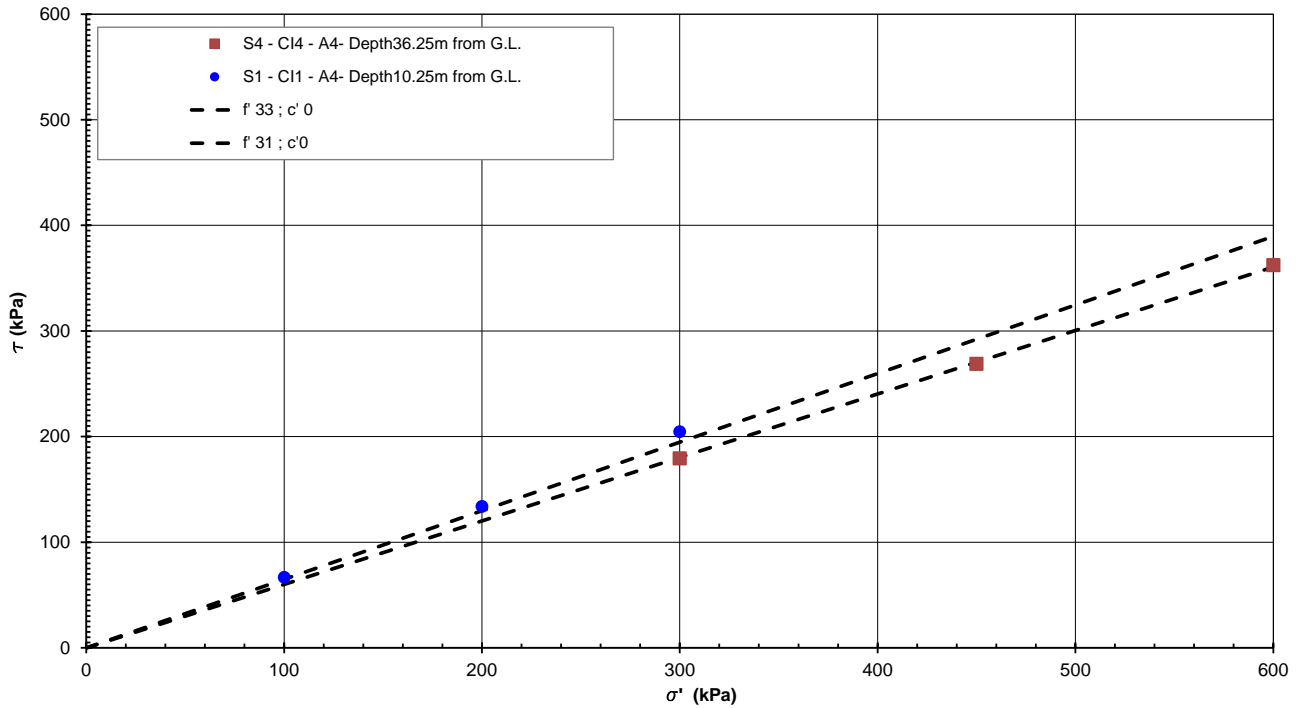
Figura 9-28: SL - Prove di taglio diretto
