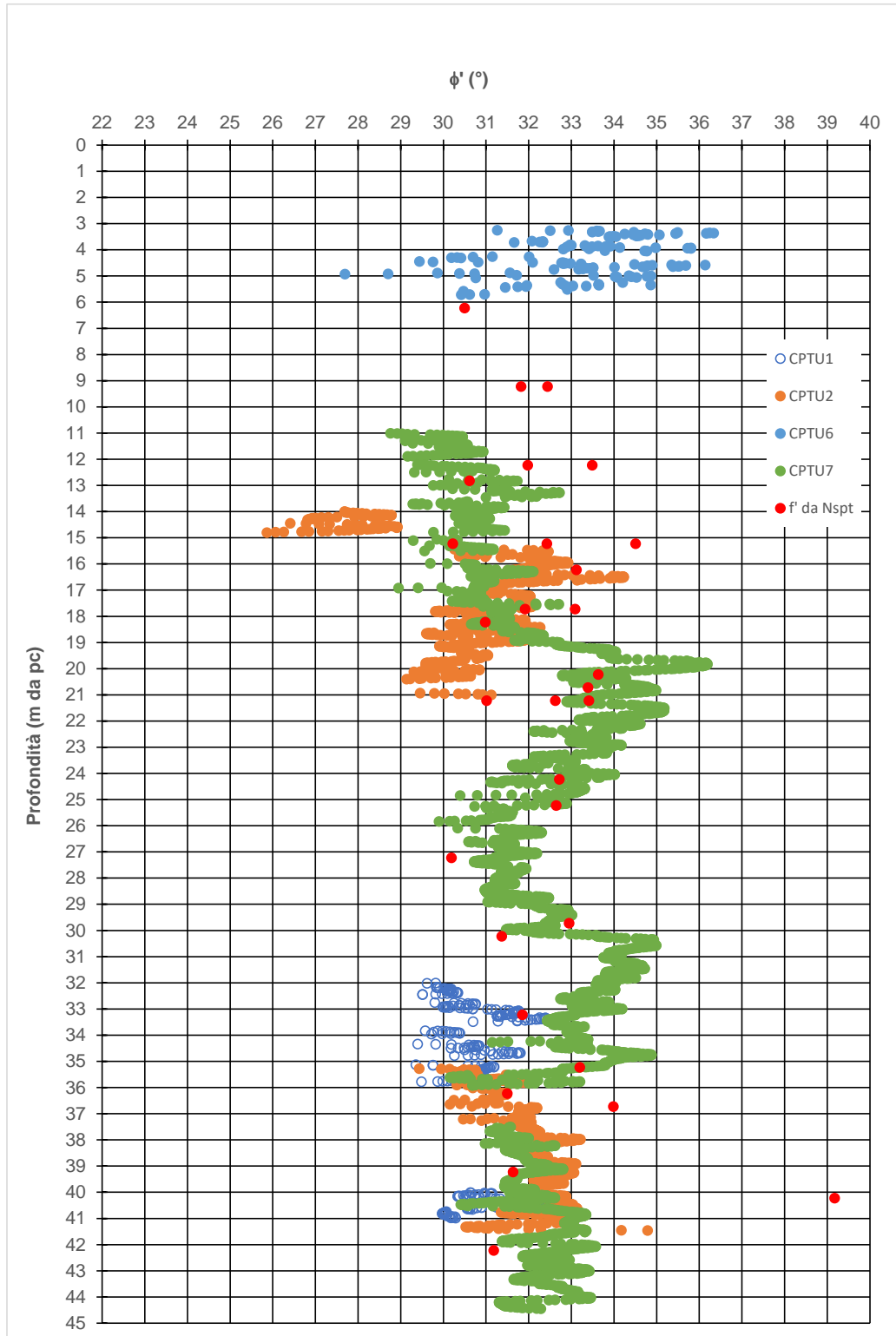
Figura 9-30: SL - Angolo d'attrito da prove in sito
