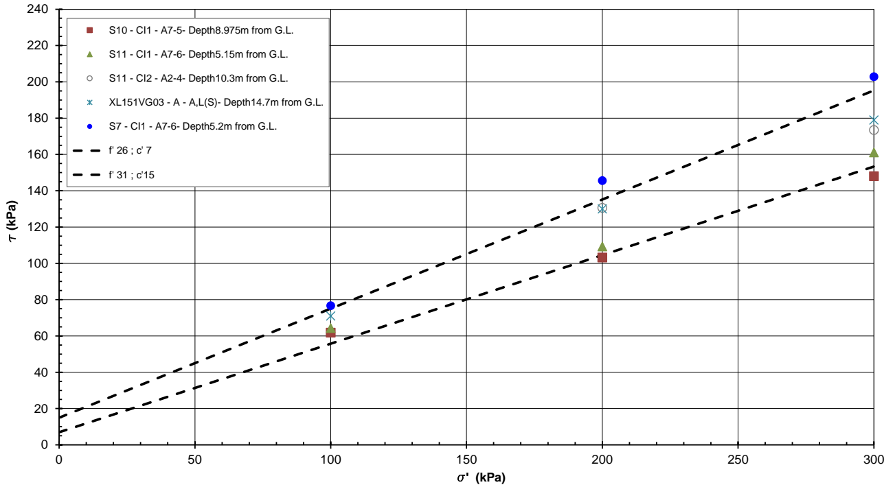
Figura 9-62: AL2 – Prove di taglio diretto TD
