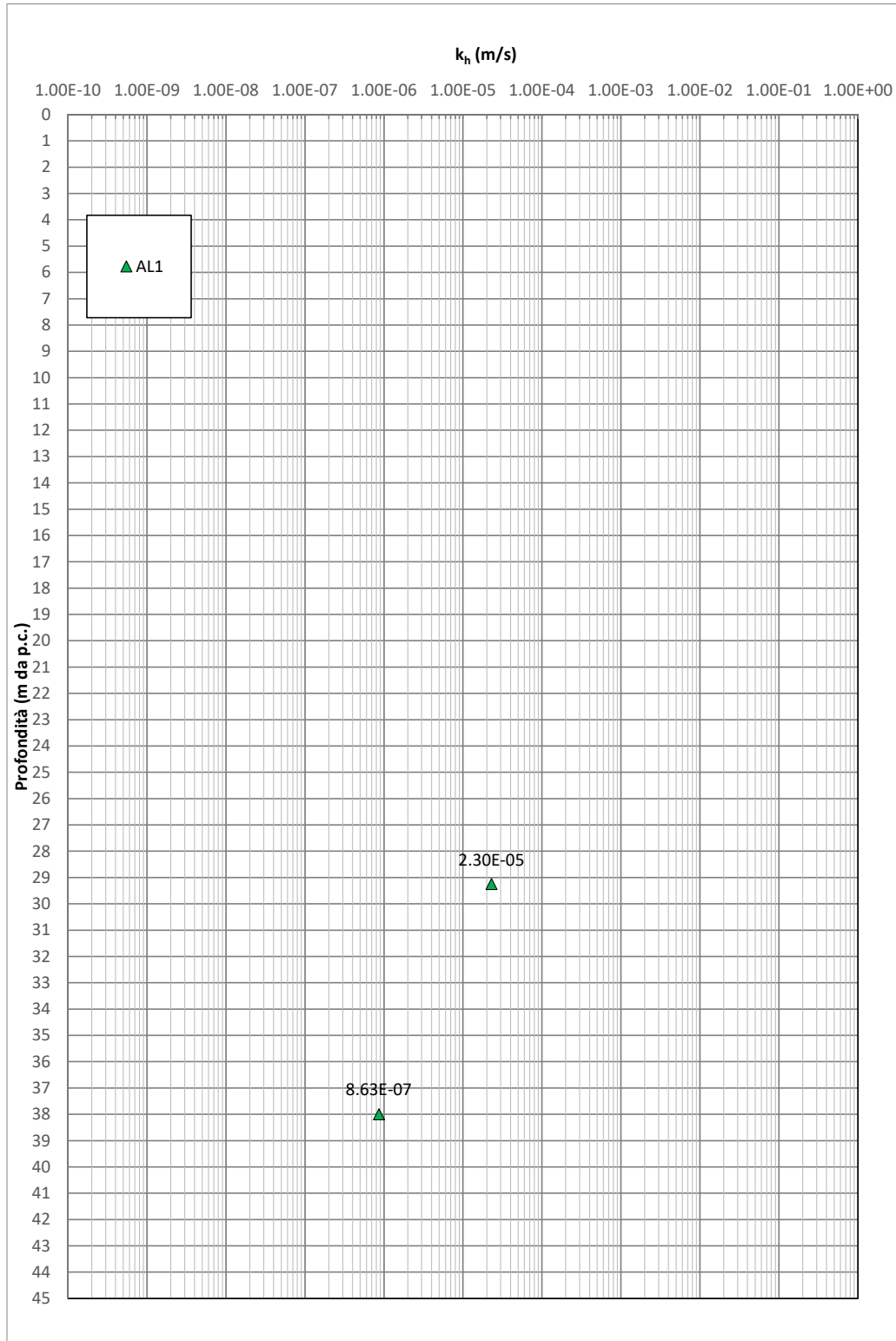
Figura 9-49: AL1– Permeabilità da prove Lefranc
