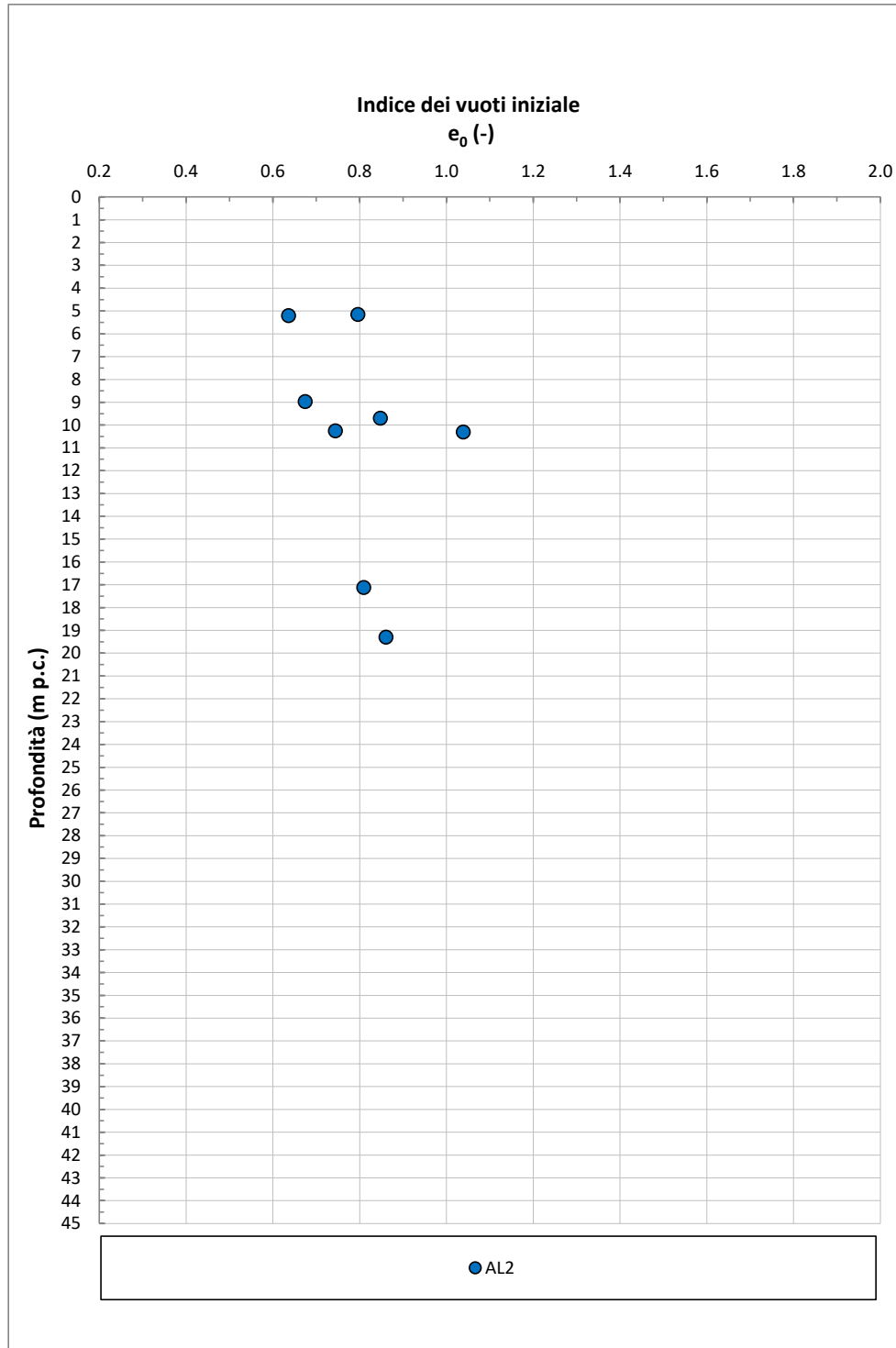
Figura 9-55: AL2 – Indice dei vuoti iniziale e_0
