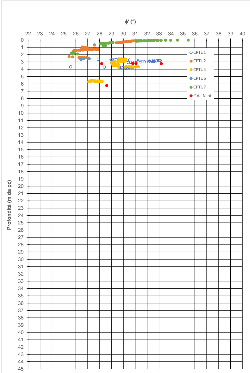
Figura 9-6: R - Angolo d'attrito
