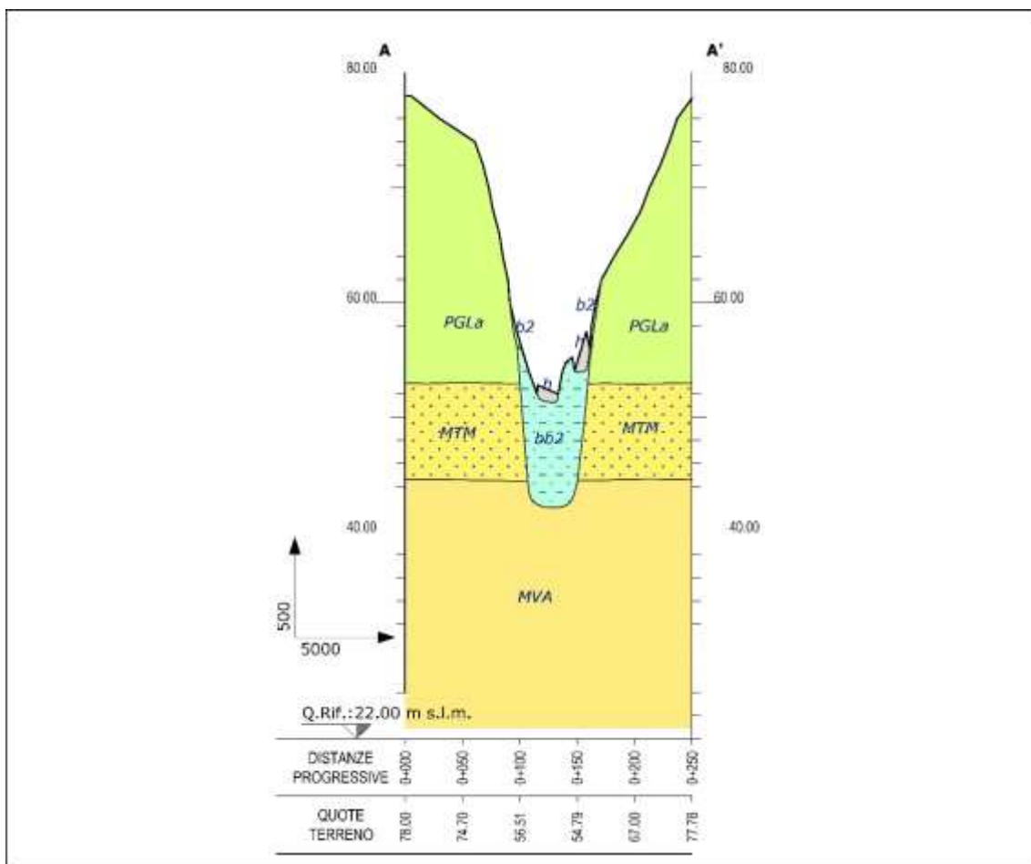
Figura 11-4: sezione geologia e geotecnica dell'area interessata dalla paratia
