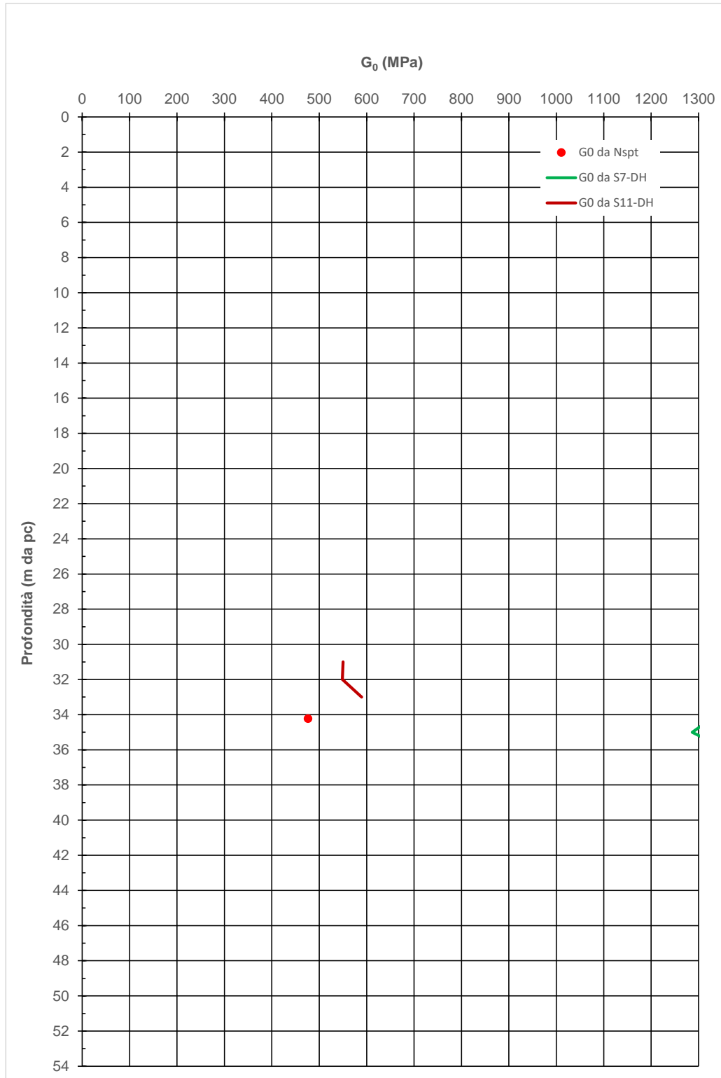
Figura 9-77: GSL - G_0 da prove in sito
