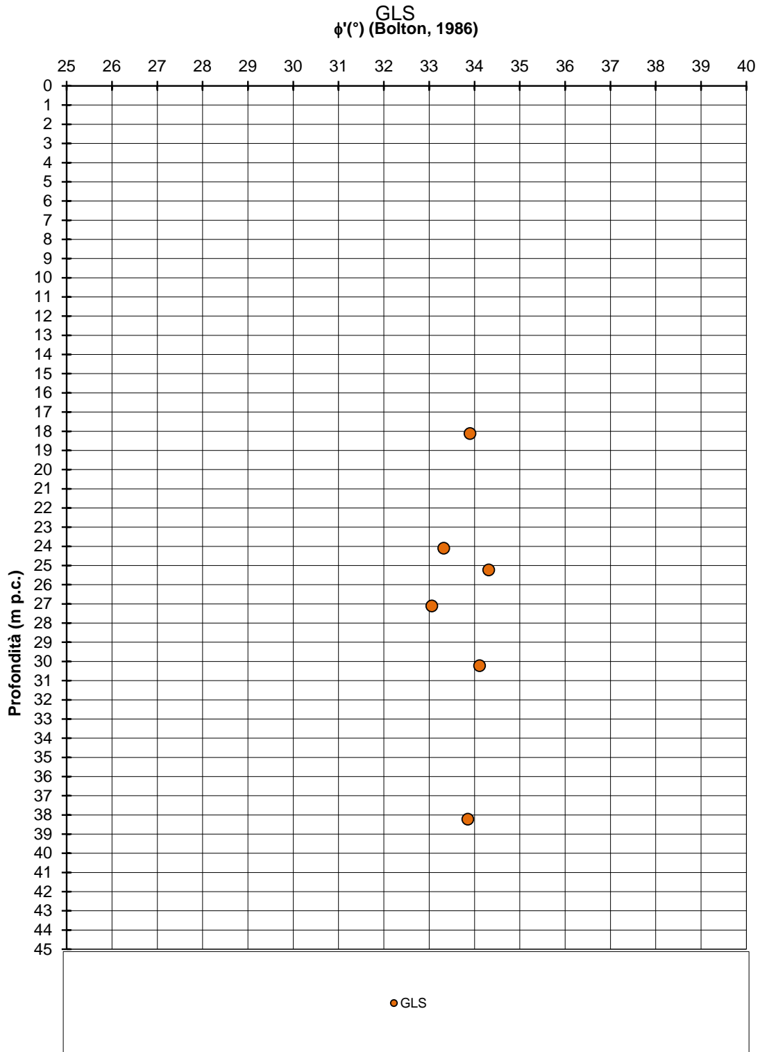
Figura 9-70: GLS - Angolo d'attrito da prove in sito N_{SPT}
