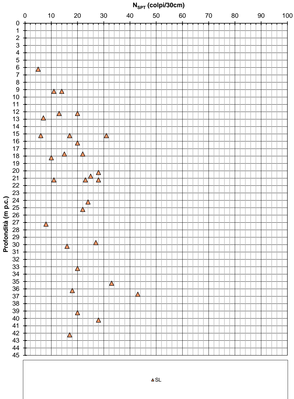
Figura 9-22: SL - N_{SPT}
