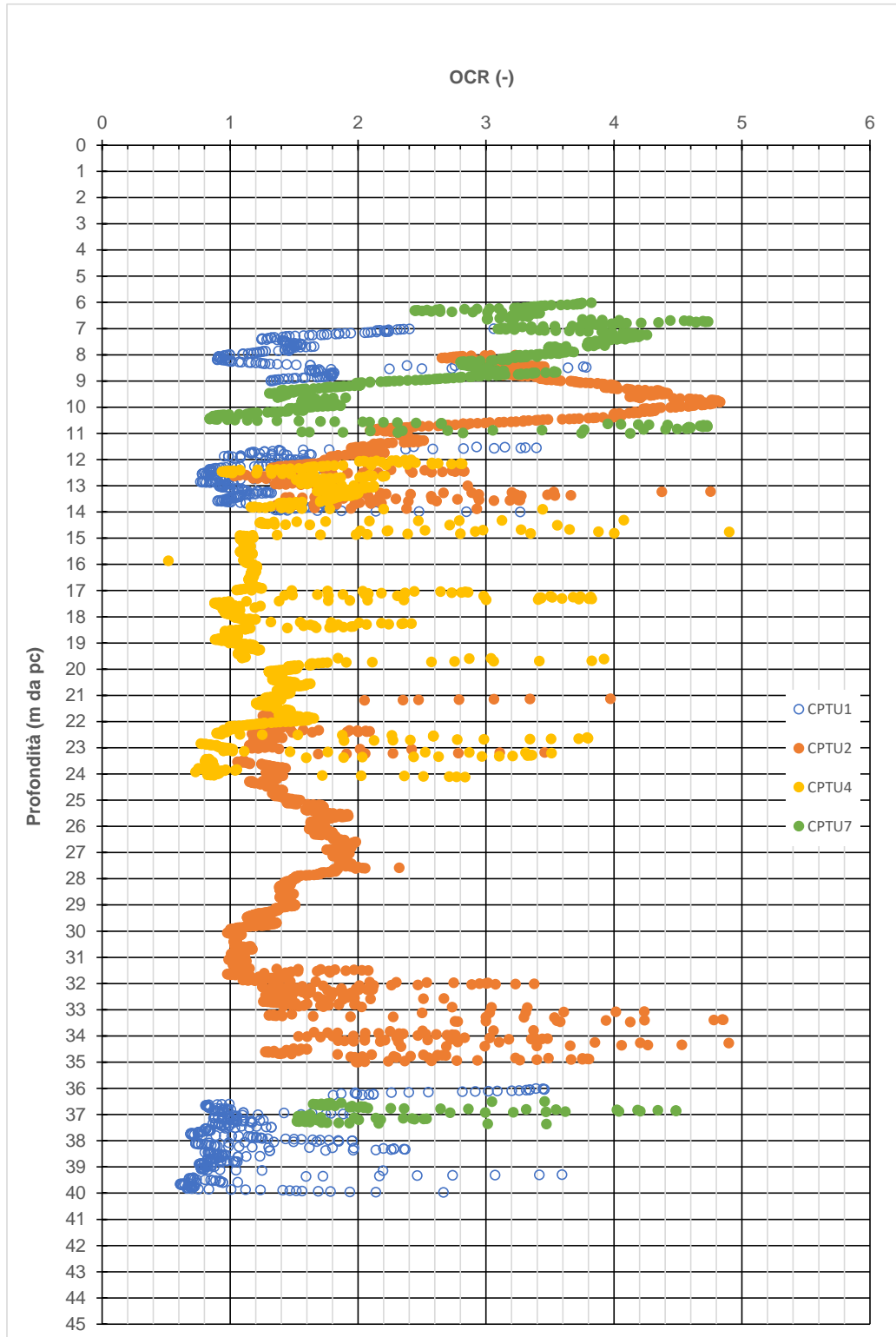
Figura 9-43: AL1 – Grado di sovraconsolidazione da prove CPTu
