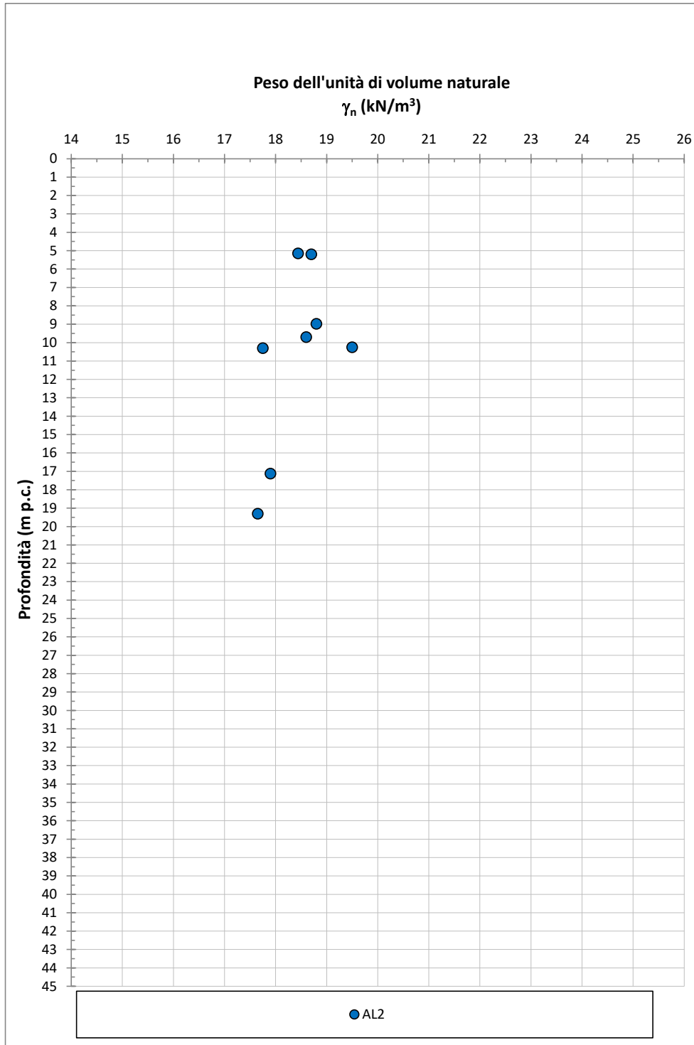
Figura 9-53: AL2 – Peso dell'unità di volume \gamma_t
