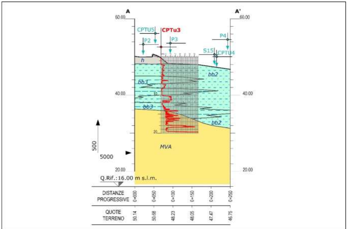
Figura 11-3: sezione geologica e geotecnica relativa alla zona dei fabbricati tecnologici di progetto in zona Pineto
