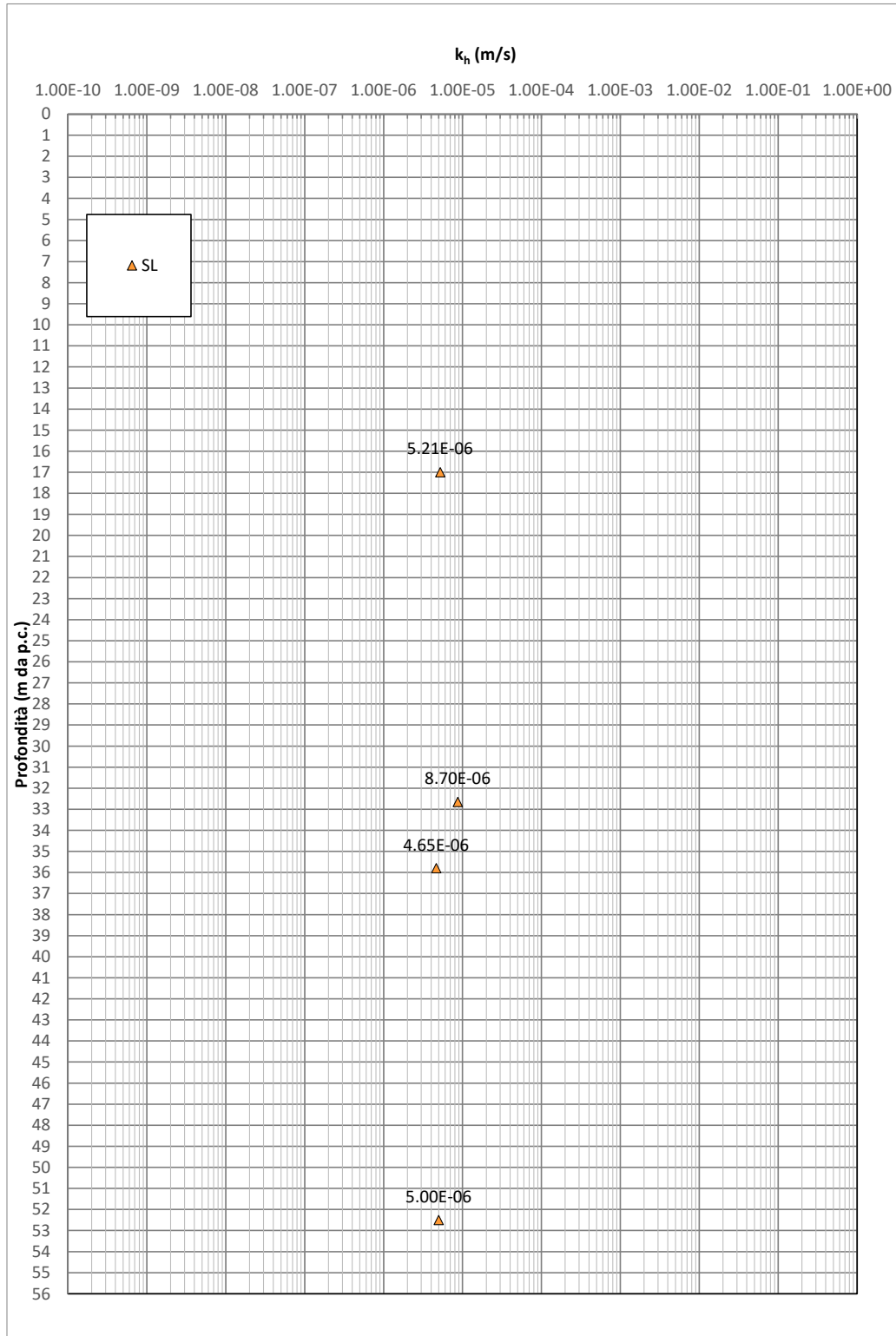
Figura 9-32: SL – Permeabilità da prove Lefranc
