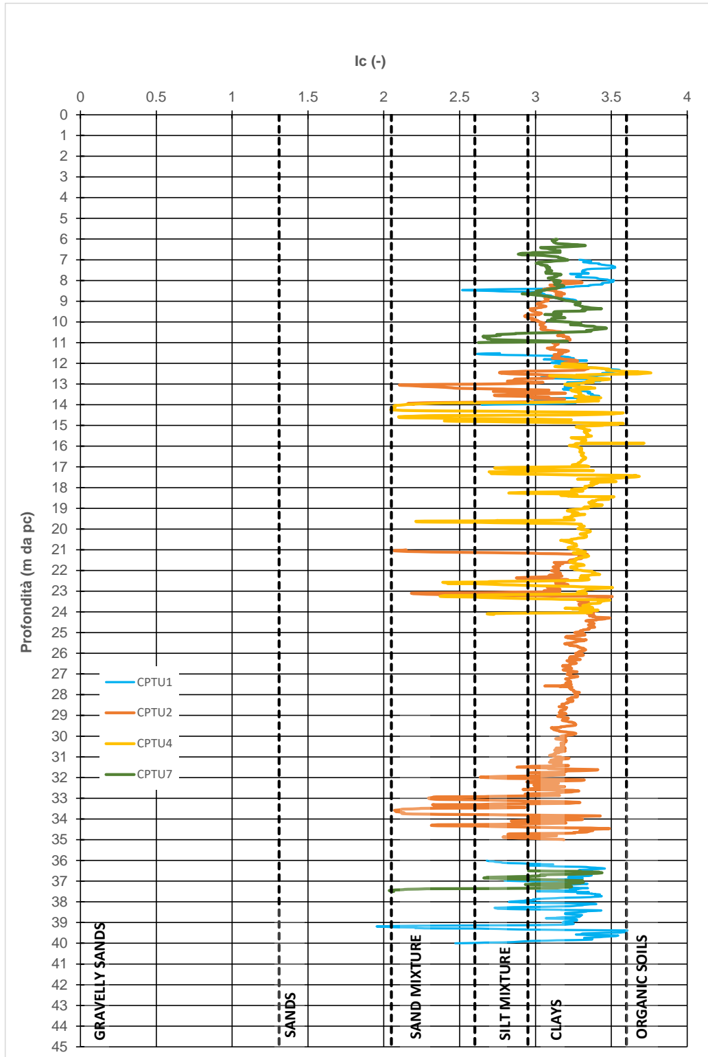
Figura 9-35: AL1 – Indice di comportamento I_c
