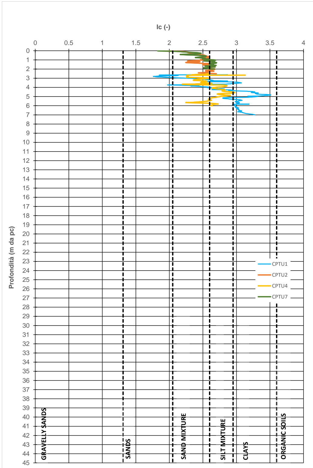
Figura 9-3: R – Indice di comportamento I_c
