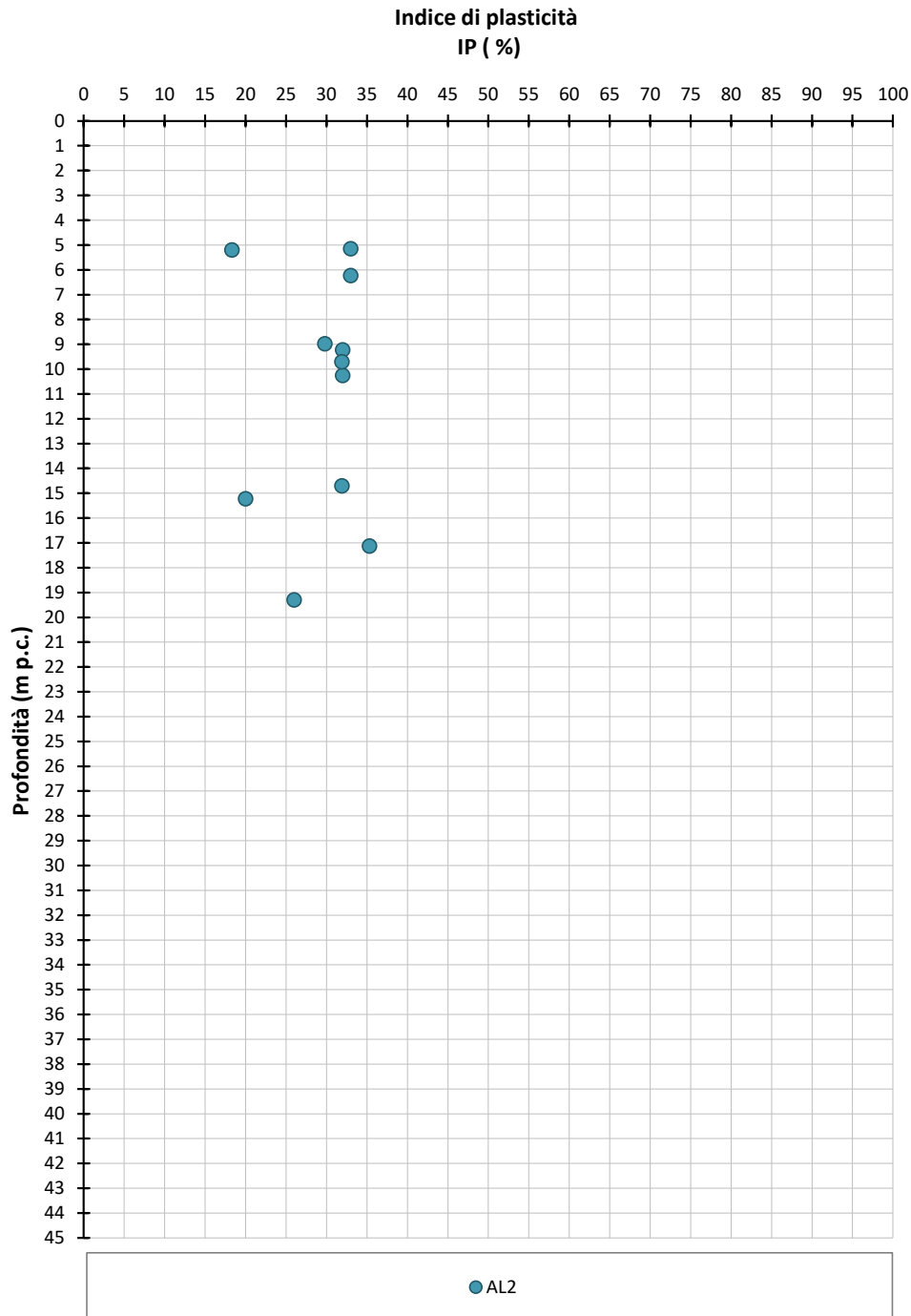
Figura 9-59: AL2 - Indice di plasticità PI
