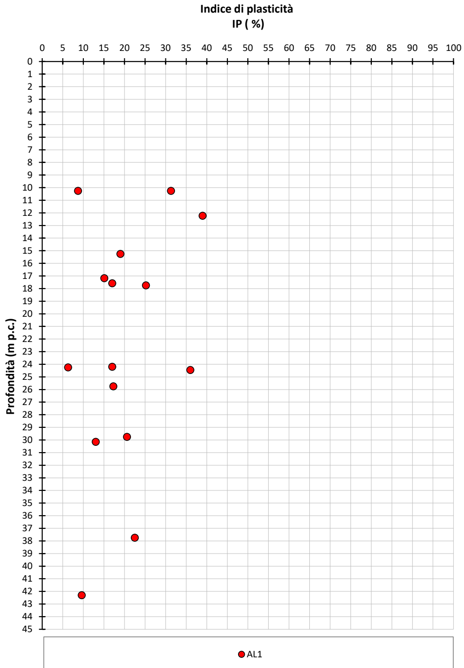
Figura 9-42: AL1 - Indice di plasticità PI
