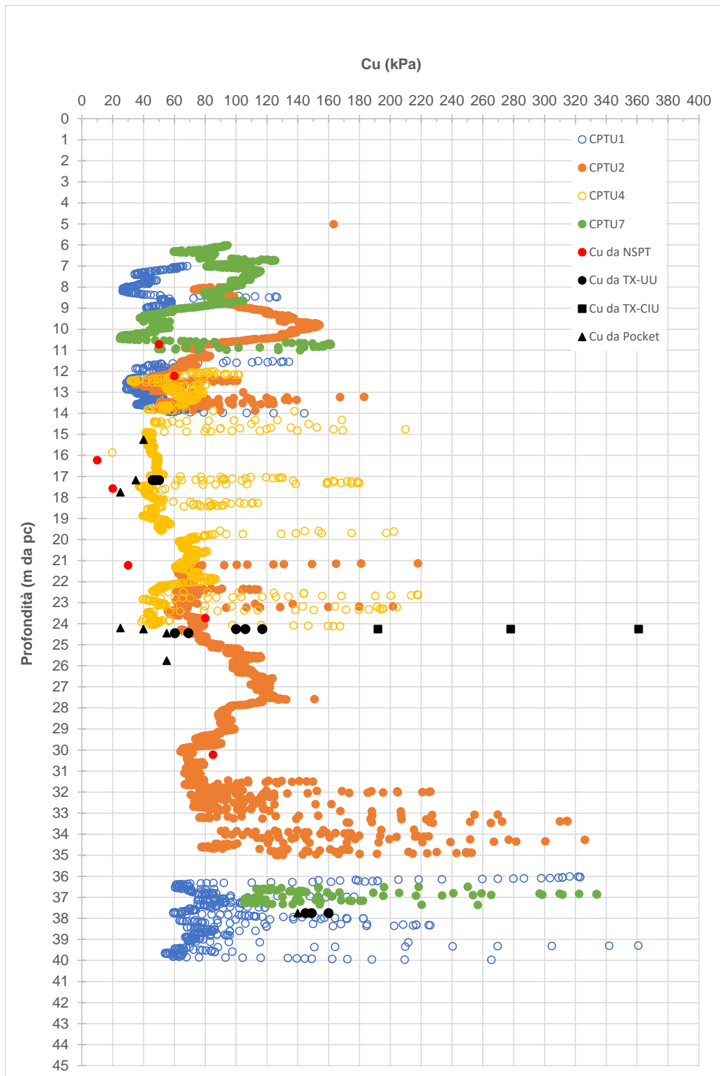
Figura 9-44: AL1 – Cu da prove in sito e laboratorio
