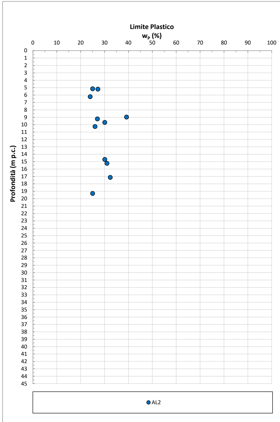
Figura 9-58: AL2 – Limite Plastico
