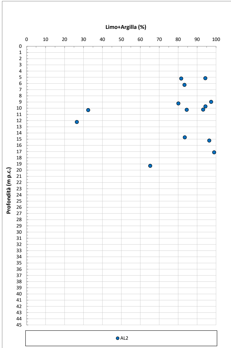
Figura 9-54: AL2 – Contenuto di fini Limo+Argilla
