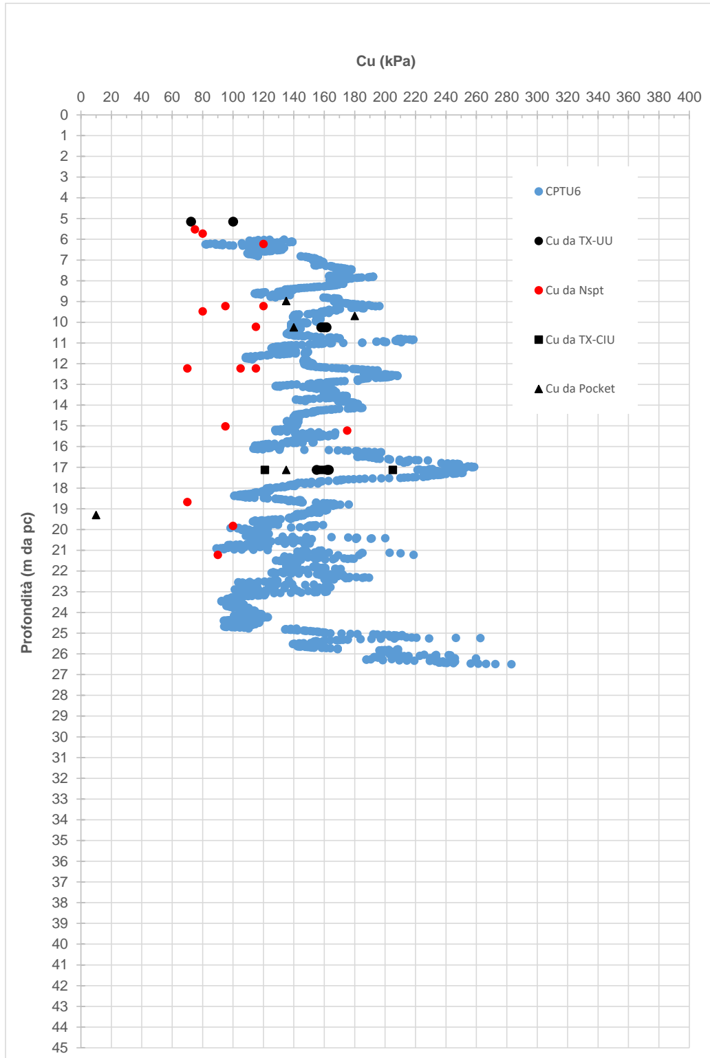
Figura 9-61: AL2 – Cu da prove in sito e laboratorio
