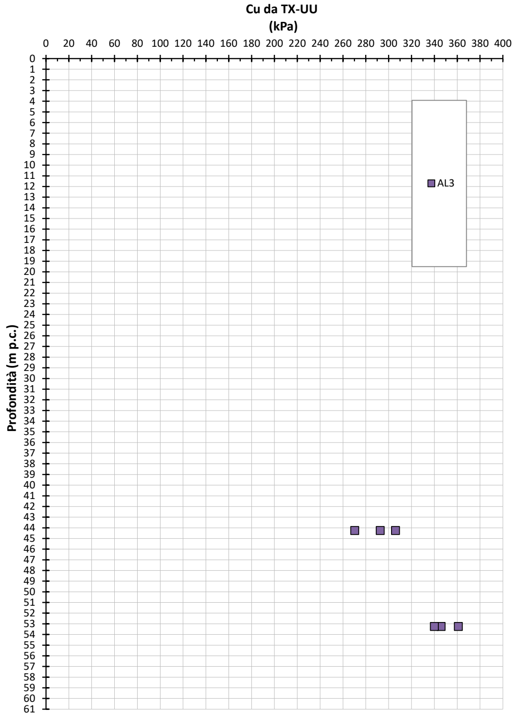
Figura 9-85: AL3 – Cu da prove di laboratorio TX-UU
