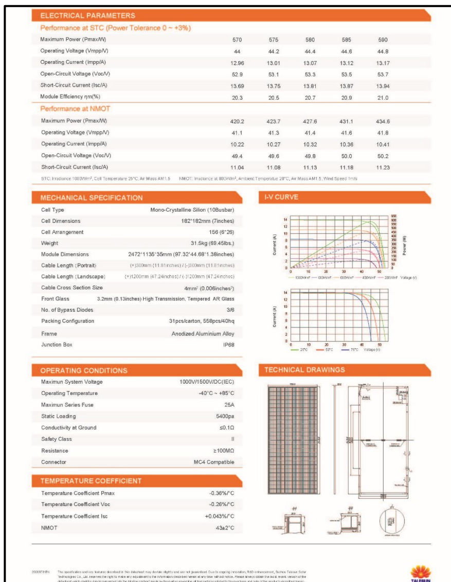
Figura 6: Scheda elettrica modulo fotovoltaico
