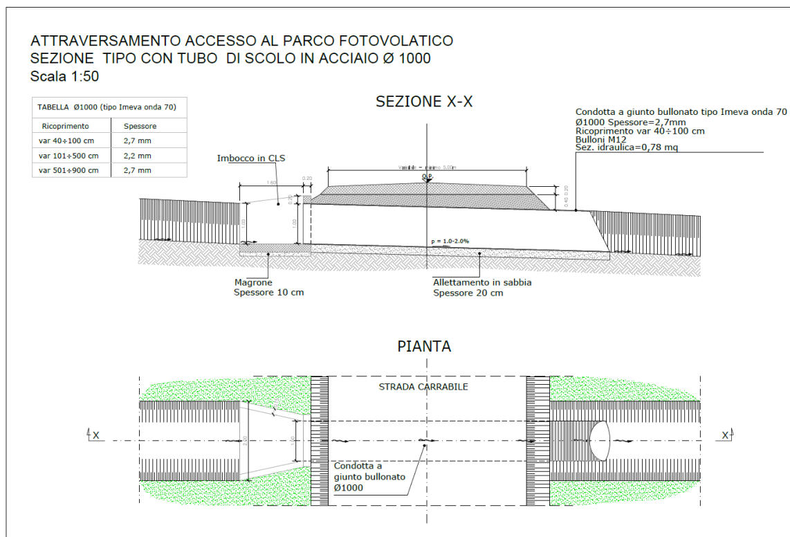
Figura 14: sezione tipo attraversamento canale
