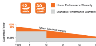
Figura 5 - Scheda tecnica commerciale di un modulo fotovoltaico compatibile con il progetto
