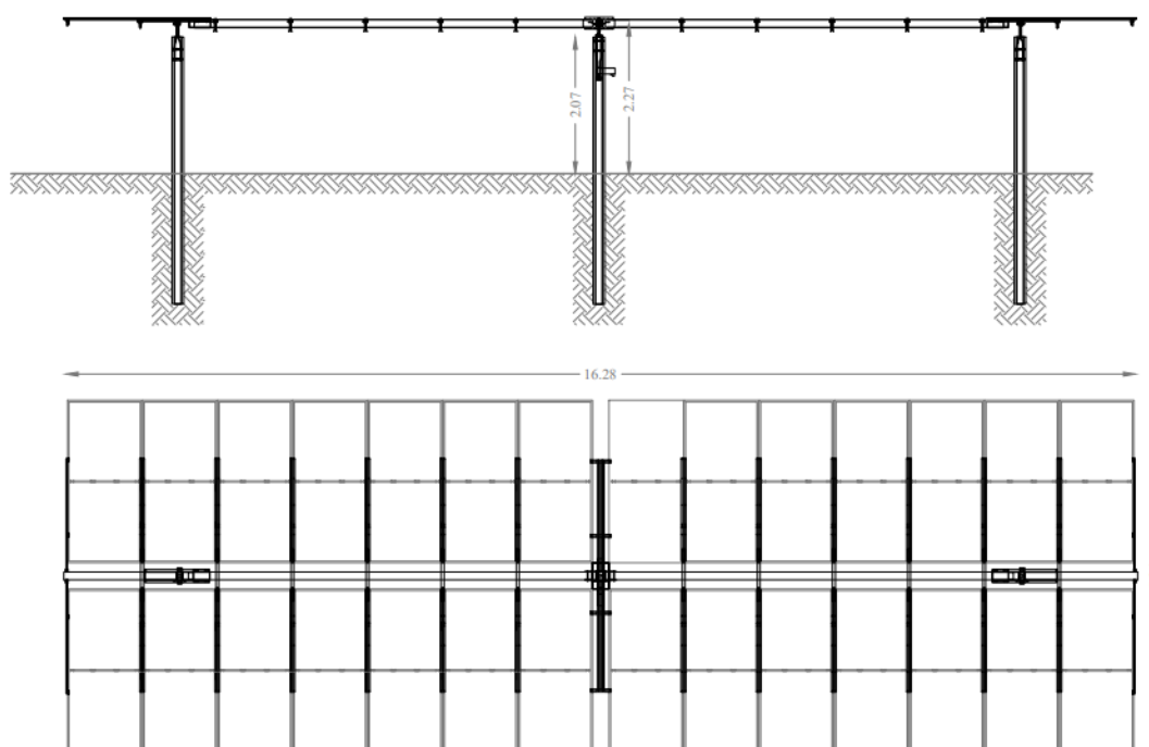
Figura 7: Struttura di Supporto – inseguitori mono assiali per i moduli fotovoltaici
