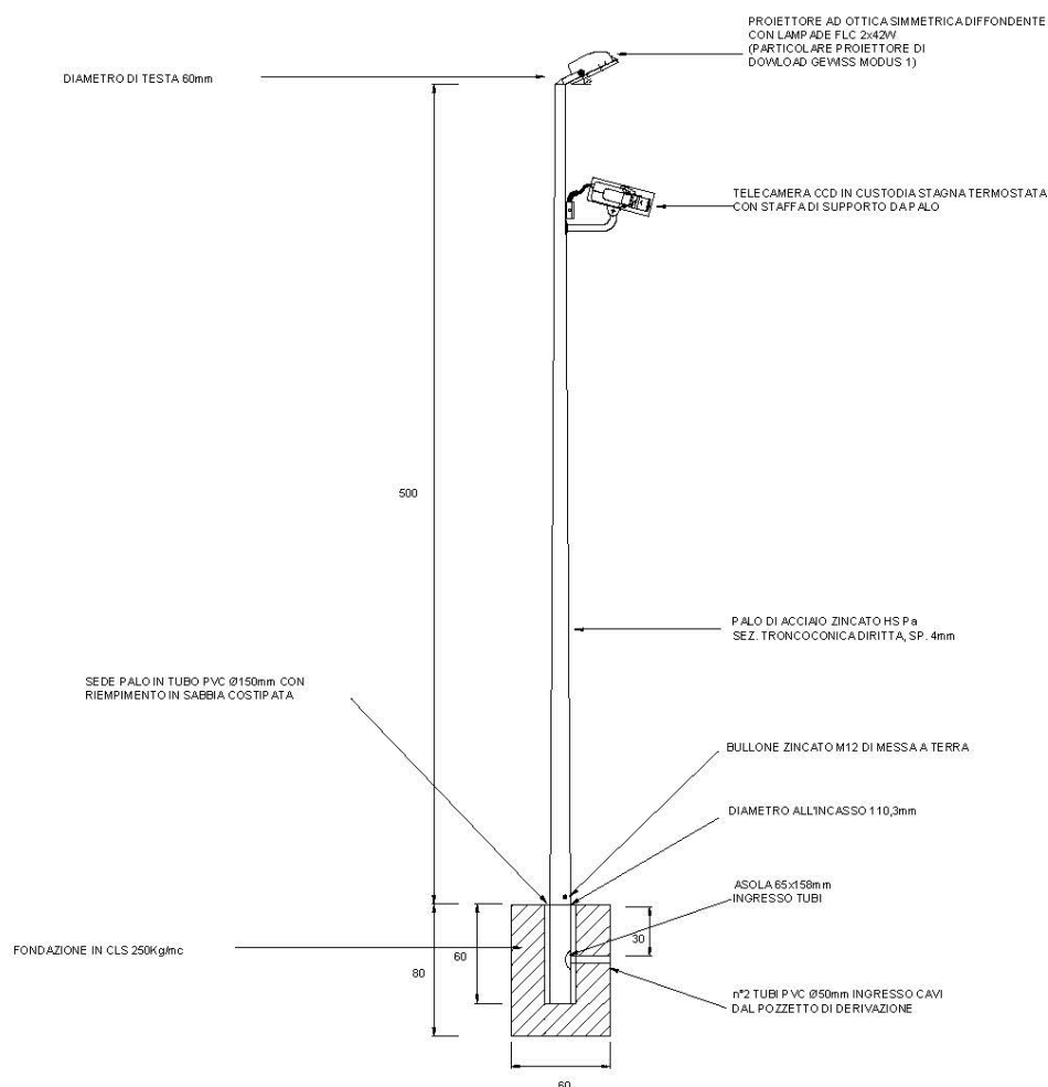
Figura 16: Impianto illuminazione e sorveglianza tipo
