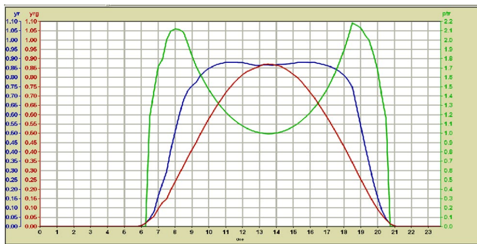
Figura 4 - Confronto tra un impianto fisso (linea rossa) ed un impianto con inseguitori (linea blu), l'area compresa tra le due linee indica la maggior produzione.
