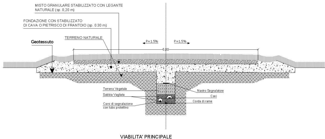
Figura 12: sezione stradale tipo
