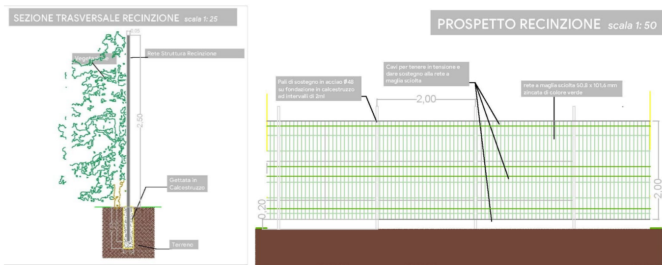
Figura 15: particolare recinzione
