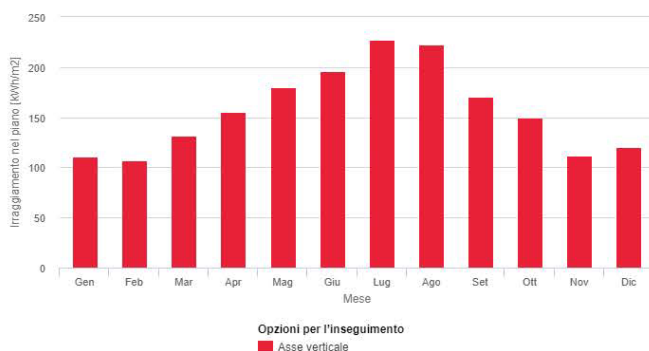
Figura 18: irraggiamento /energia media mensile
