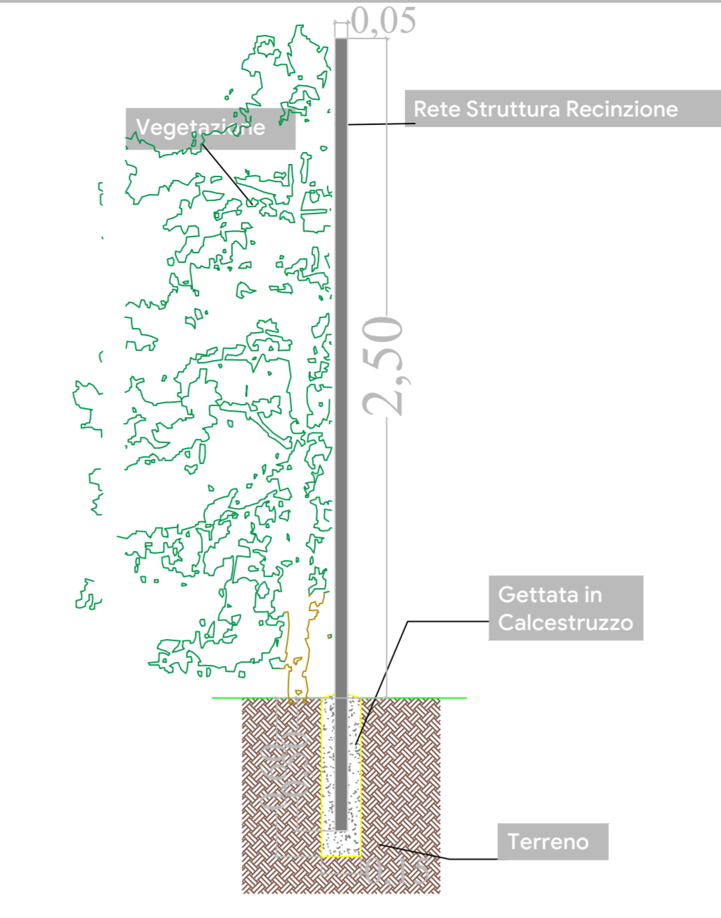
PROSPETTO RECINZIONE scala 1: 50
