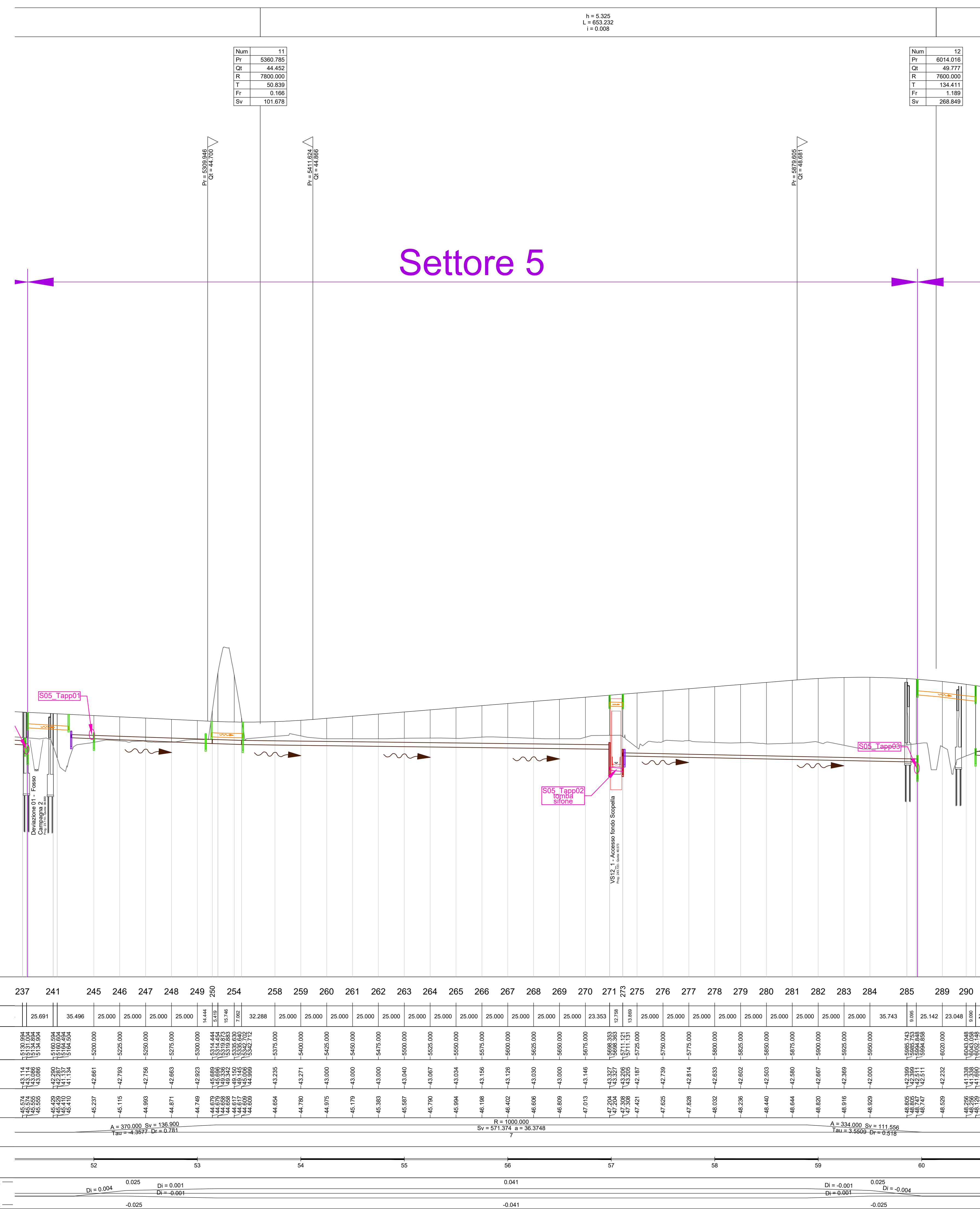
Profilo longitudinale reti impianti di trattamento tubazione lato DX - quinto settore
