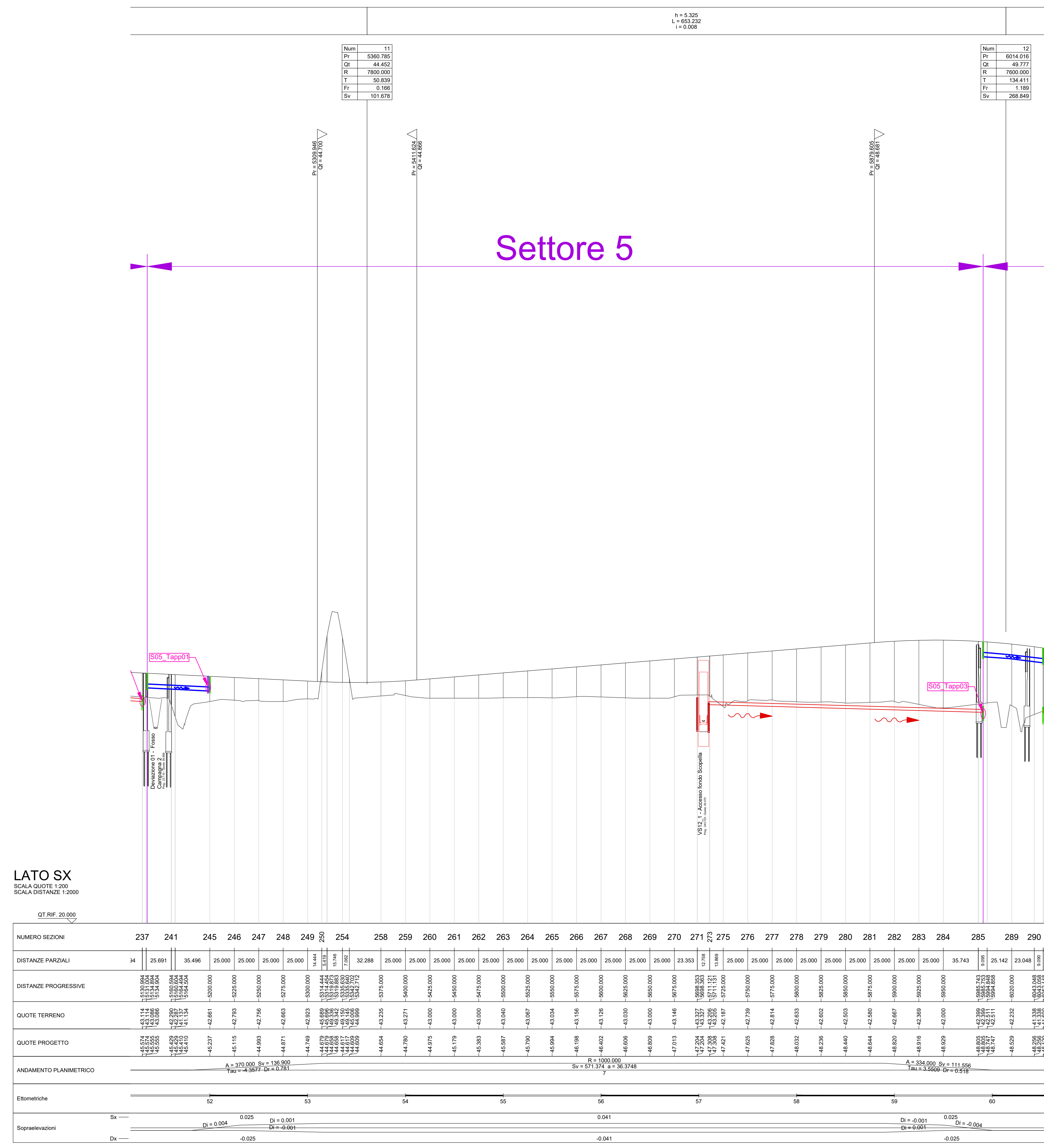
Profilo longitudinale reti impianti di trattamento tubazione lato SX - quinto settore
