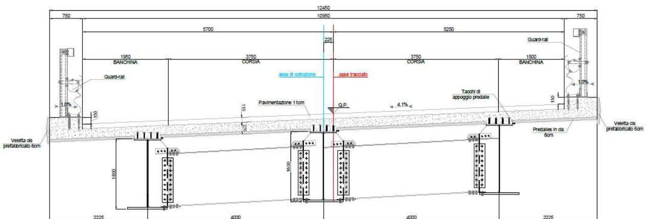
Figura 1.4 sezione trasversale dell'impalcato
