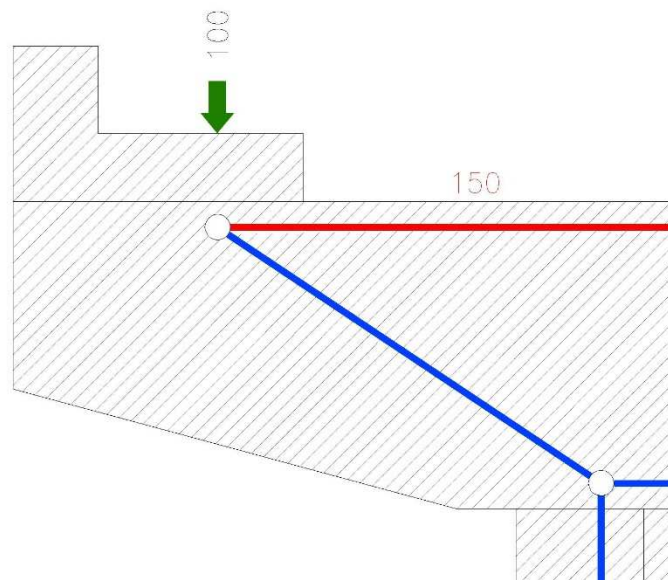
Figura 8.2. Schema di calcolo
