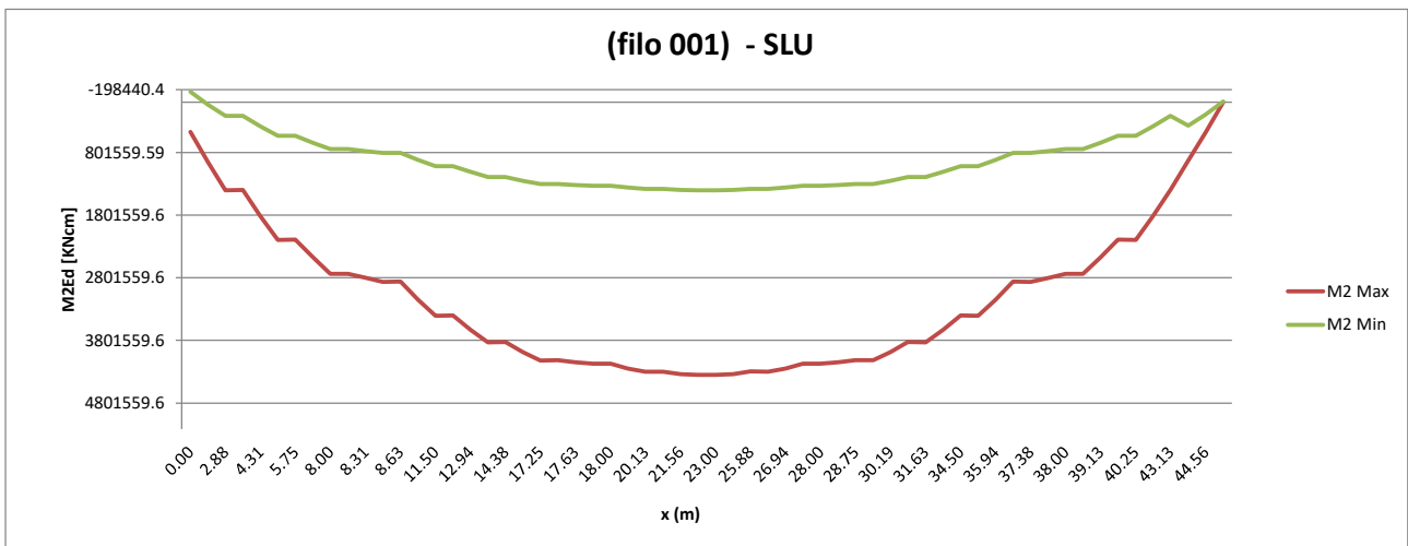
Figura 6.15: Involuppo del momento sulla trave esterna (filo 001).
