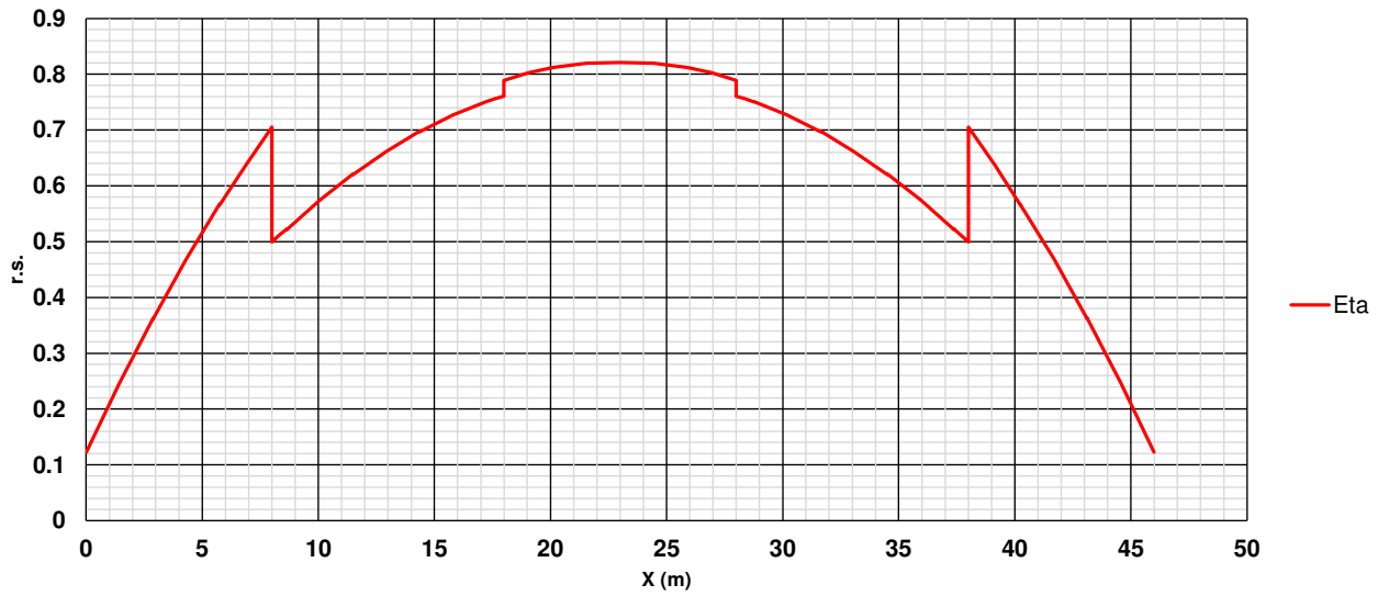
SLU: rapporto di sfruttamento assoluto eta
