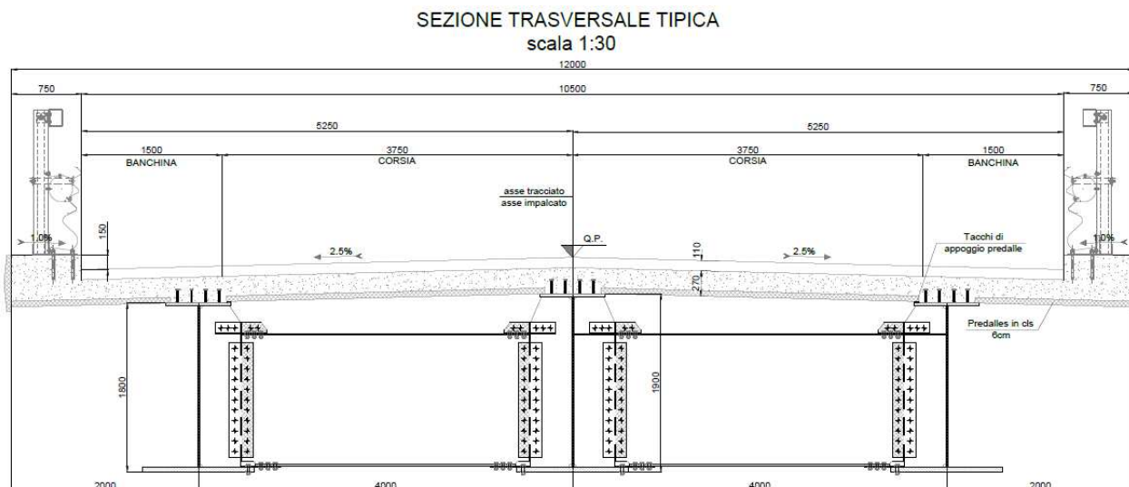
Figura 1.1. Sezione trasversale tipologica
