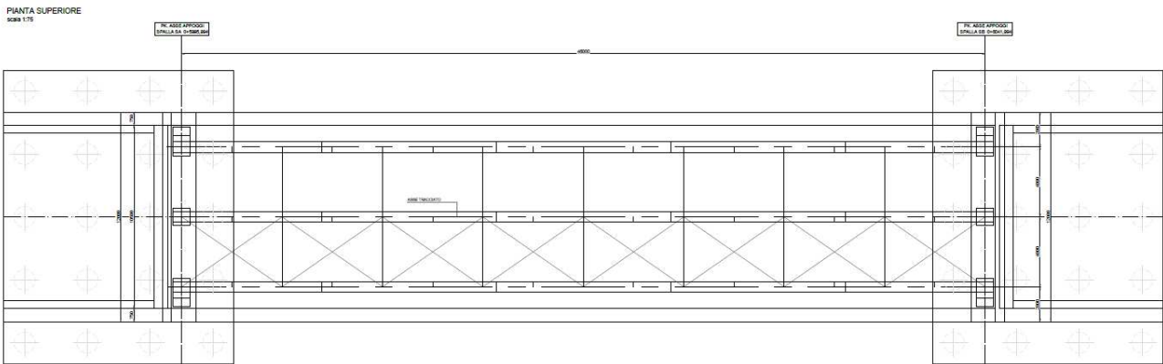
Figura 1.2. Pianta superiore impalcato
