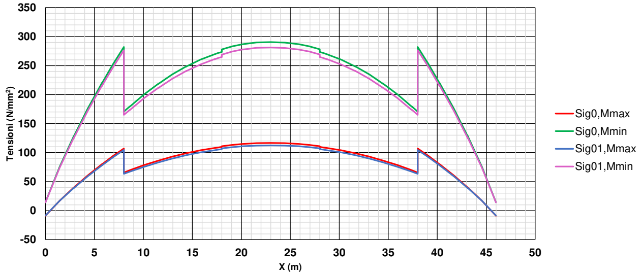
SLU: tensioni elastiche all'intradosso della trave
