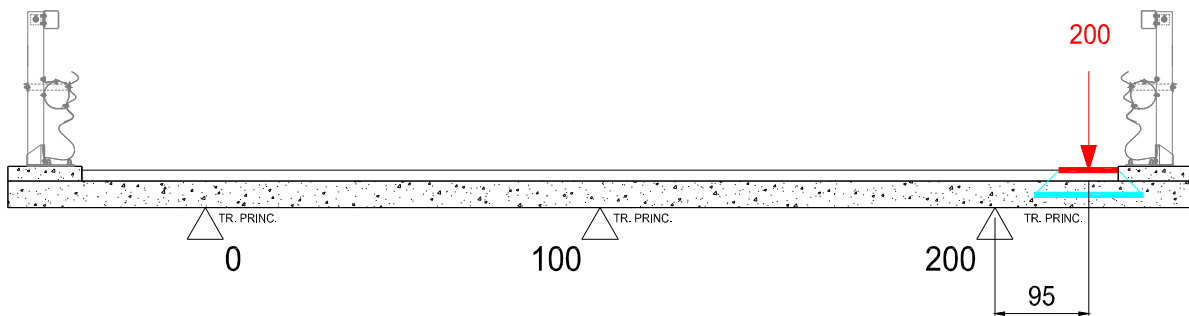
Figura 9.10. Minimo momento negativo su trave esterna - Schema di carico 2
