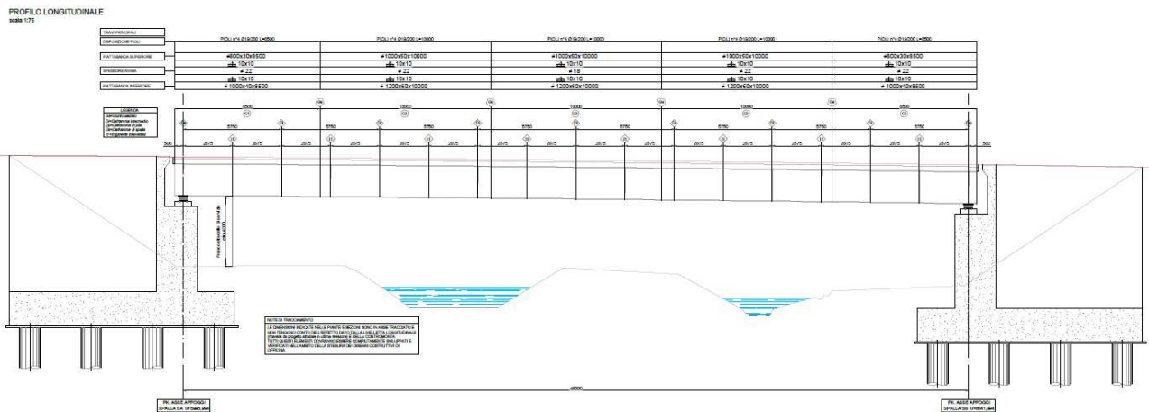
Figura 1.3. Profilo longitudinale
