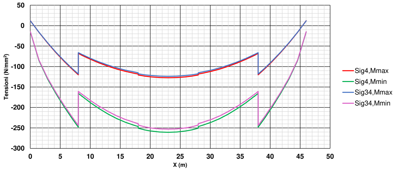
SLU: tensioni elastiche all'estradosso della trave
