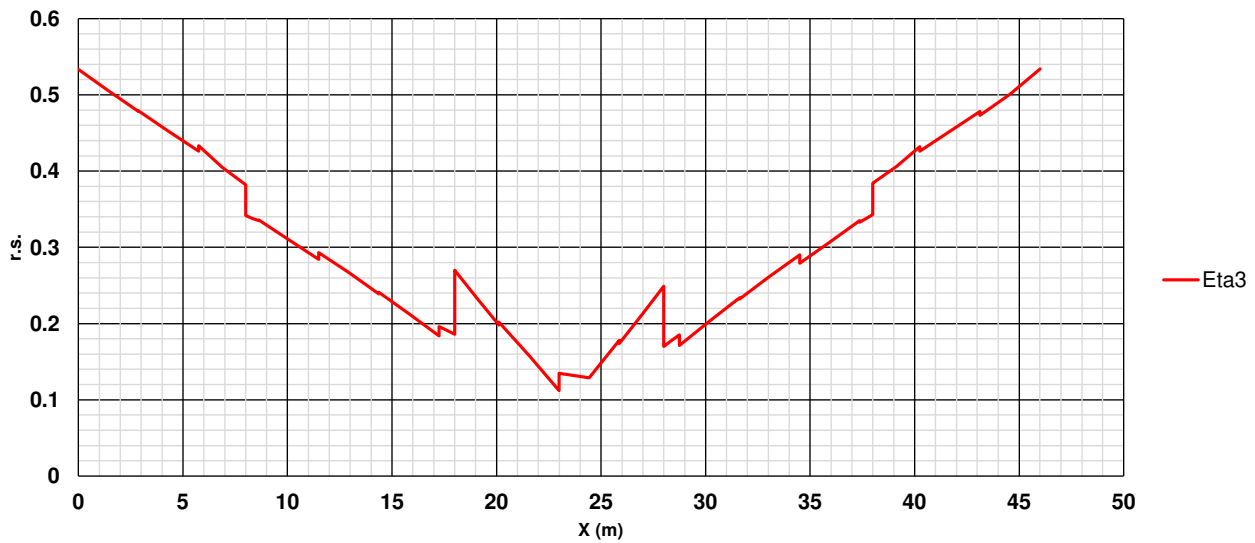
SLU: rapporto di sfruttamento a taglio eta3
