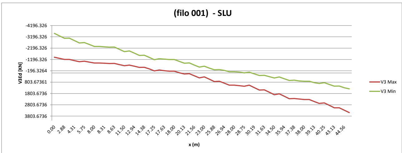
Figura 6.16: Involuppo del taglio sulla trave esterna (filo 001).
