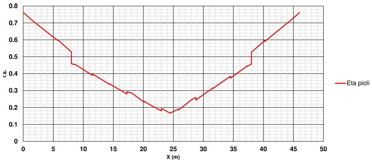
SLE: rapporto di sfruttamento dei connettori
