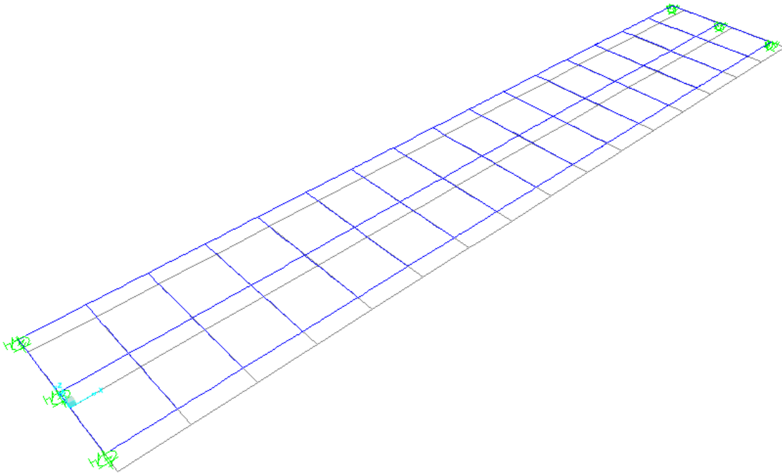
Figura 6-3: Primo modo di vibrare ( T = 1.399 )
