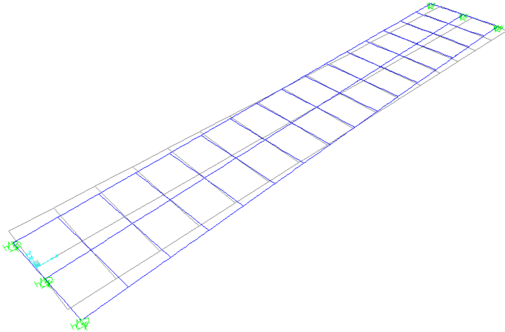
Figura 6-5: Terzo modo di vibrare ( T = 0.828 )
