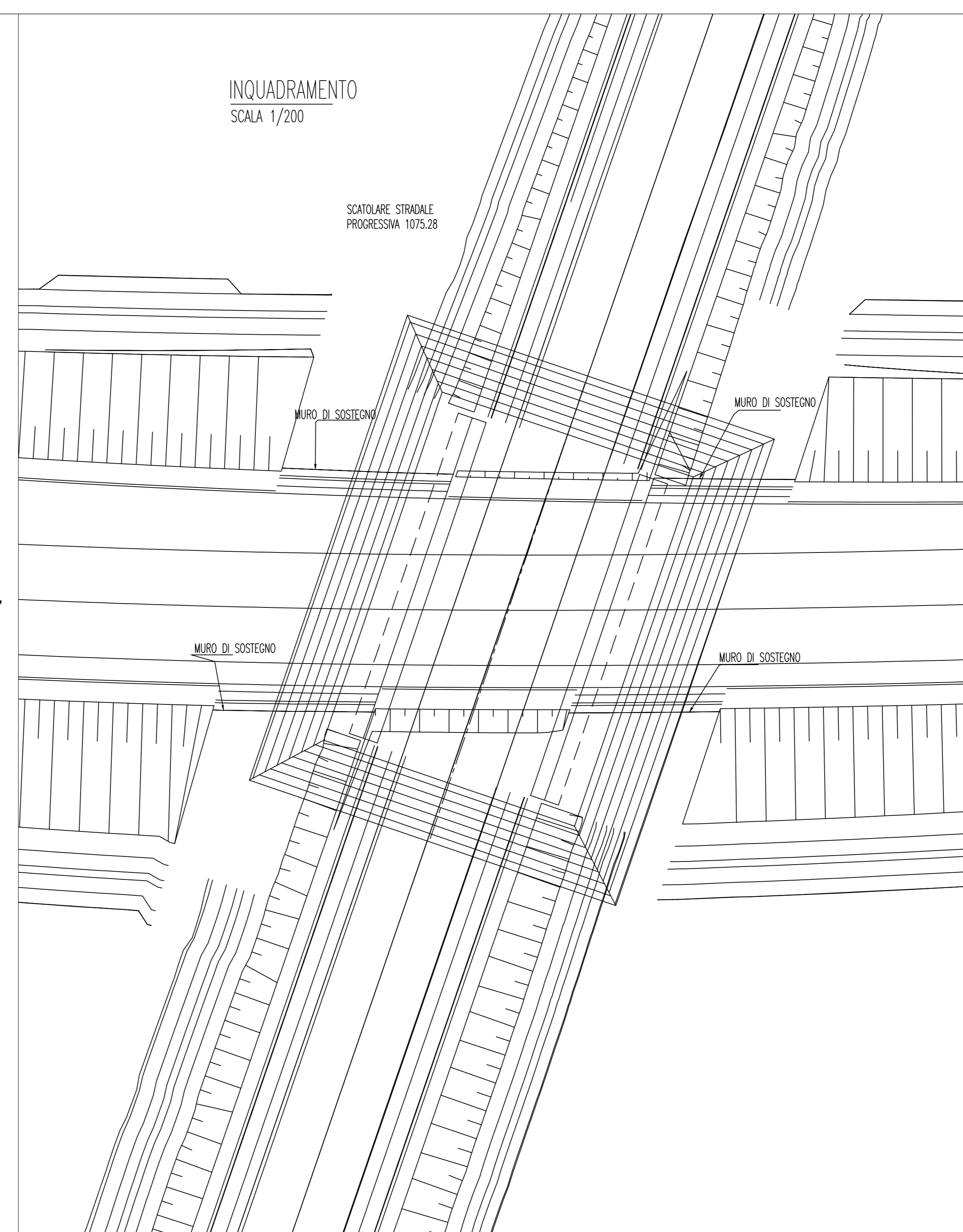
SOTTOVA SCATOLARI E MURI DI SOSTEGNO - CLS E ACCIAIO
