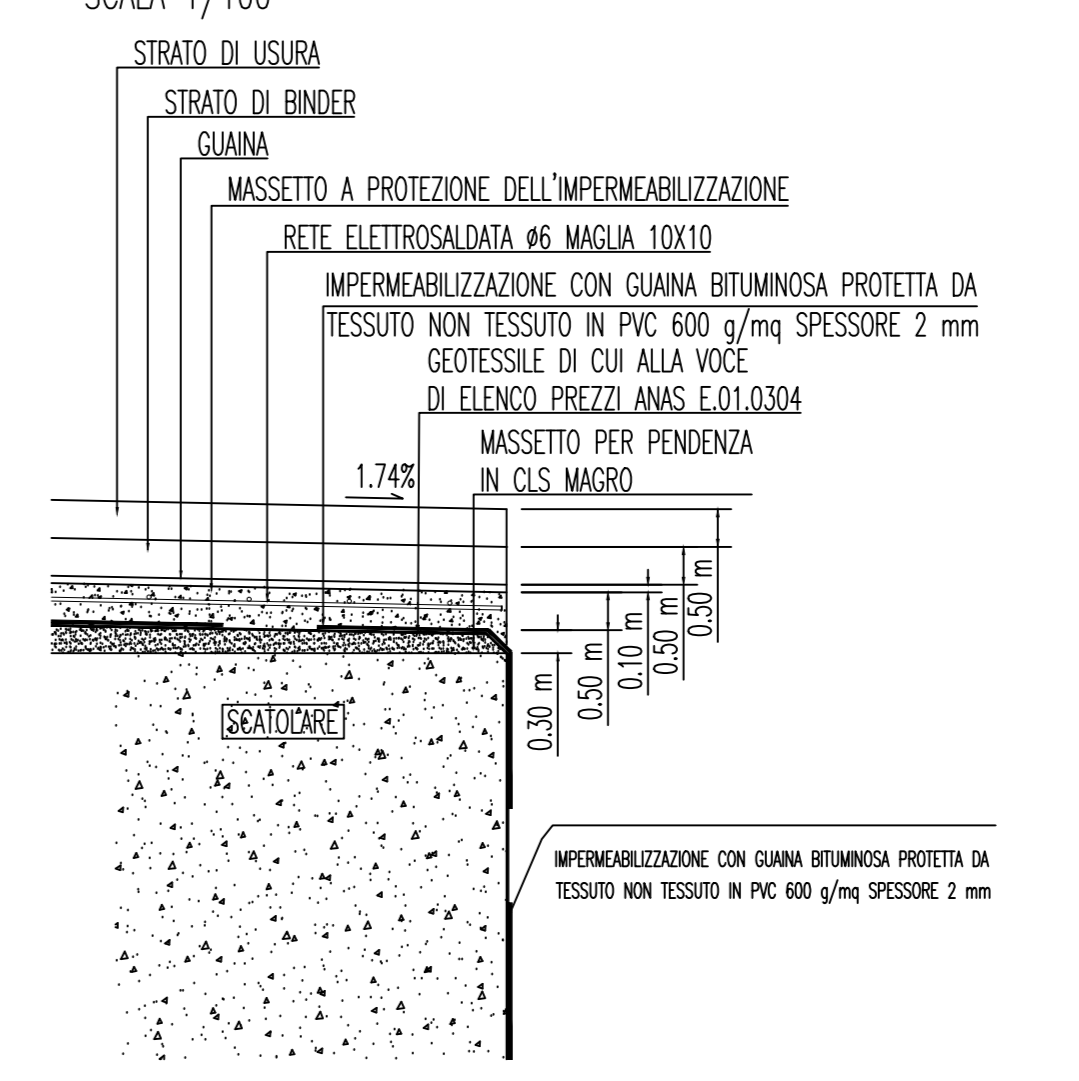
DETTAGLIO 1 SCALA 1/100
