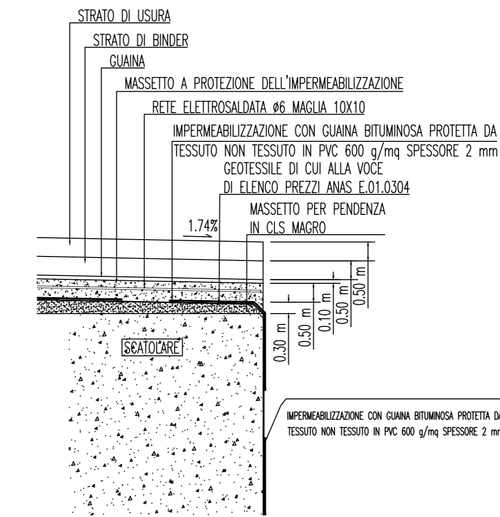
DETTAGLIO 1 SCALA 1/100
