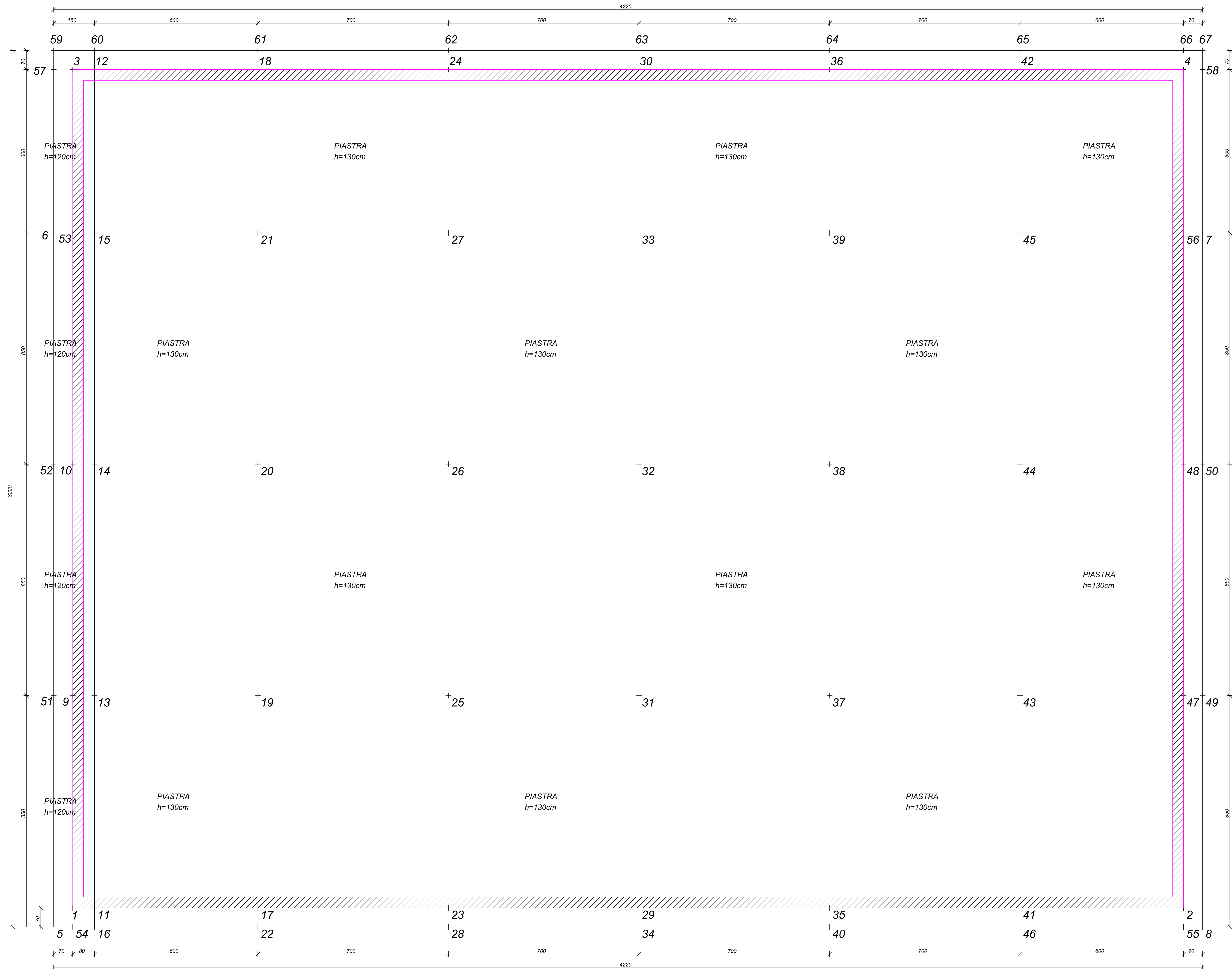
PIANTA IMPALCATO QUOTA m: 0.00
