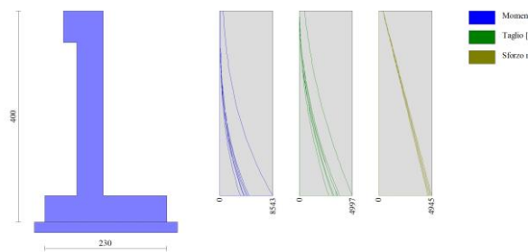
Fig. 5 - Paramento (Inviluppo)
