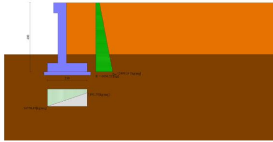
Fig. 2 - Diagramma delle pressioni (combinazione statica) (Combinazione n° 10)
