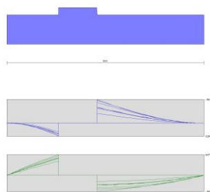
Fig. 7 - Fondazione (Inviluppo)
