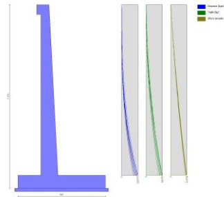
Fig. 5 - Paramento (Inviluppo)
