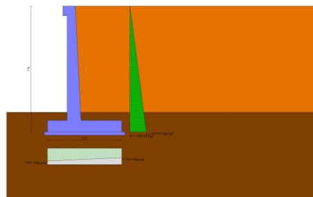
Fig. 2 - Diagramma delle pressioni (combinazione statica) (Combinazione n° 1)
