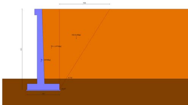
Fig. 5 - Cuneo di spinta (combinazione statica) (Combinazione n° 1)
