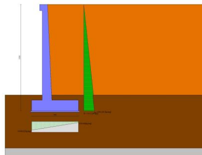
Fig. 2 - Diagramma delle pressioni (combinazione statica) (Combinazione n° 1)
